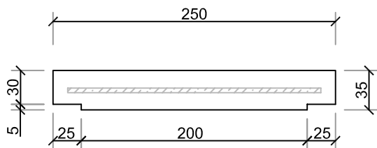
TAPA 500X250X35
