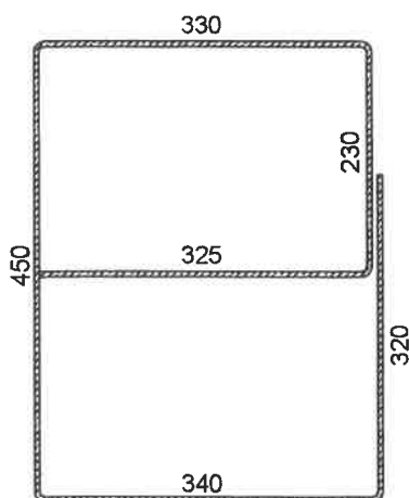
DETALLE DE ESTRIBO Ø5
