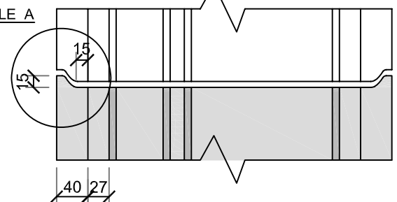
PLANTA BORDE CANALETA
