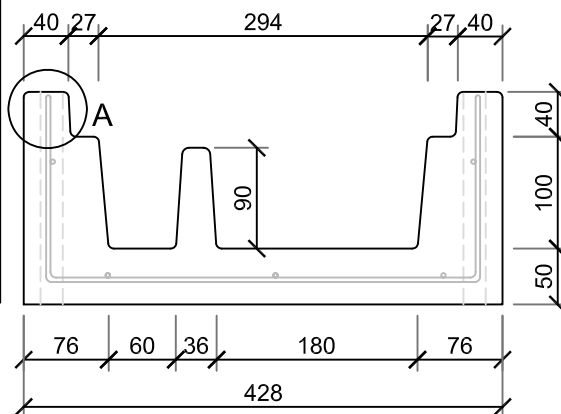
DETALLE DE ESTRIBO Ø5 mm.
