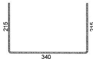
CORTE DE MALLA 950X770
