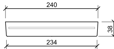
ALZADO LATERAL TAPA
