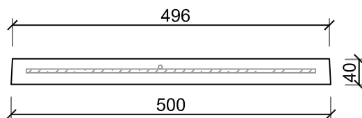
ALZADO LATERAL TAPA
