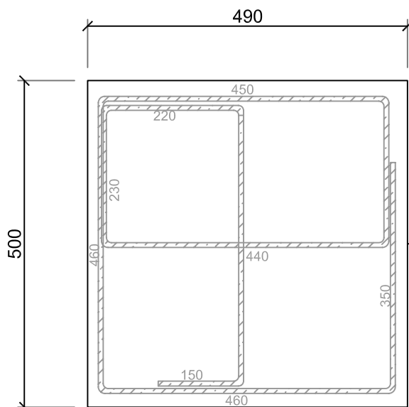
DETALLE DE ESTRIBO Ø6 mm.
