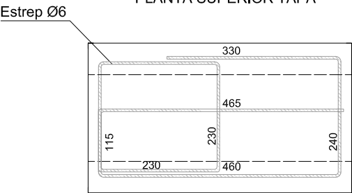
PLANTA SUPERIOR TAPA
