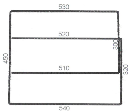
DETALLE DE ESTRIBO Ø6
