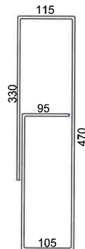
Detalle de armadura en TAPA
