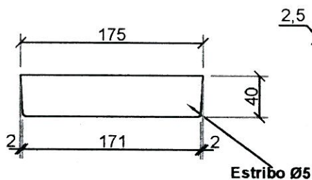
ALZADO FRONTAL TAPA
