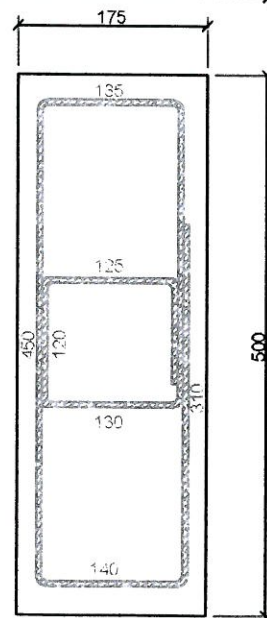
DETALLE DE ESTRIBO Ø 5 MM.
