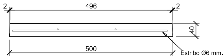
ALZADO FRONTAL TAPA
