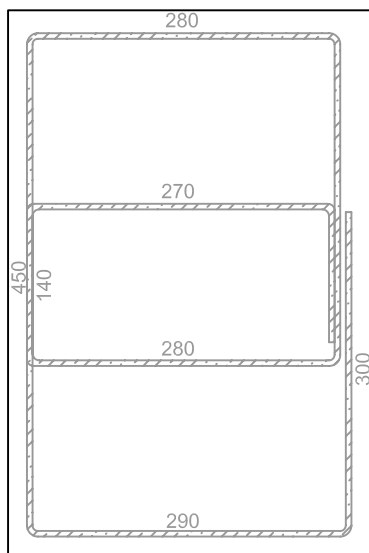
DETALLE DE ESTRIBO Ø5 mm.
