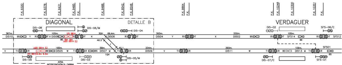
Imatge 3. Esquema CCVV i senyals tram Diagonal - Verdaguier L5 de F.M.B.
