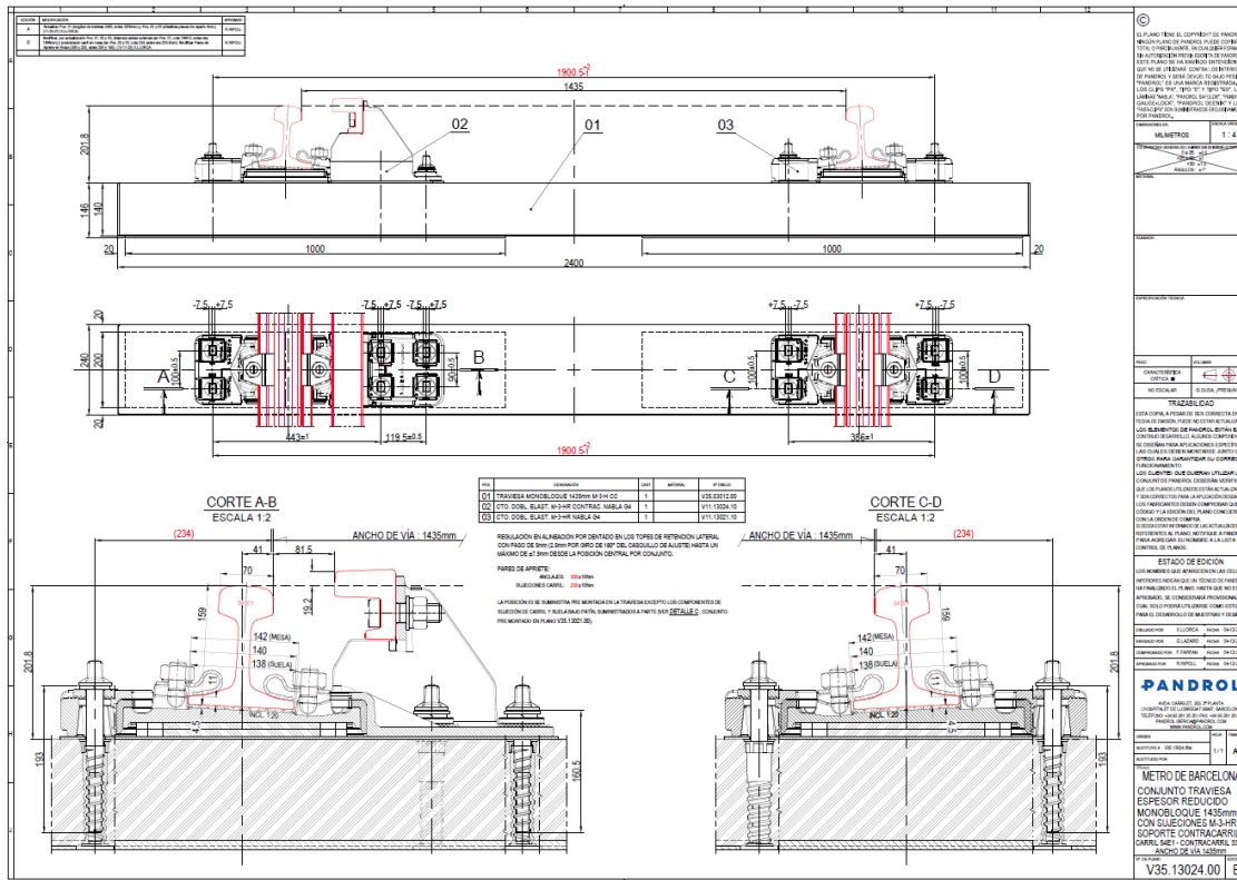
Plànol 4. Exemple tipus de travessa monobloc amb cantell reduït amb fixació antivibratòria d'FMB per a corba
