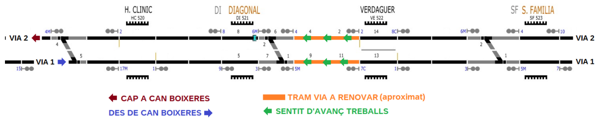
Il·lustració 13. Croquis àmbit dels treballs (aproximat) i sentit de renovació de via.
