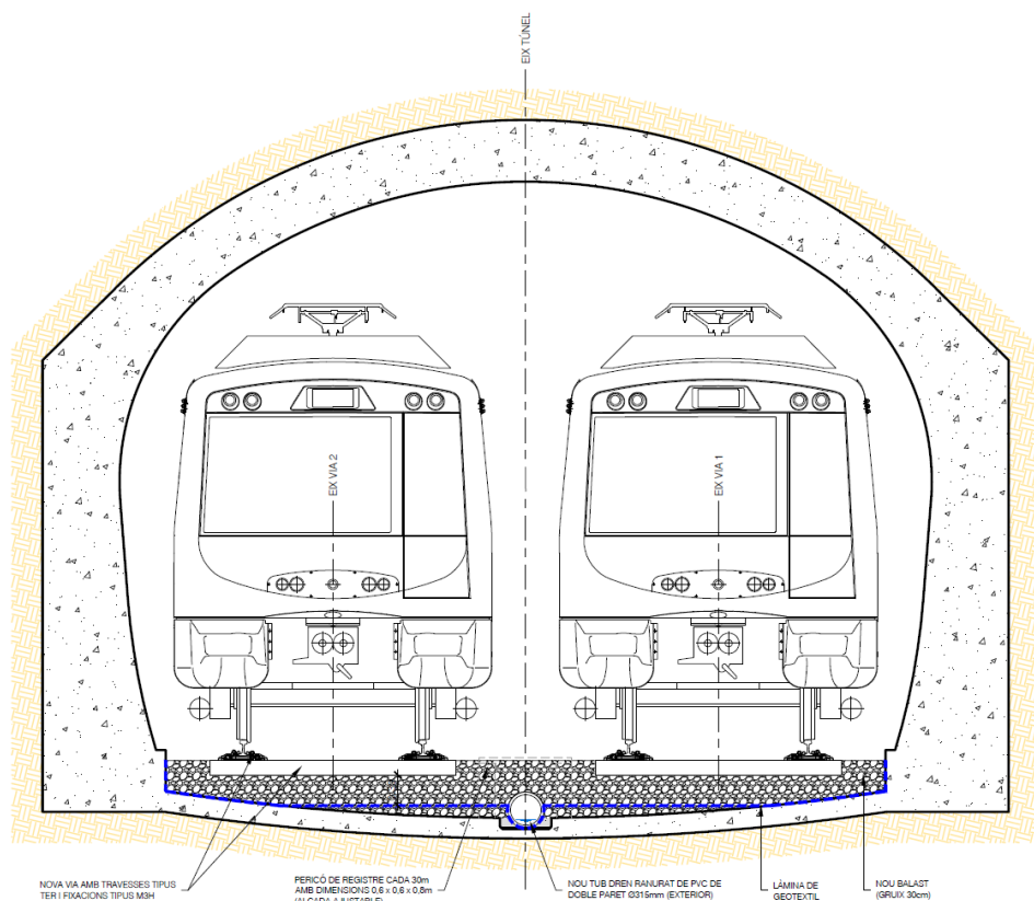
Il·lustració 11. Secció tipus via recta en Línia 5 de F.M.B.
