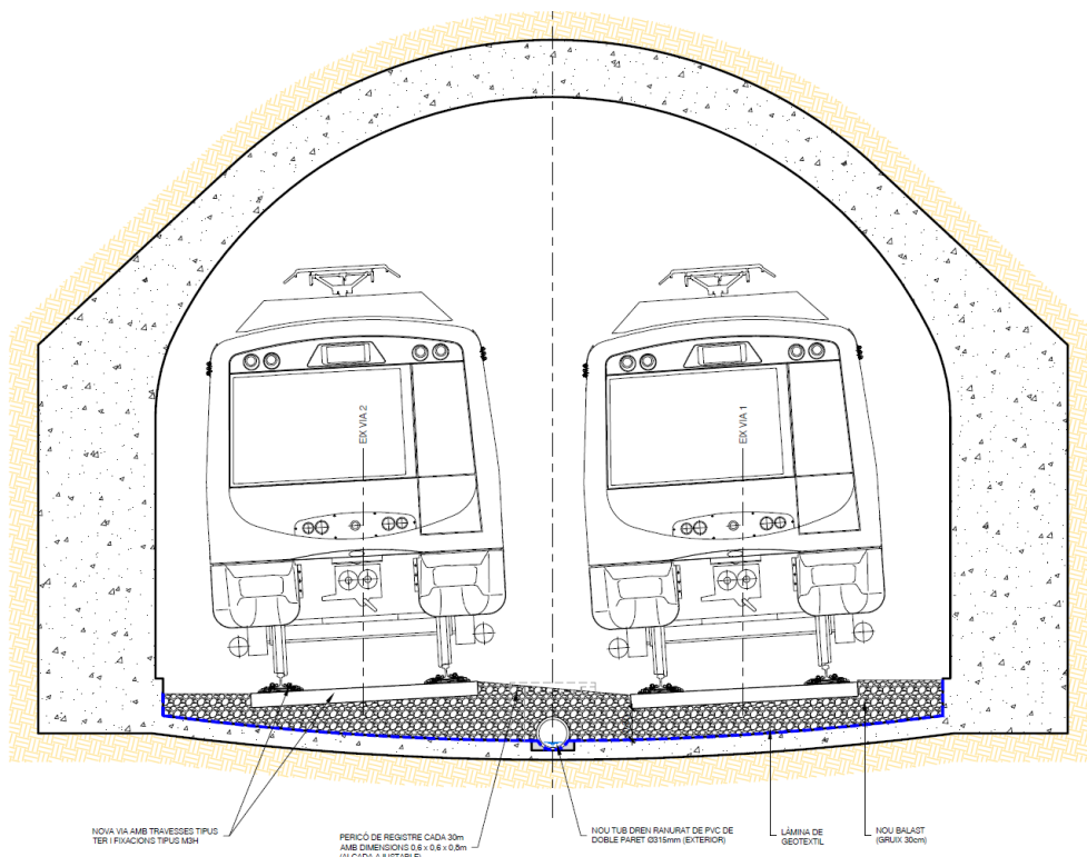
Plànol 6. Secció tipus via corba en Línia 5 de F.M.B.
