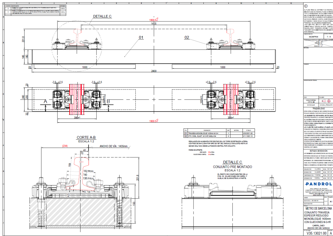
Il·lustració 10. Exemple tipus de travessa monobloc amb cantell reduït amb fixació antivibratòria d'FMB per a recta
