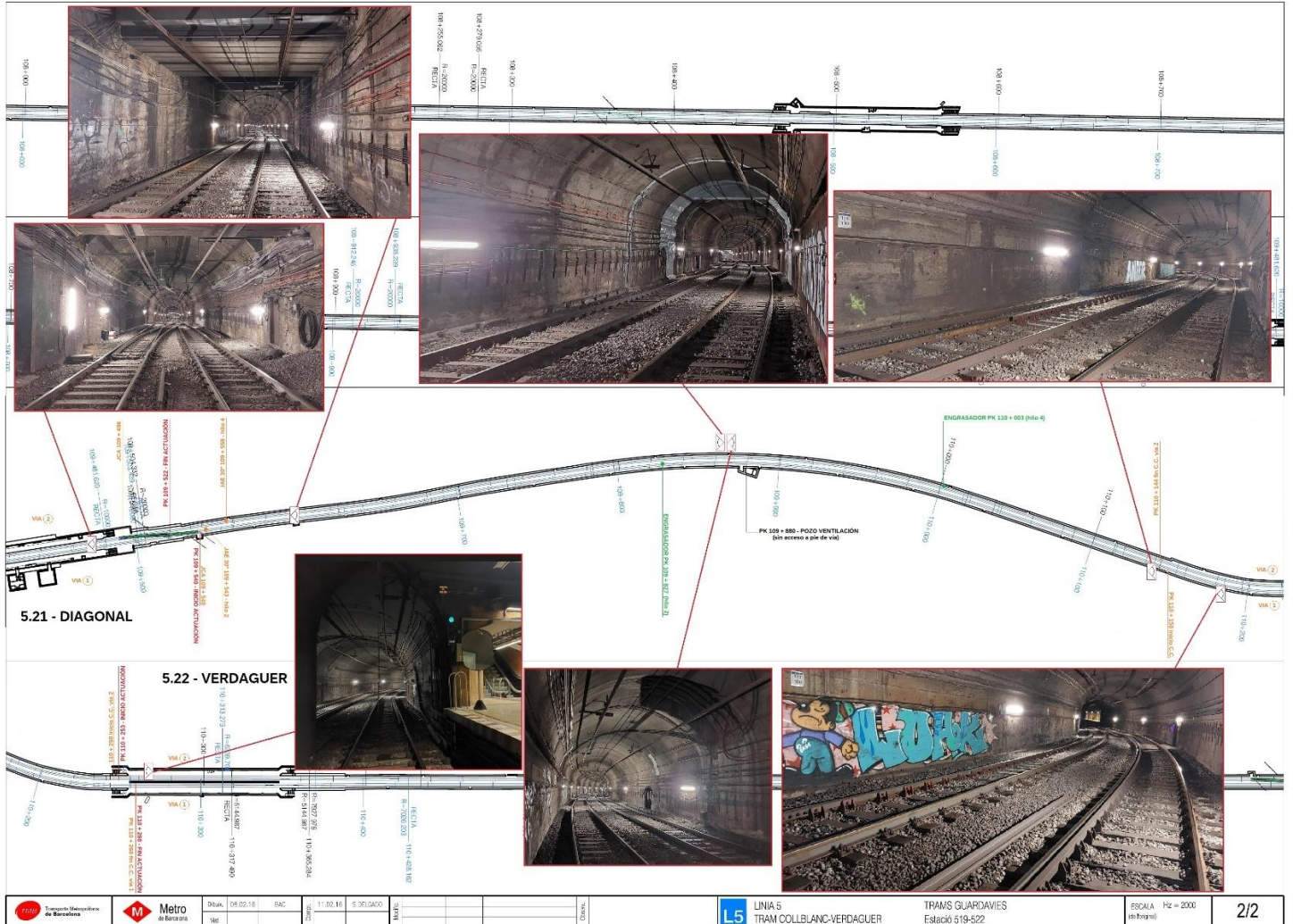
Il·lustració 9. Detall tram de via a renovar
