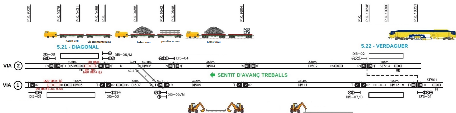
Il·lustració 5. Croquis proposta fase renovació i canvi de carril BLS via 2.
