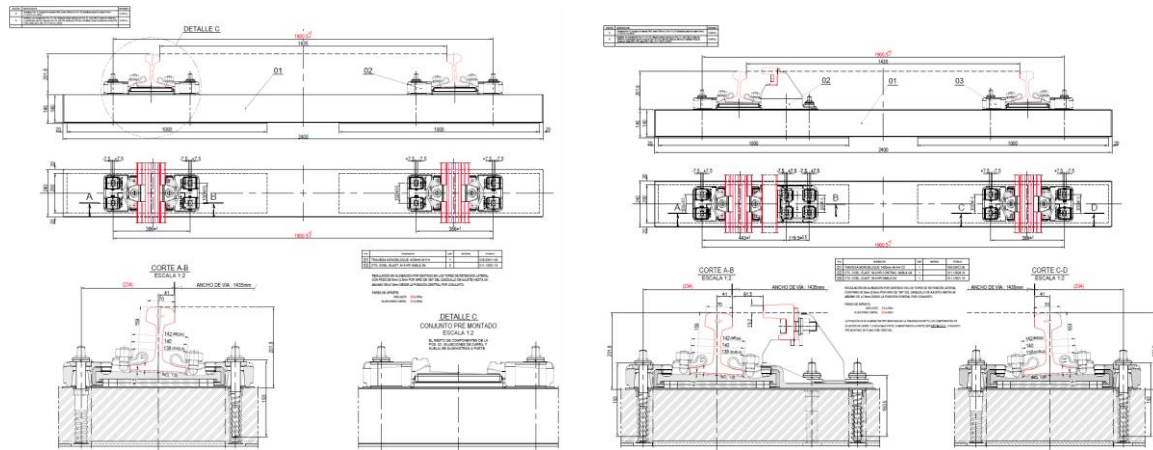
Imatge 1. Detall travesses monobloc cantell reduït F.M.B.
