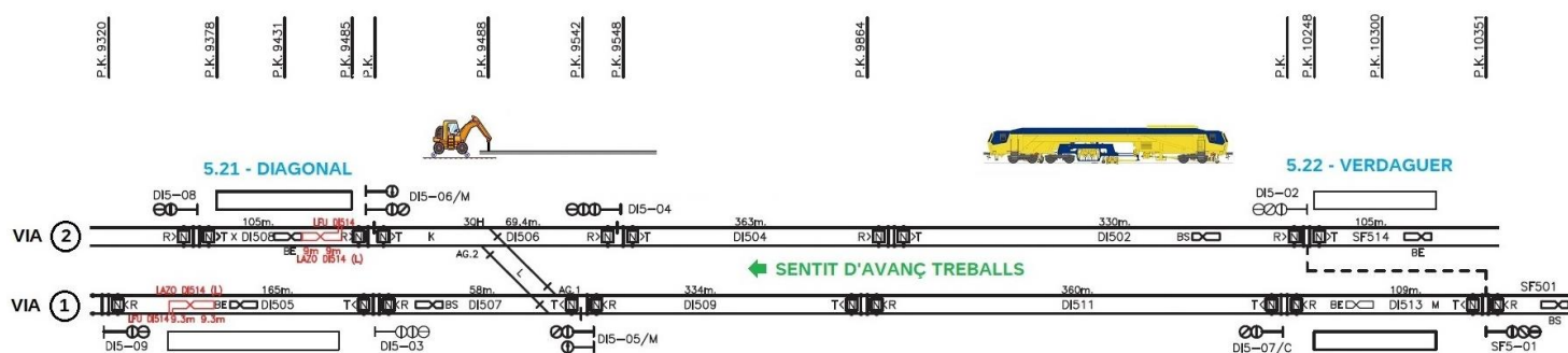
Il·lustració 6. Croquis proposta fase renovació BLS via 2 i segona nivellació.
