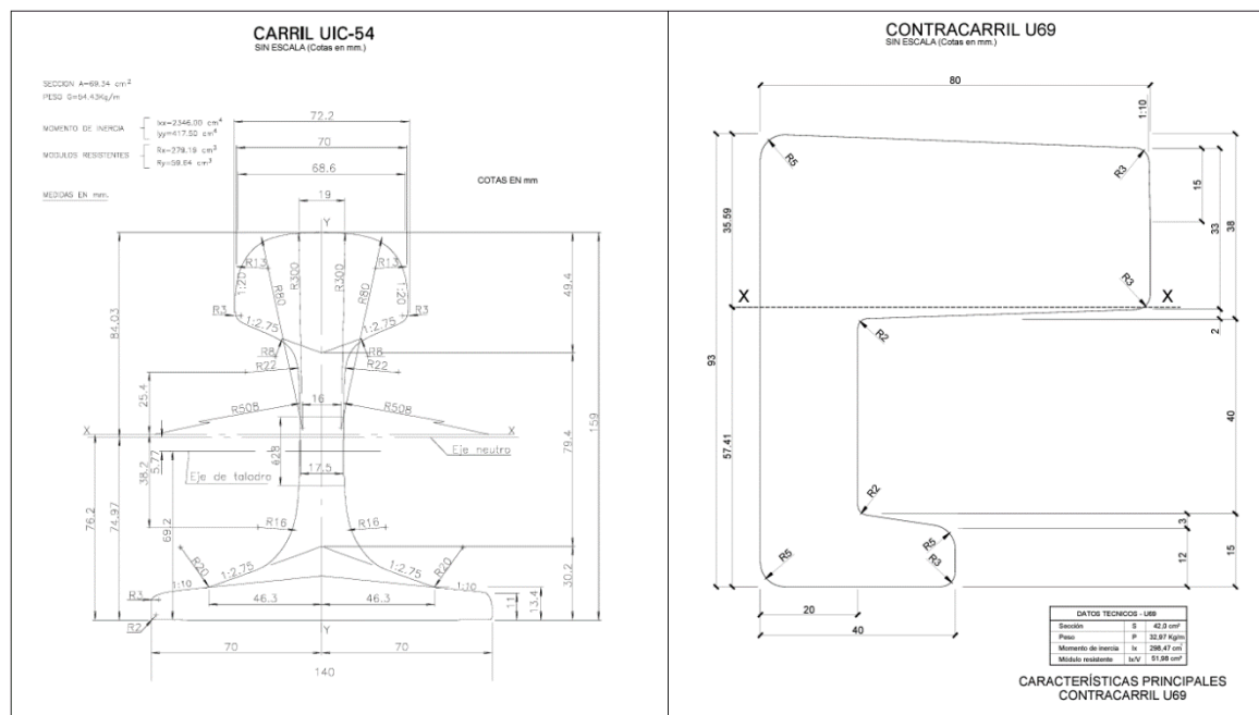
Imatge 2. Detall carril i contracarril a muntar.
