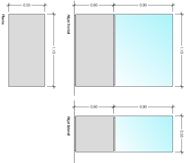
DETALL 3 / ESCALA 1:20
