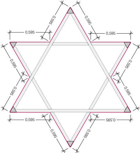
ESTRELLA PAS 4 / ESCALA 1:20
