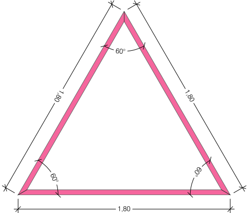
ESTRELLA PAS 1 / ESCALA 1:20
