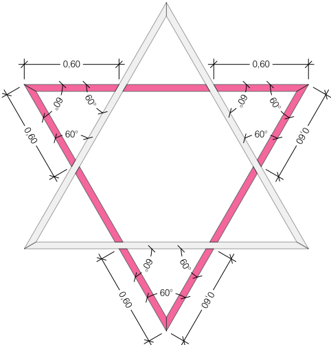
ESTRELLA PAS 2 / ESCALA 1:20
