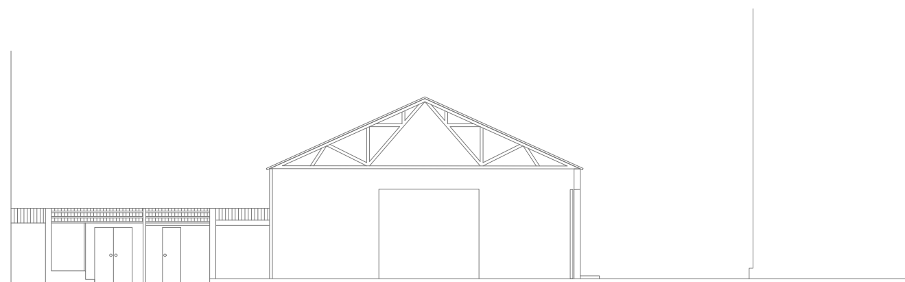
SECCIÓ C-C'
