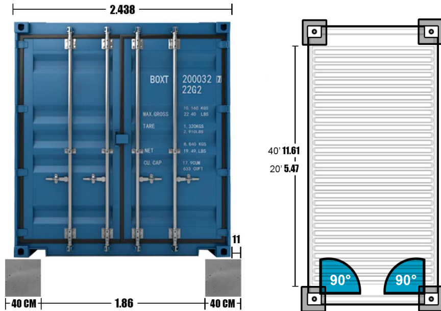
Proposta de suport en base a les mides aproximades del contenidor
