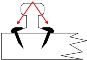
Mostra del tipus d'ancoratge amb claus de rails.
