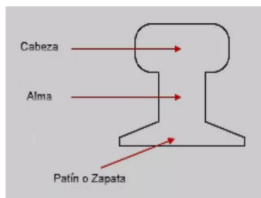
Perfil d'un rail de vagoneta
