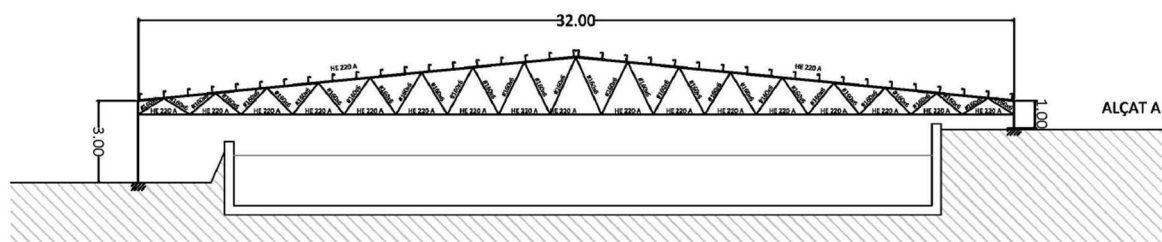
Imatge 5: dimensions del pòrtic
