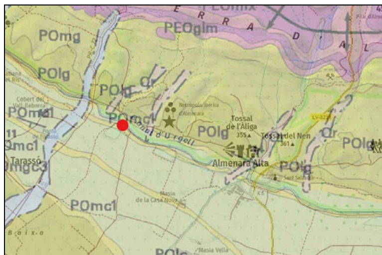
Figura 6. Mapa geològic de la zona d'estudi a escala 1:50.000. Font: ICGC.
