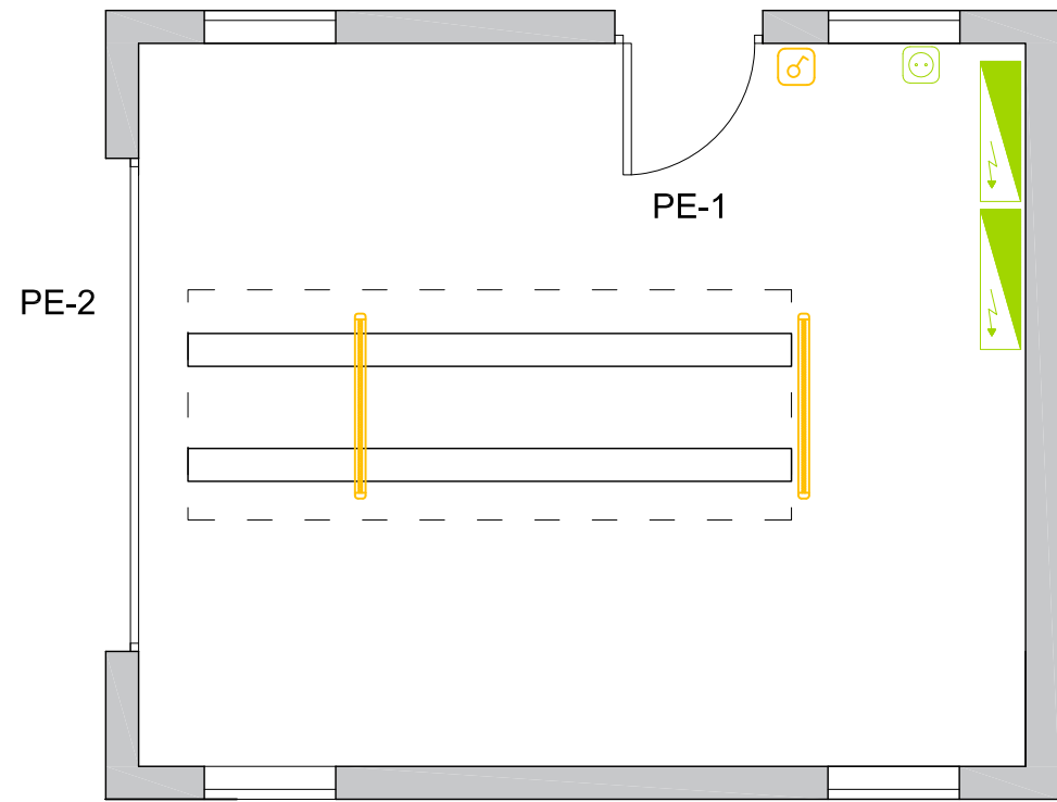
PLANTA ELECTRICITAT
