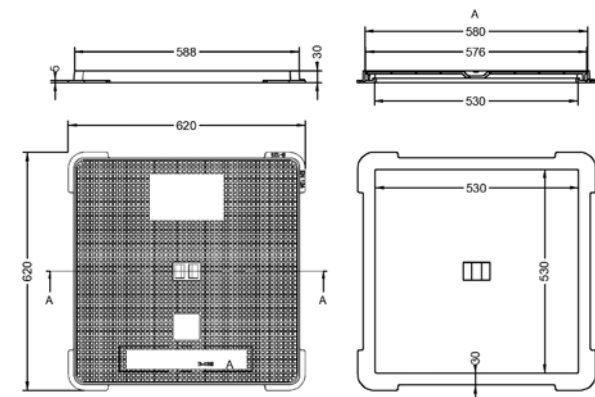
TAPA ARQUETA 60X60CM
