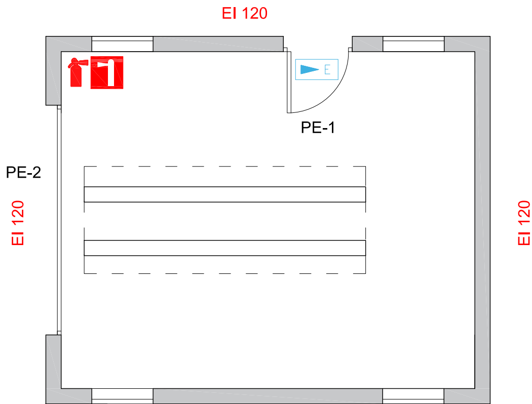
PLANTA INCENDIS
