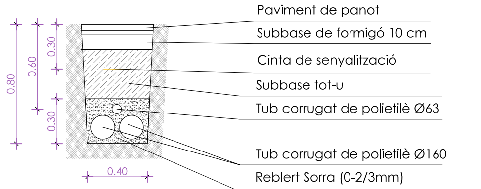
DETALL RASA 2Ø160 + 1Ø63 - AMB ACABAT AMB PANOT
