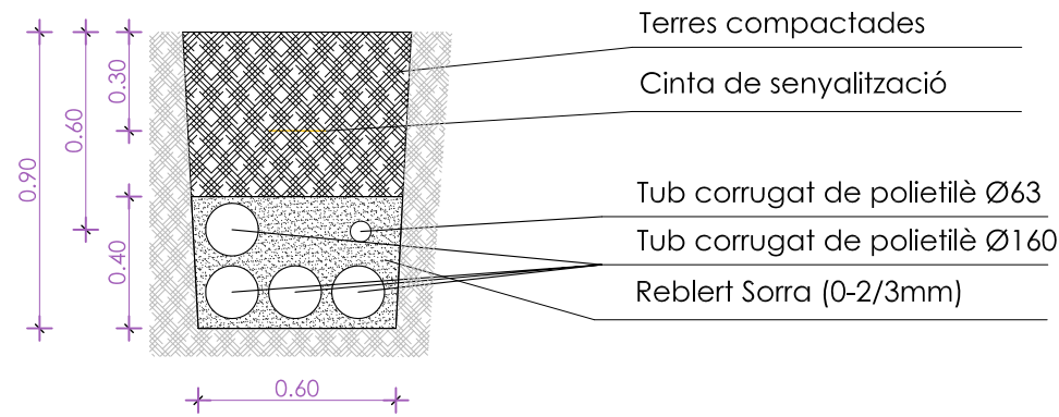
DETALL RASA 4Ø160 + 1Ø90 + 1Ø63 - AMB ACABAT DE TERRES
