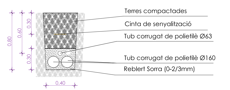
DETALL RASA 2Ø160 + 1Ø63 - AMB ACABAT DE TERRES
