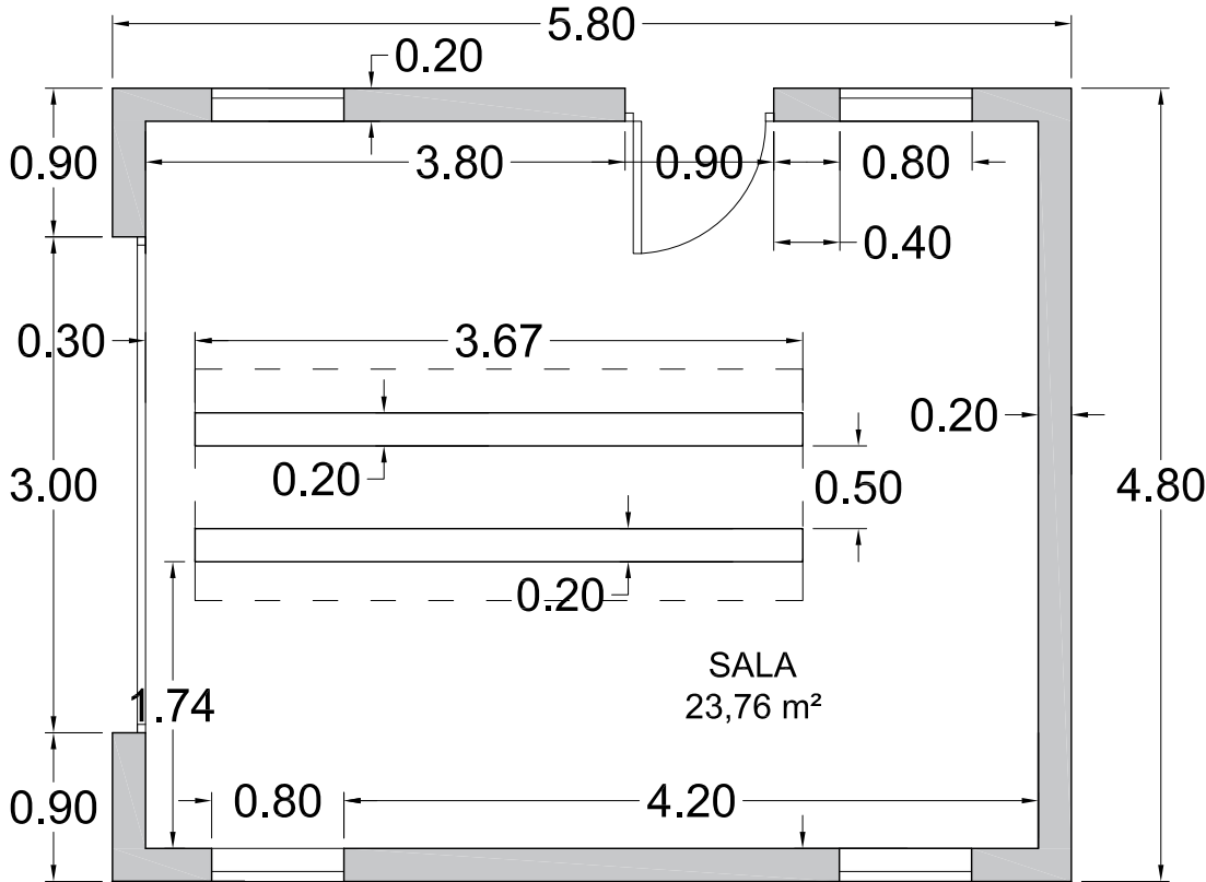
PLANTA COTES
