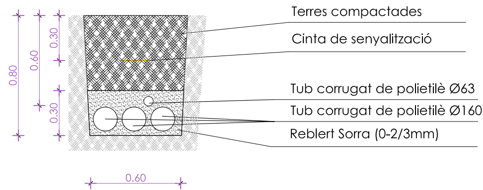
DETALL RASA 3Ø160 + 1Ø90 + 1Ø63 - AMB ACABAT DE TERRES
