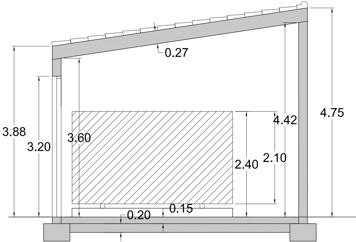
SECCIÓ
