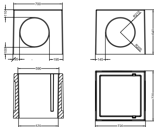
ARQUETA 60X60CM
