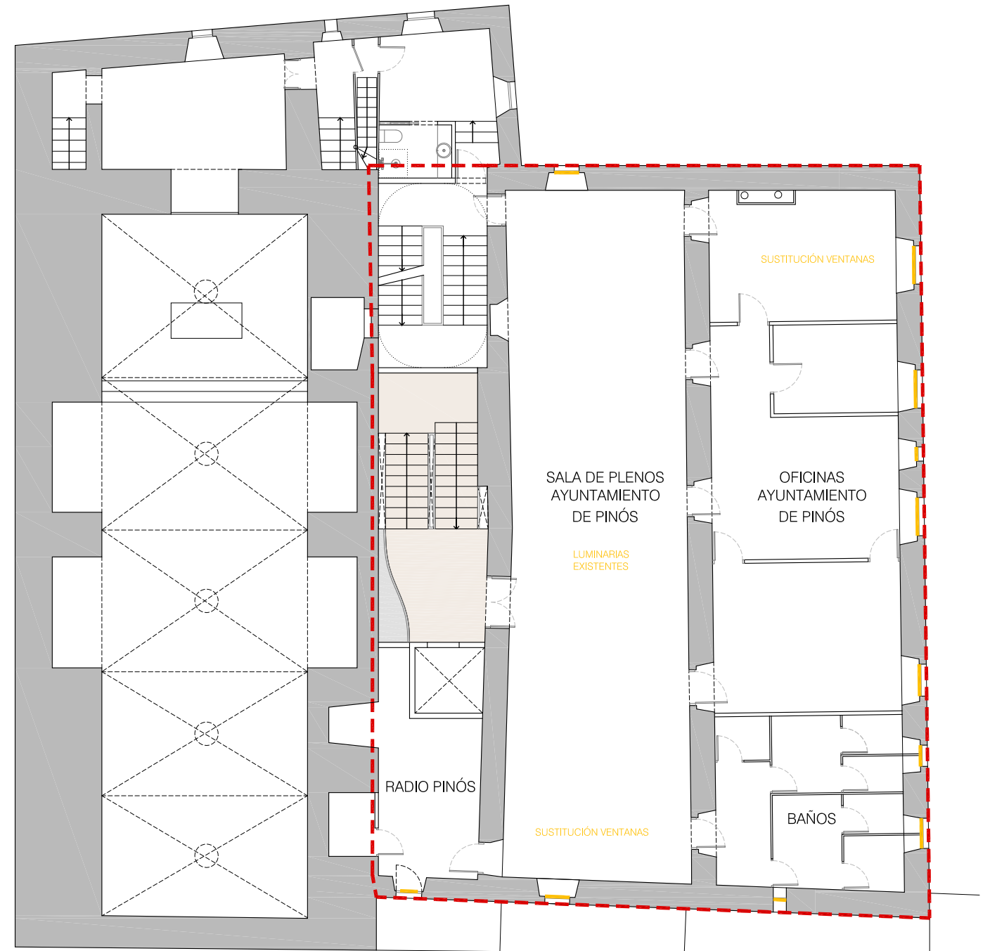
PLANTA 1
