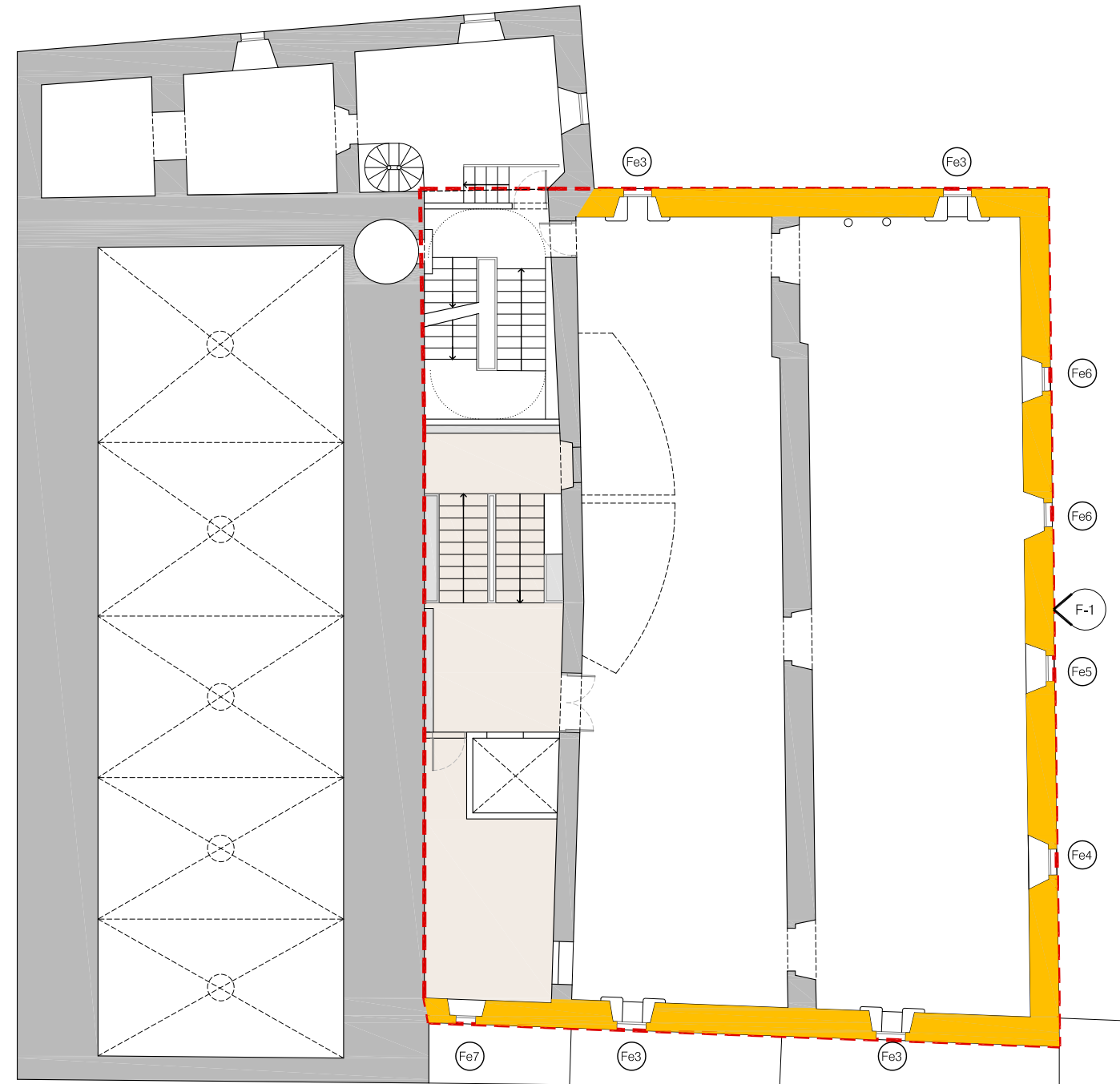
PLANTA 2
