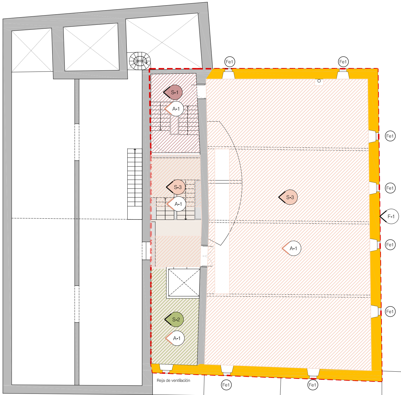
PLANTA 3
