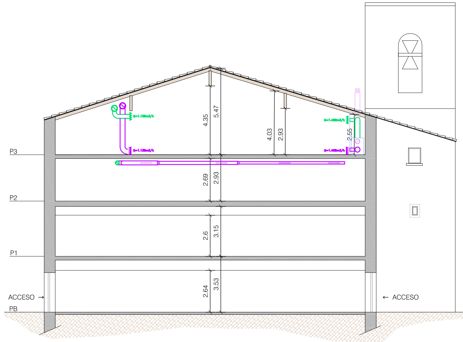
SECCIÓN LONGITUDINAL 2
