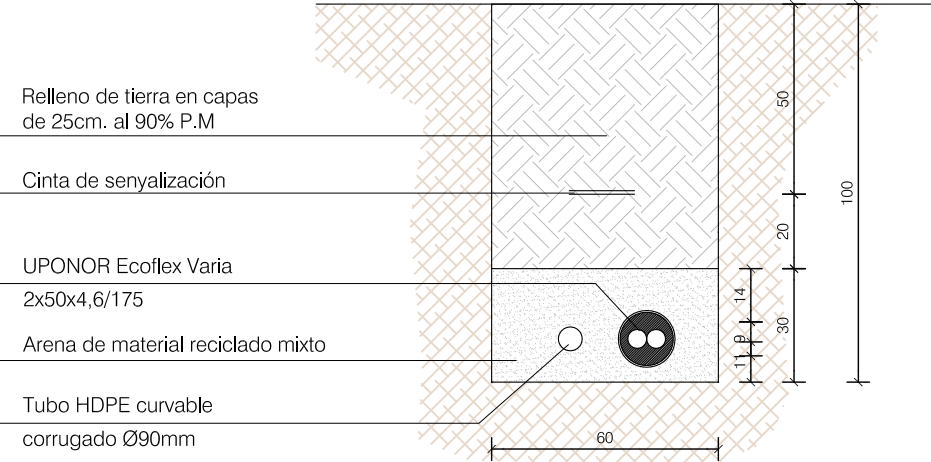
DETALLE ZANJA CONEXIÓN INSTALACIONES (ESCALA 1:25 - COTAS EN CM)
