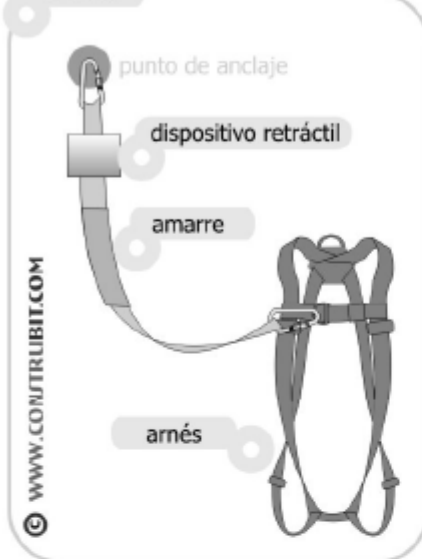
retráctil
