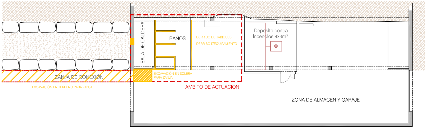
PLANTA SEMISOTANO - LOCAL SOCIAL
