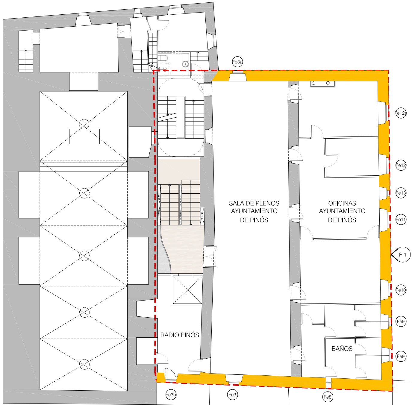
PLANTA 1
