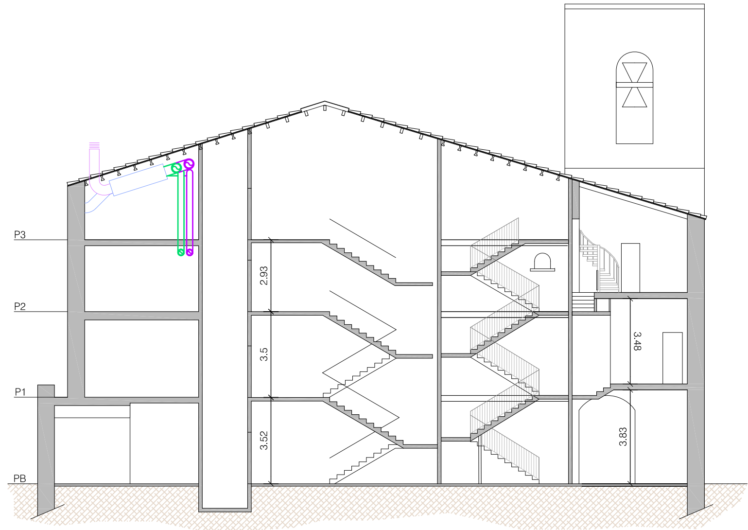
SECCIÓN LONGITUDINAL 1
