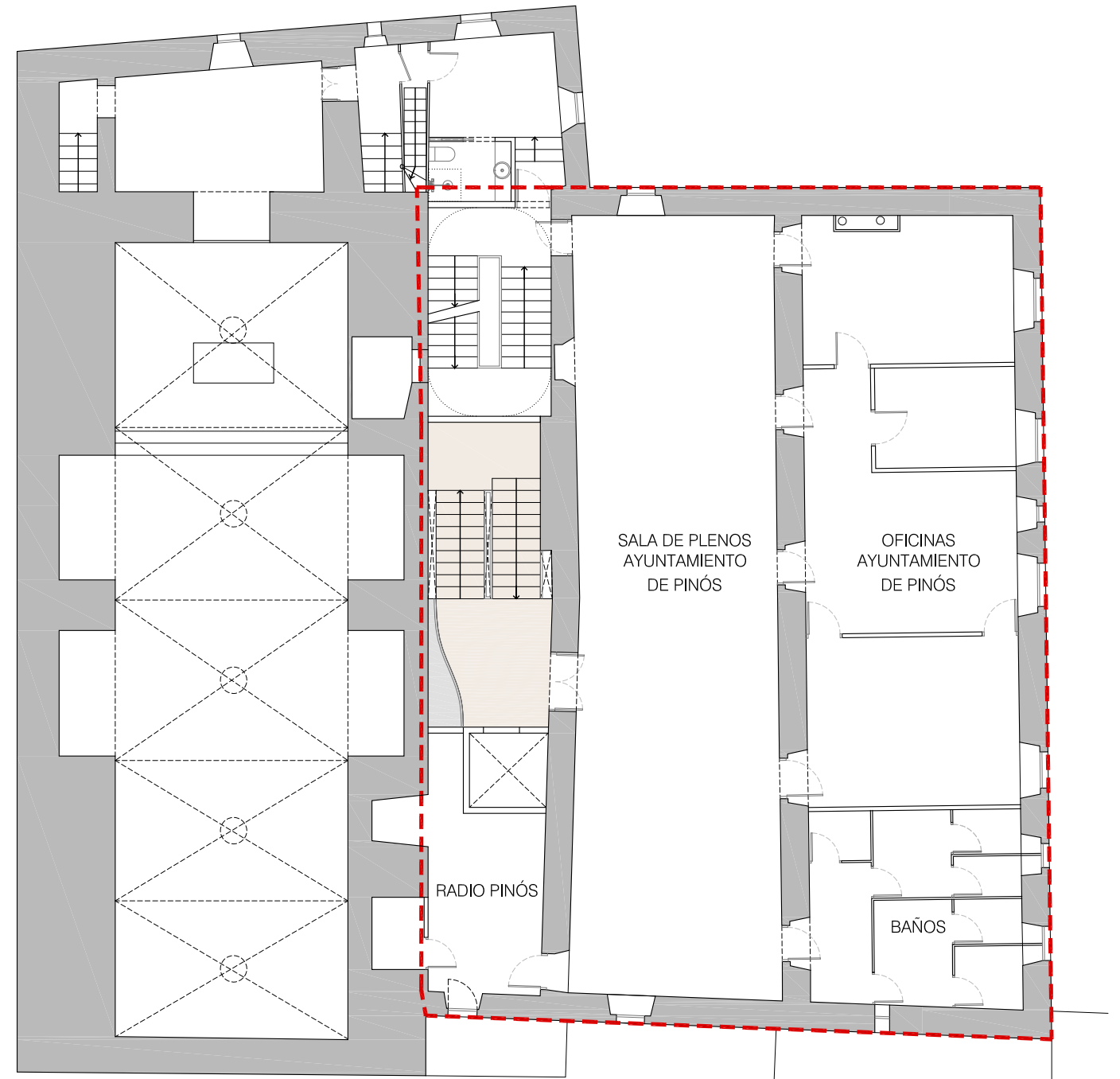
PLANTA 1
