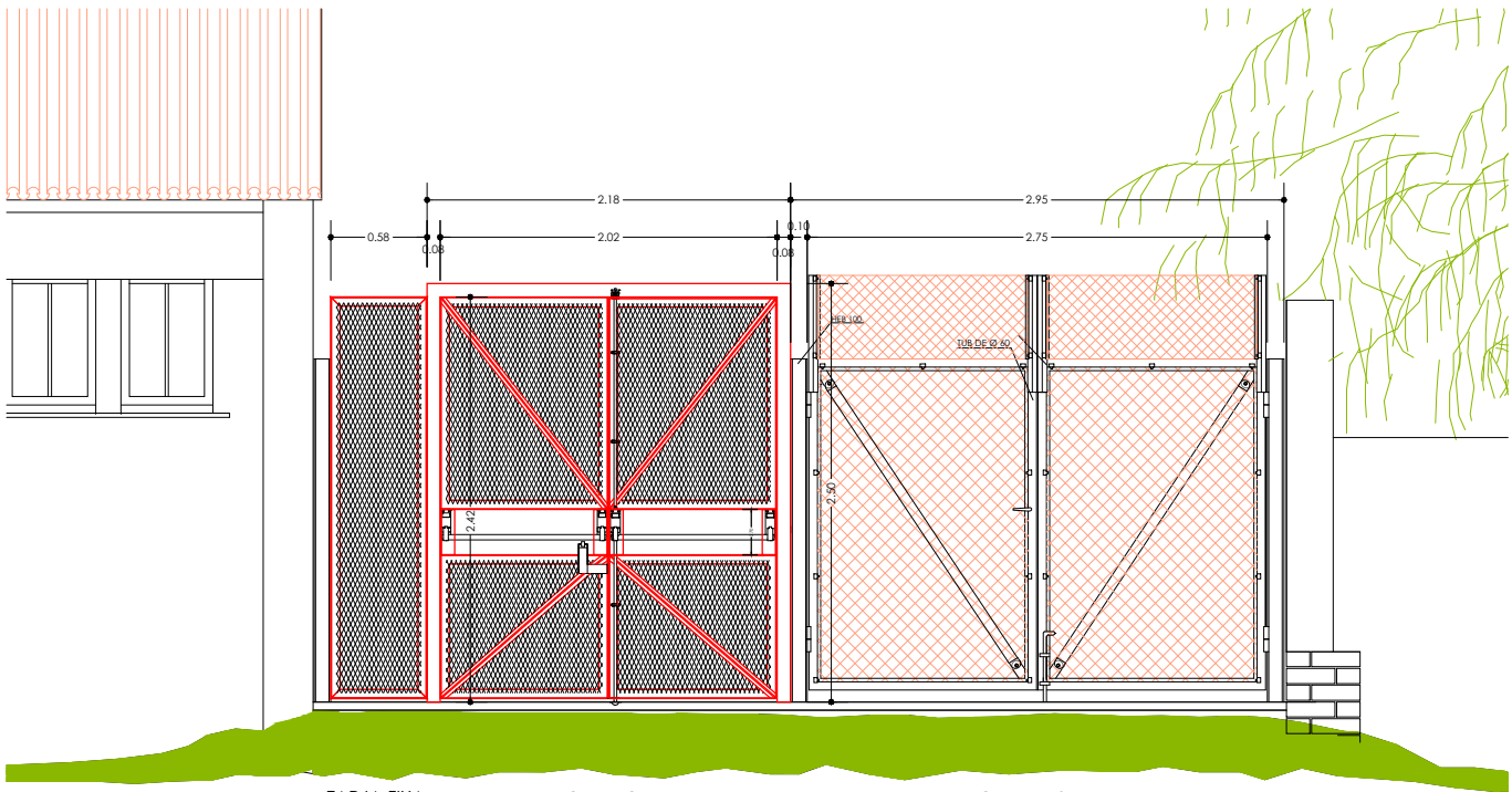
TARJA FIXA NOVA PORTA DOBLE FULLA 2,00 m CAP. EVAC. 2x600 =1200 p PORTA EXISTENT DOBLE FULLA 2,75 m MANTENIMENTS
