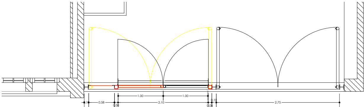
TARJA FIXA NOVA PORTA DOBLE FULLA 2,00 m CAP. EVAC. 2x600 =1200 p PORTA EXISTENT DOBLE FULLA 2,75 m MANTENIMENTS
