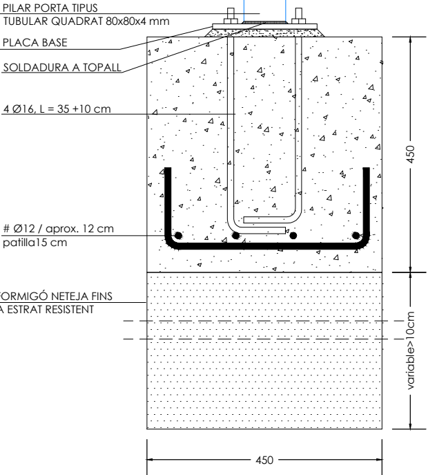
SABATA TIPUS (RECTANGULAR O QUADRADA)
