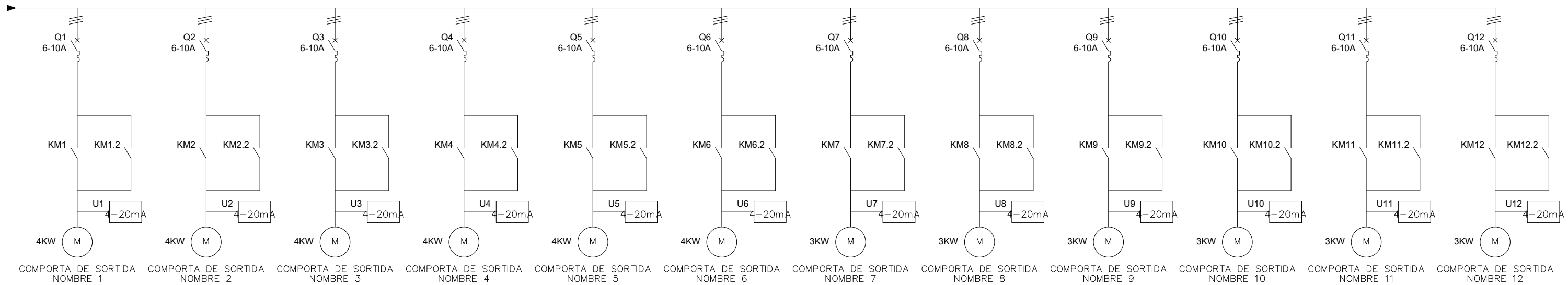
LINIES UNIFILARS COMPORTES DE SORTIDA
