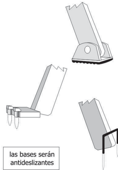
zapatasy anclajes
