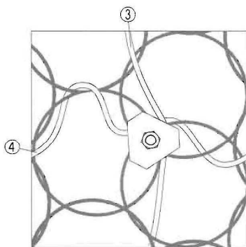
Detalle de anclaje intermedio
