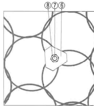
Detalle de anclaje adicional
