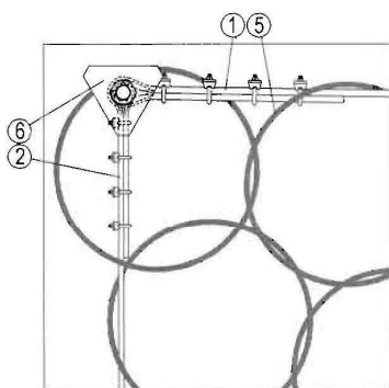
Detalle de anclaje en los extremos
