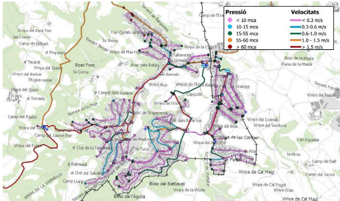
Figura 45. Model de consum de la xarxa actual amb consums punta futurs
