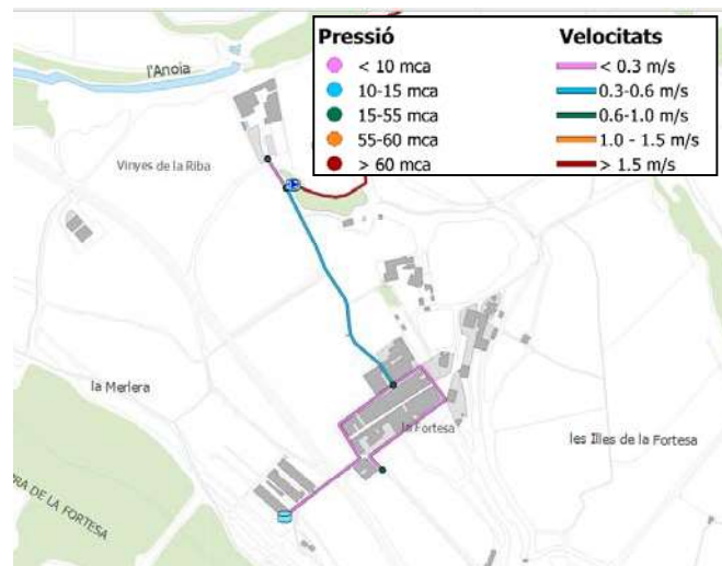
Figura 46. Model de consum de la xarxa actual amb consums punta futurs
