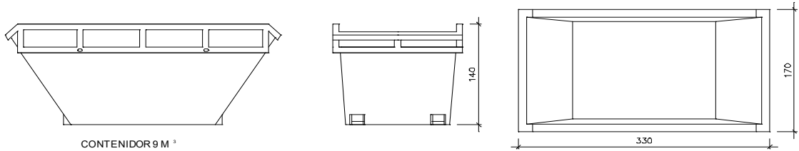
CONTENIDOR 9 M 3
