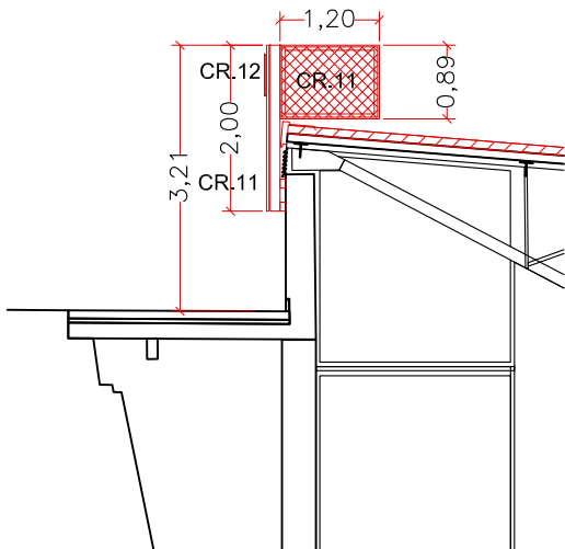
SECCIO TRANSVERSAL
