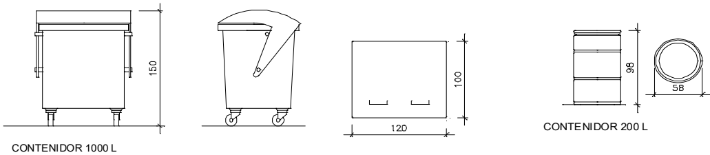
CONTENIDOR 1000 L
