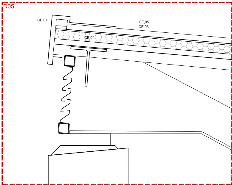
SECCIO LONGITUDINAL
