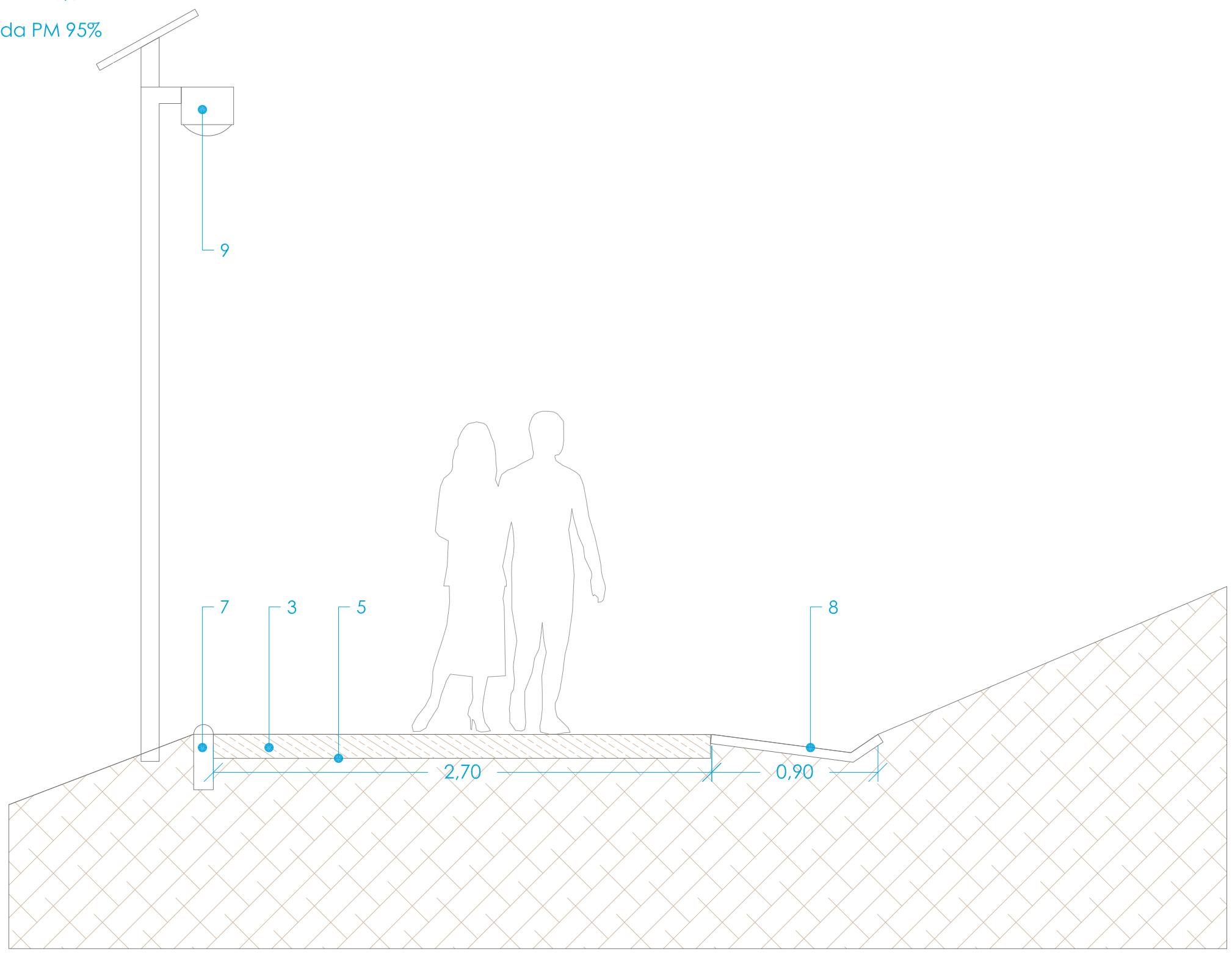
secció 3. proposta
