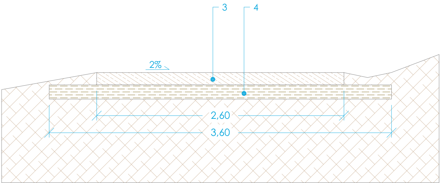
secció 1. proposta
