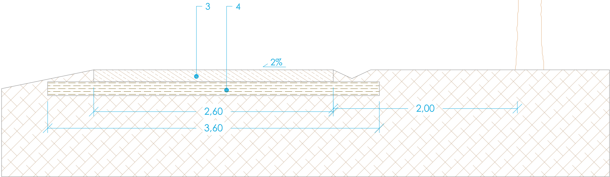
secció 2. proposta
