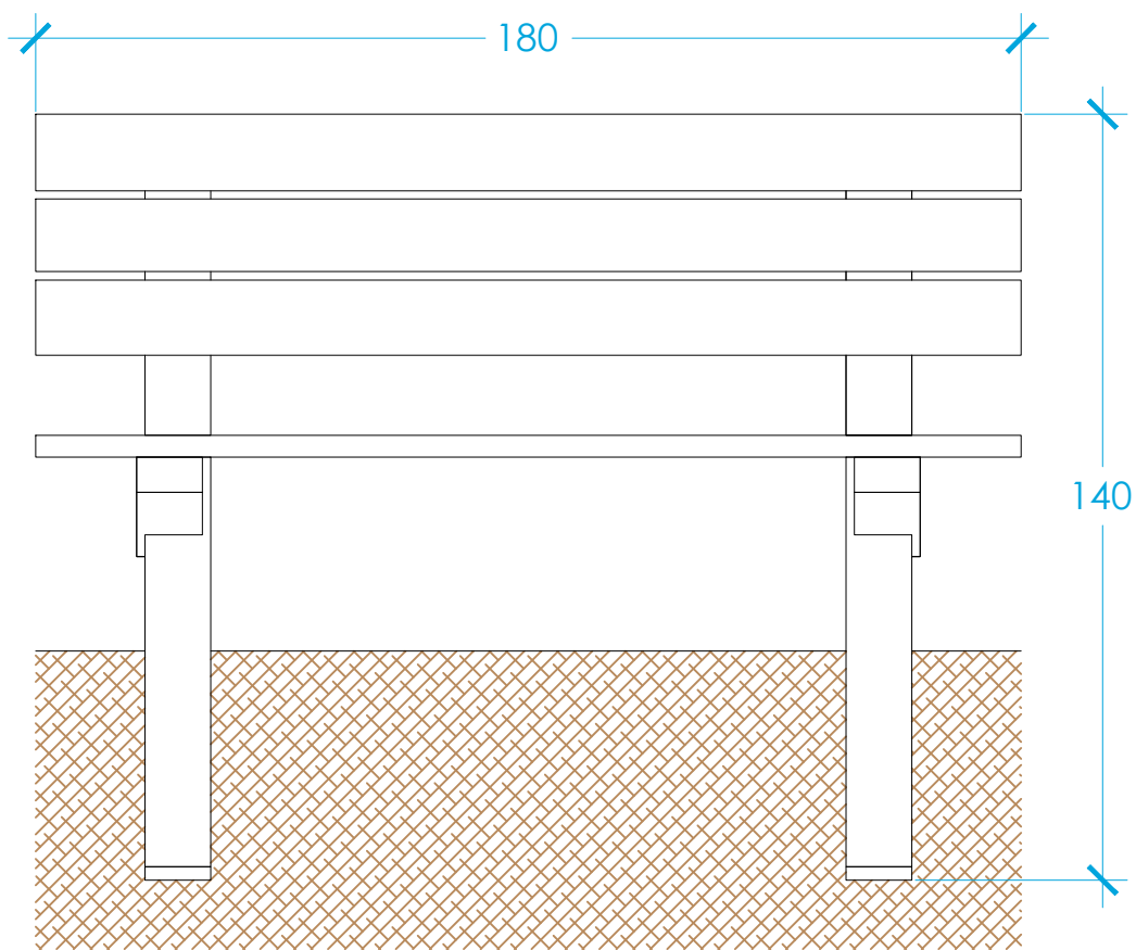
alçat frontal
