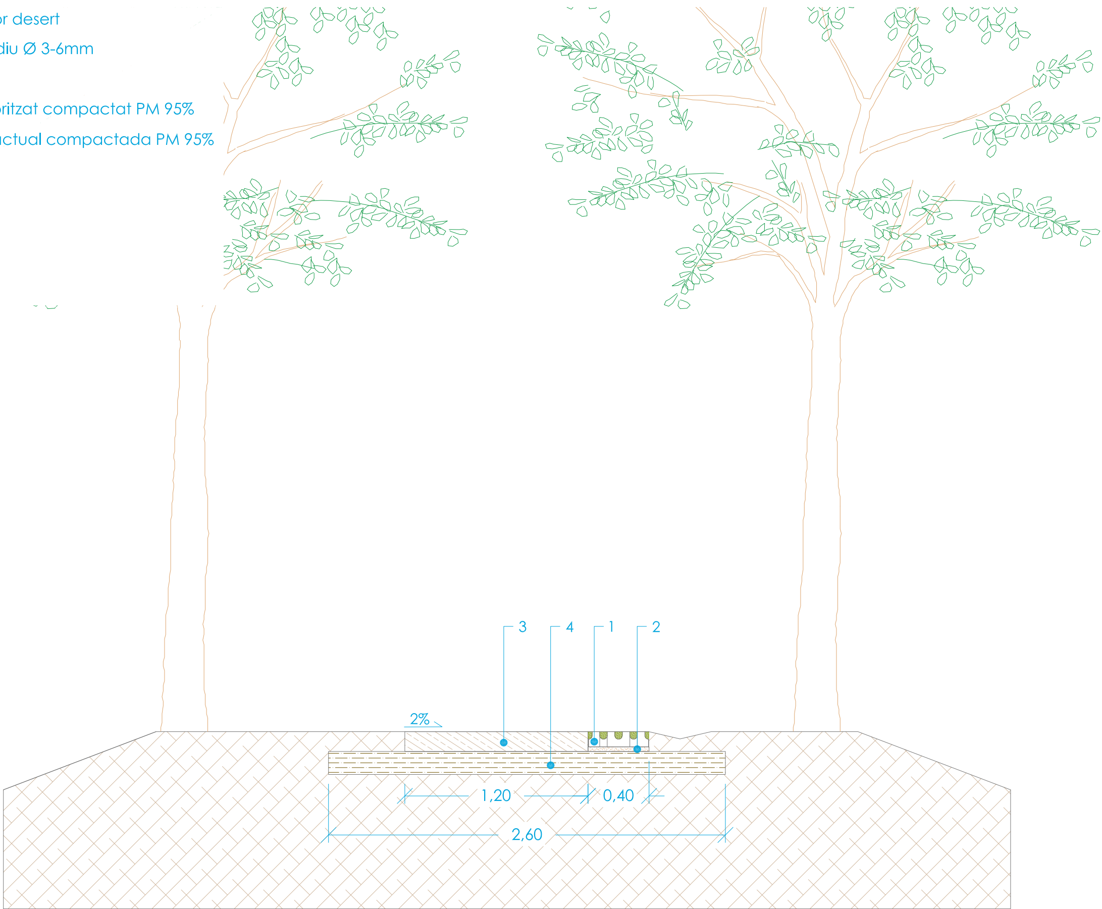
secció 6. proposta
