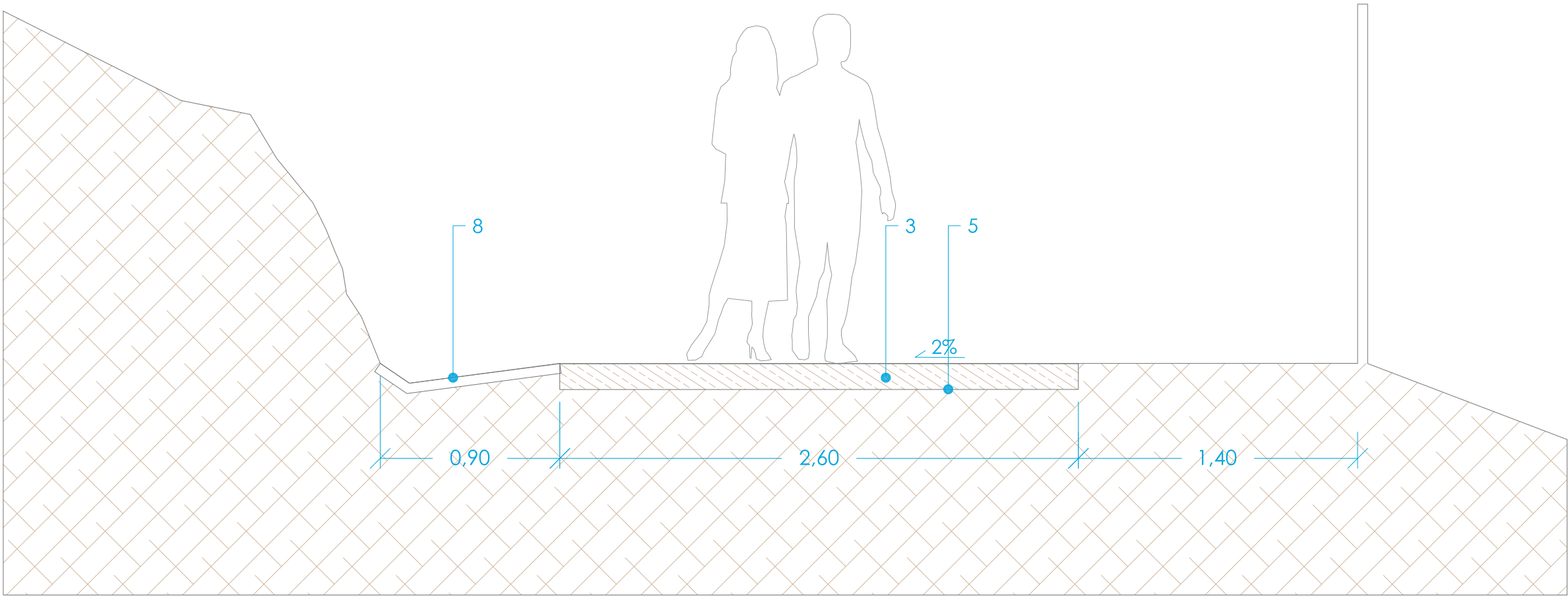
secció 5. proposta
