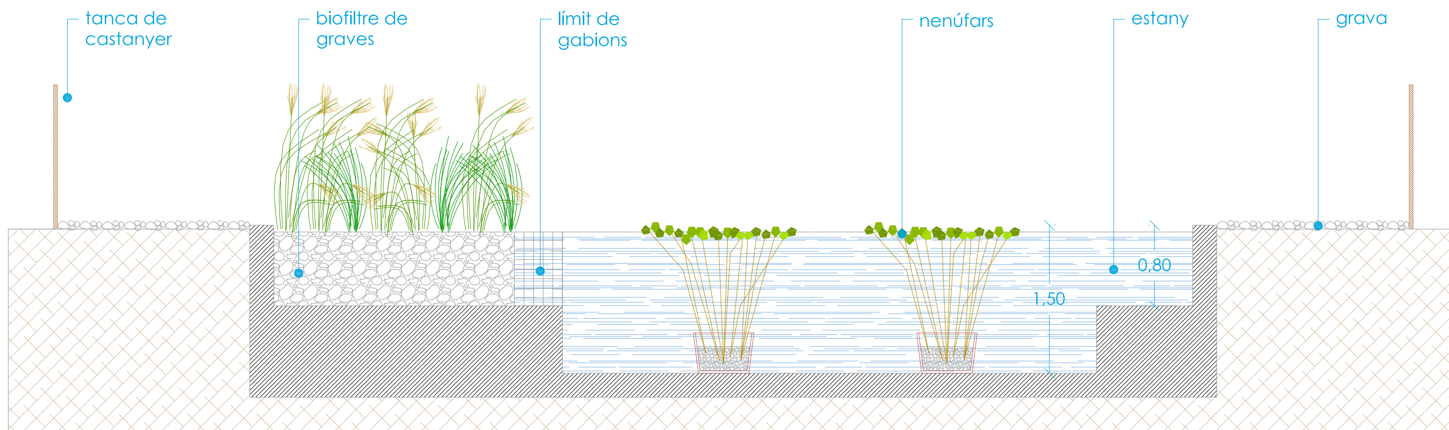
bassa proposta
