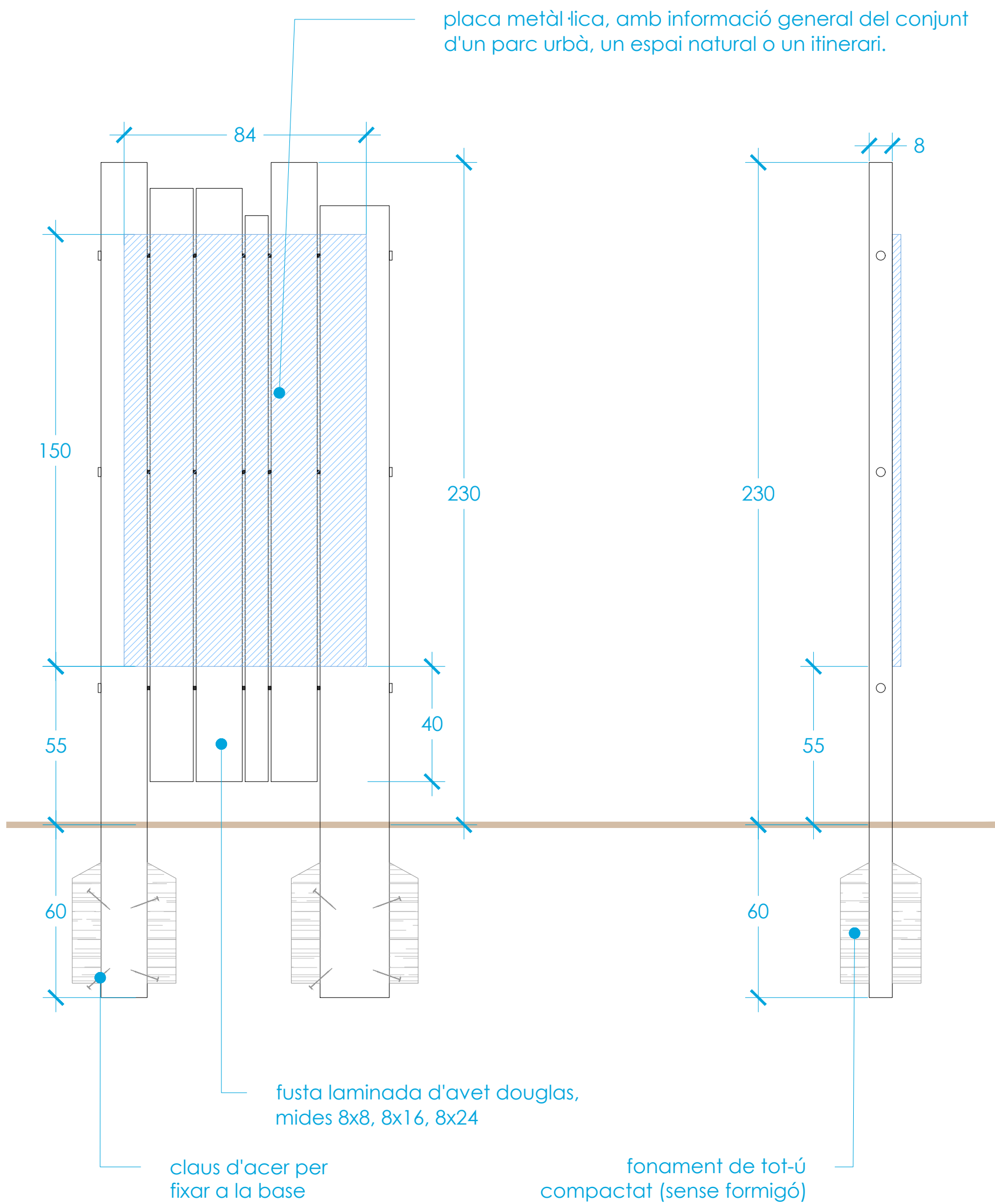
alçat frontal
