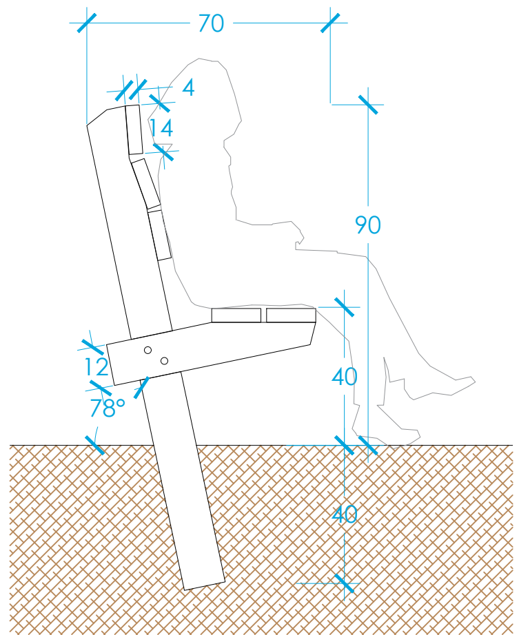
alçat lateral
