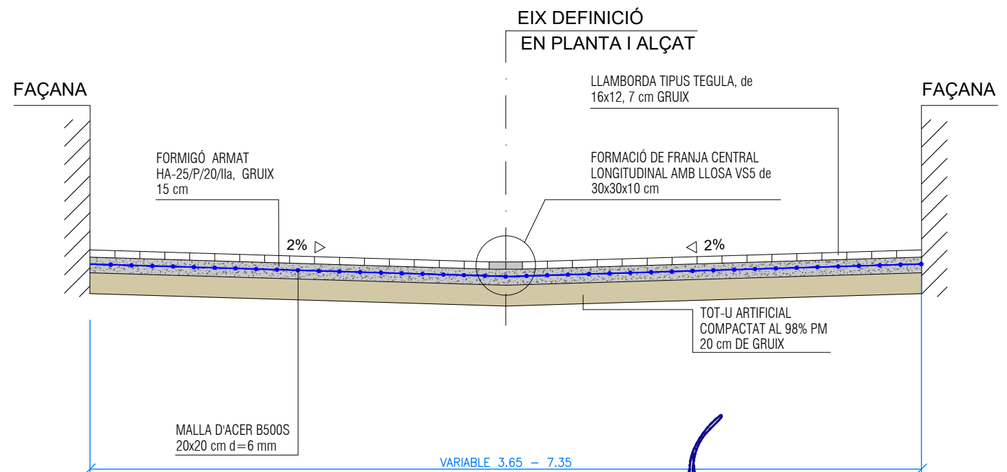
SECCIÓ B-B
