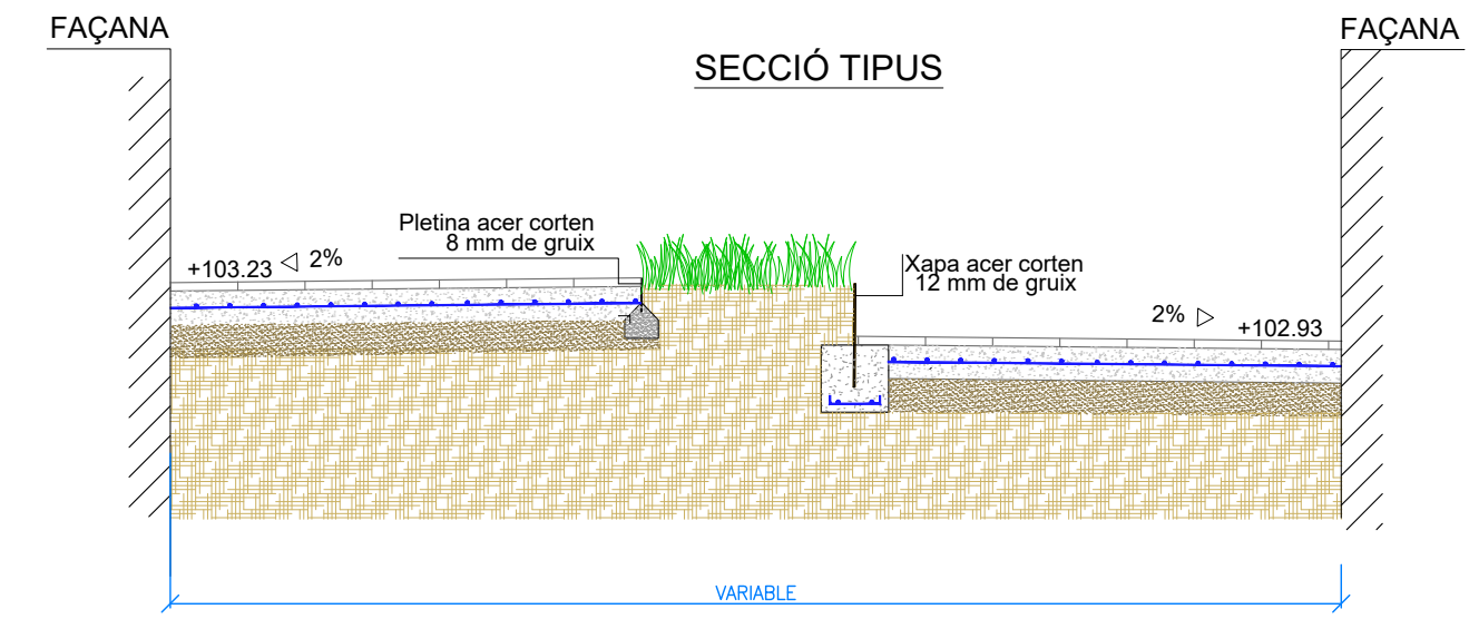
SECCIÓ A-A
