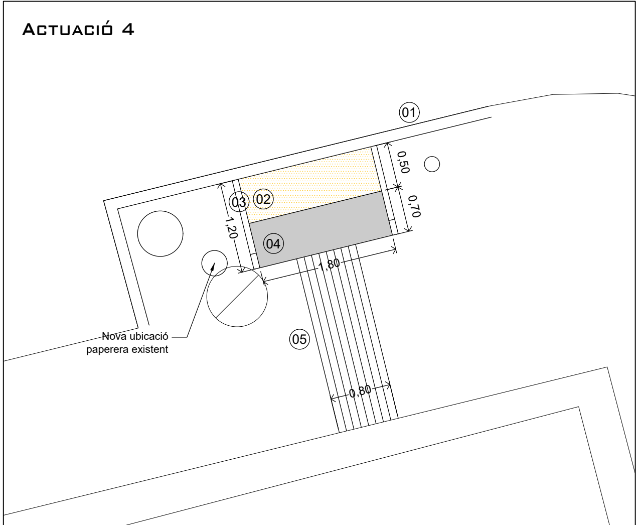
INTERVENCIÓ 3 E:1/50
