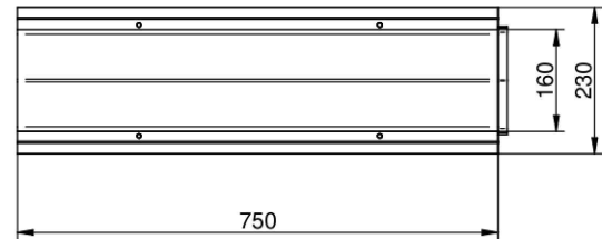
CANAL RC20 DE BENITO O EQUIVALENT
