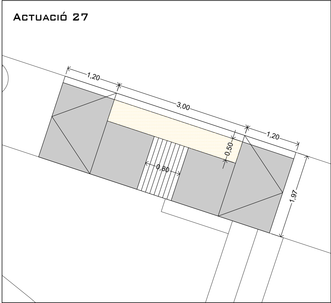
PLANTA GENERAL E:1/200
