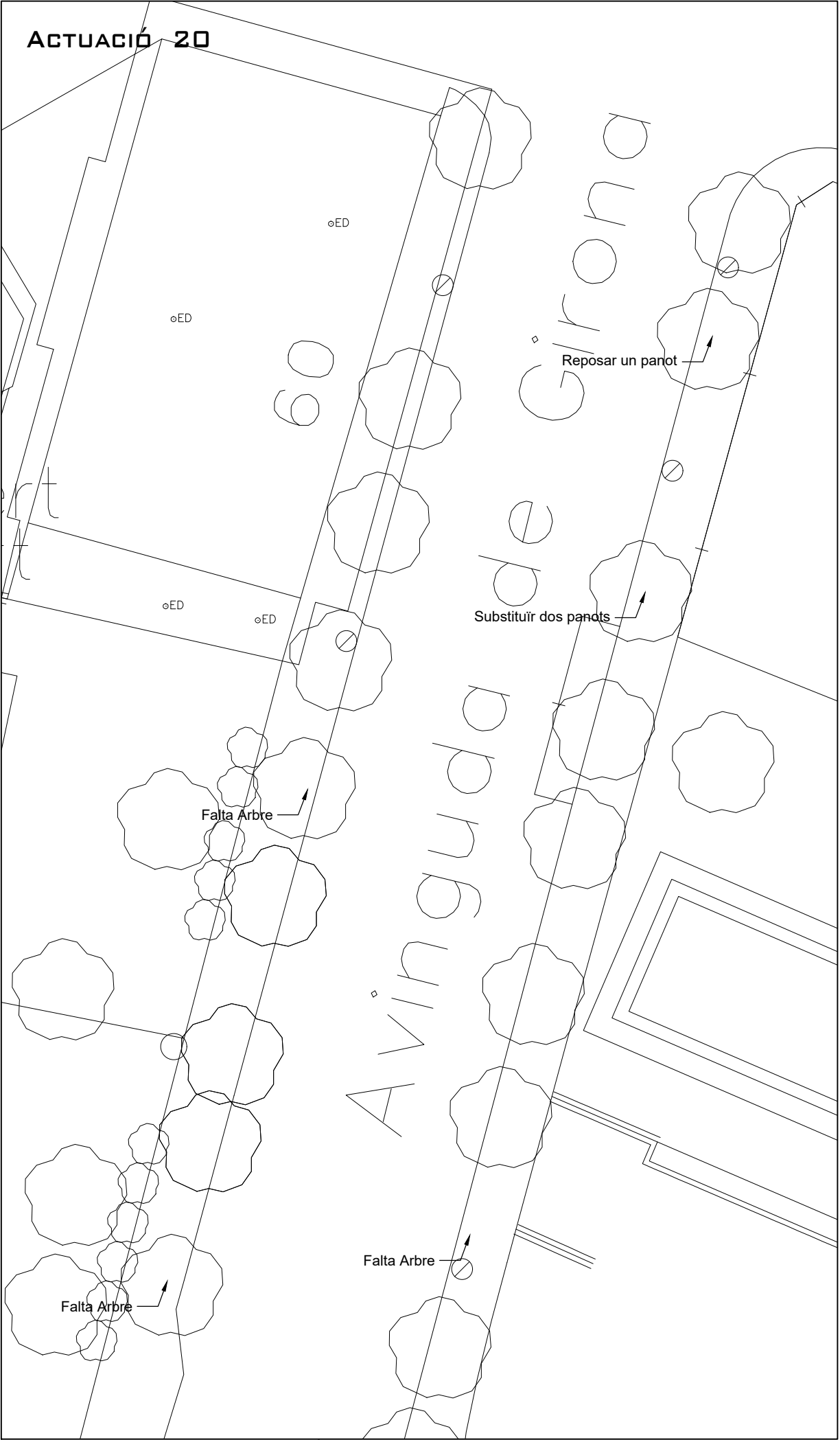
PLANTA GENERAL E:1/200
