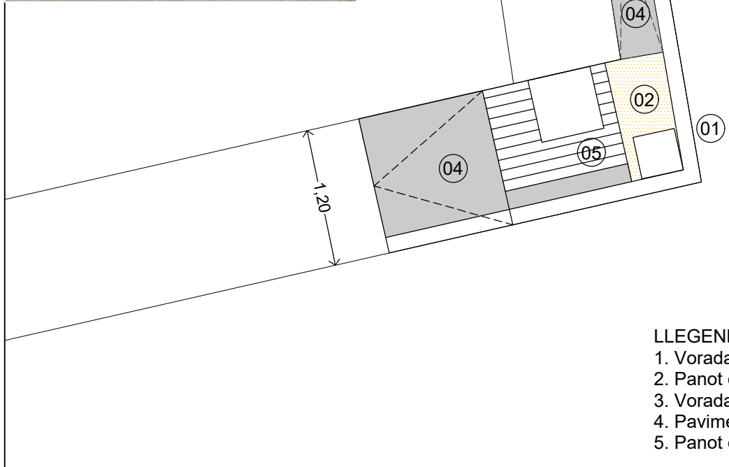
INTERVENCIÓ 1 E:1/50
