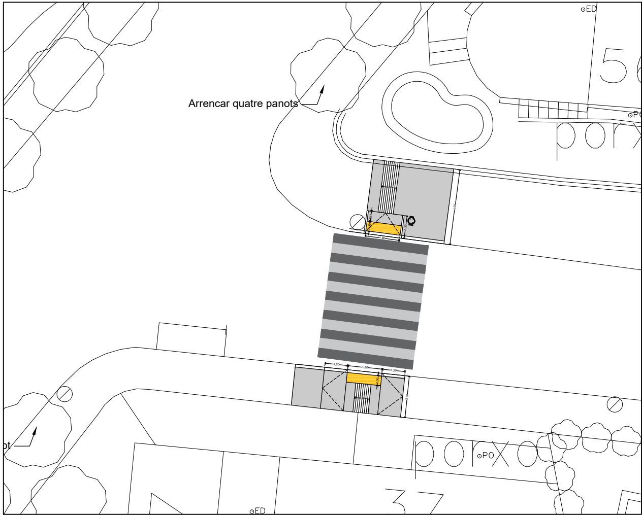
PLANTA GENERAL ESTAT PROPOSTA1/200
