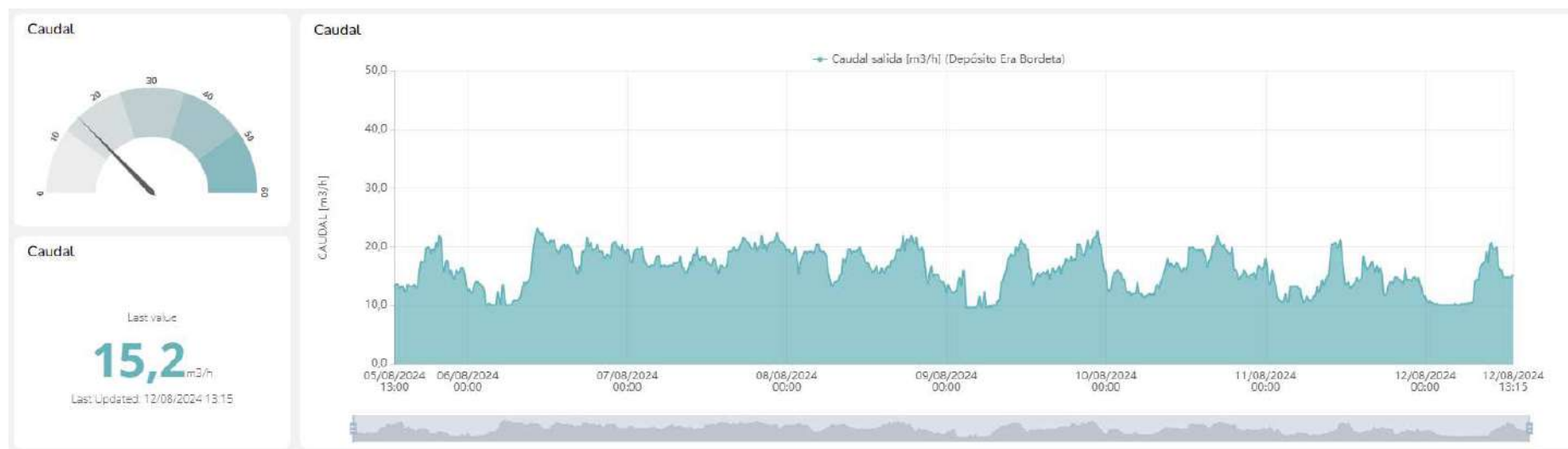
Imatge 05. Dades de cabal de sortida del dipòsit d'Era Bordeta.
