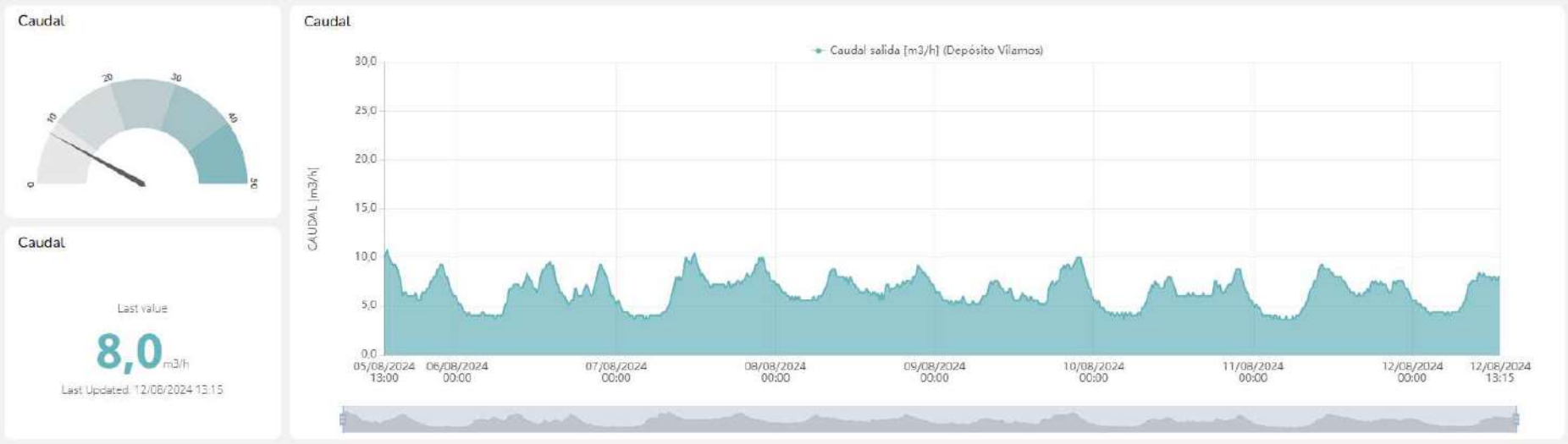
Imatge 03. Dades de cabal de sortida del dipòsit de Vilamòs.
