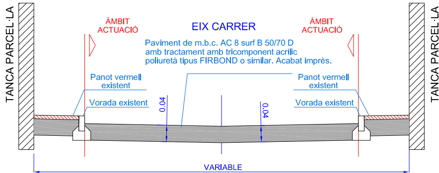
SECCIÓ TIPUS A - A' - NOU PAVIMENT DE FORMIGÓ
