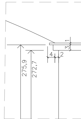
DETALL D3 e.1/10
