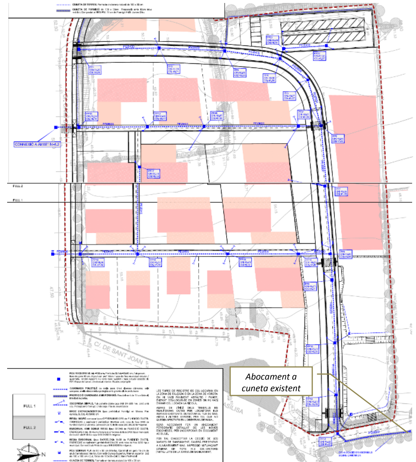
Figura 48. Proposta de xarxa aigües plujals en l'àmbit IV 6.1.
