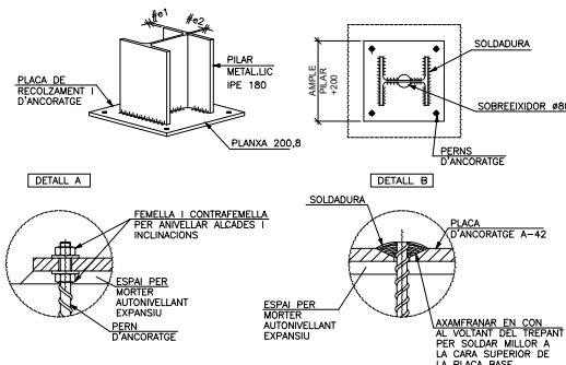
Placa d'ancoratge
