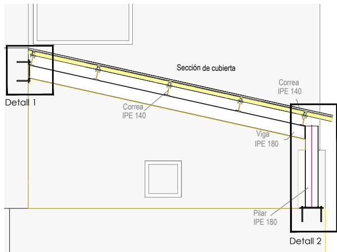
Secció coberta
