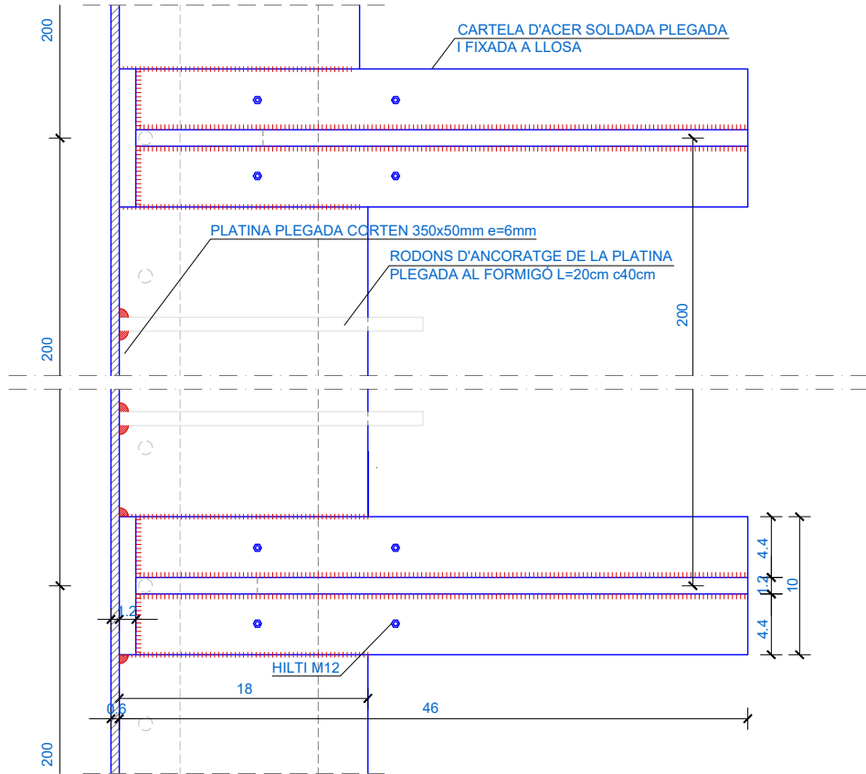
PLANTA DETALL FIXACIÓ BARANA E 1/5
