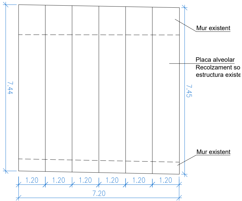
Detall forjat plaques alveolars E1/100
