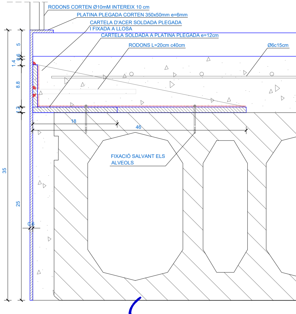
DETALL FIXACIÓ BARANA E 1/5
