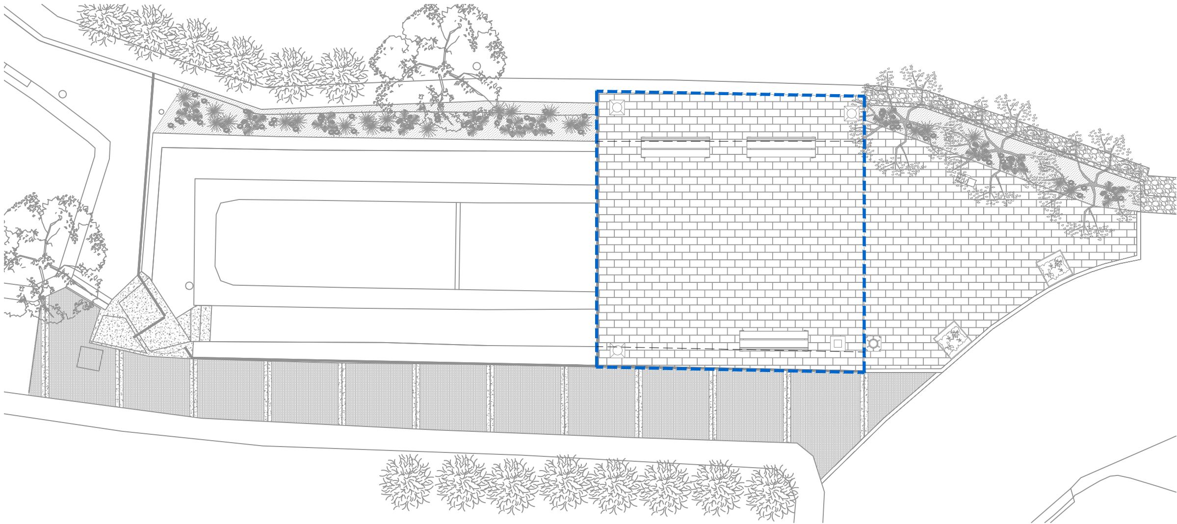
Detall forjat plaques alveolars E1/100
