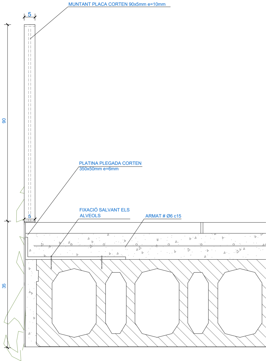
SECCIÓ TIPUS BARANA 90cm
