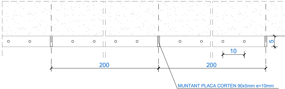
PLANTA DETALL INICI/FINAL BARANA
