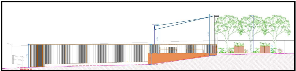
Alçat proposat per al mirador de l'antic escorxador a Bràfim, amb protecció dels antics rentadors.
