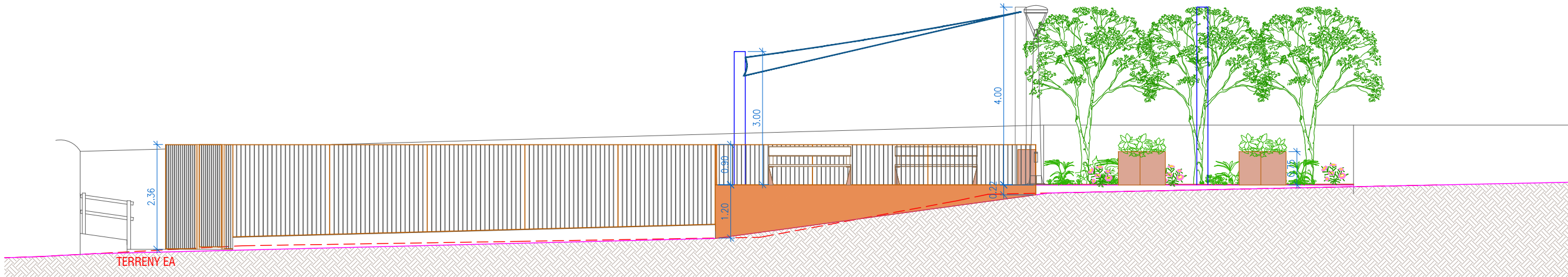
SECCIÓ B-B'
