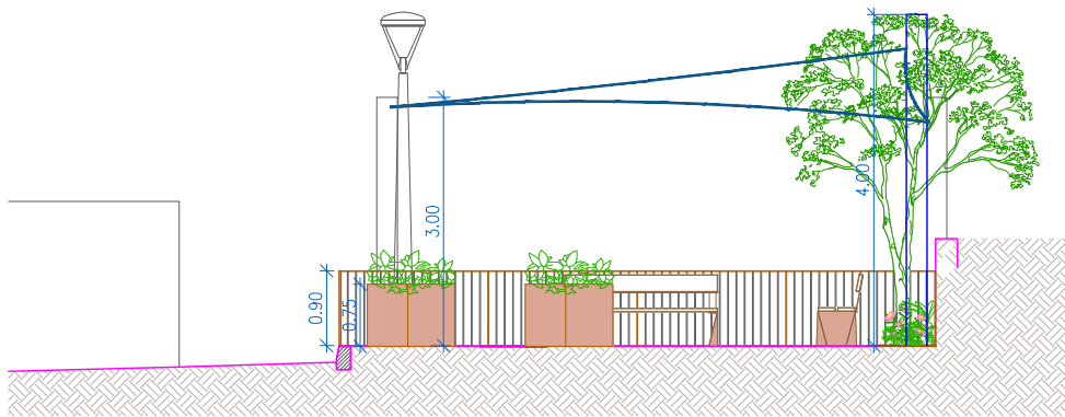
SECCIÓ A-A'
