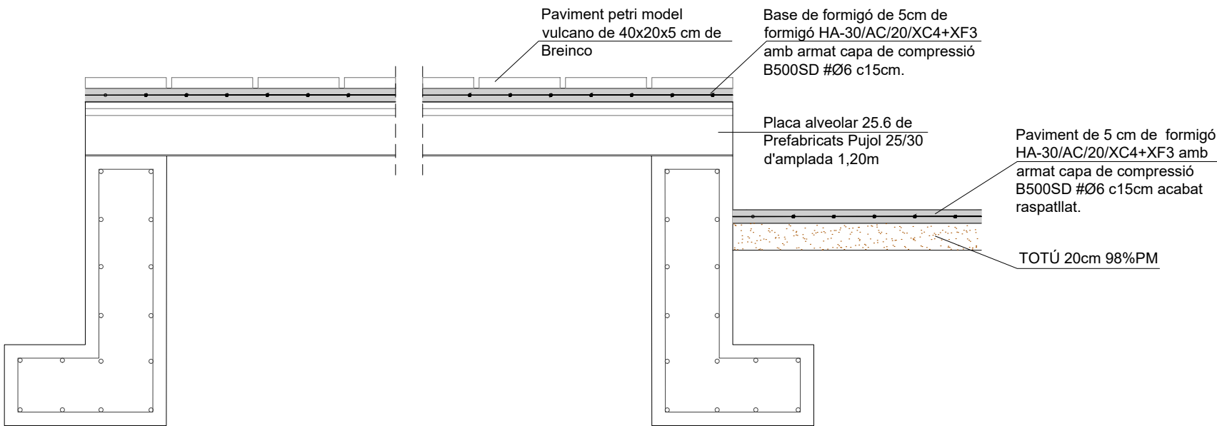
Detall forjat plaques alveolars E1/20
