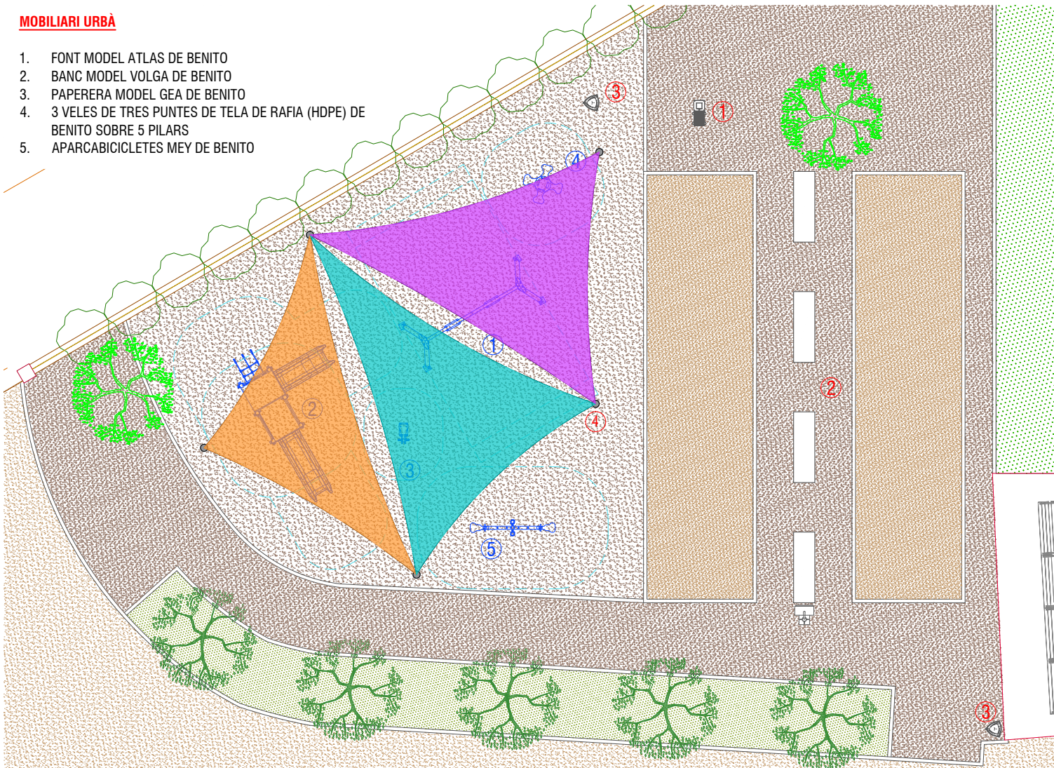
1. FONT MODEL ATLAS DE BENITO
