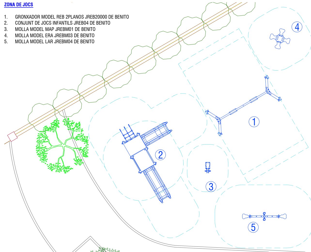
1. GRONXADOR MODEL REB 2PLANOS JREB20000 DE BENITO
