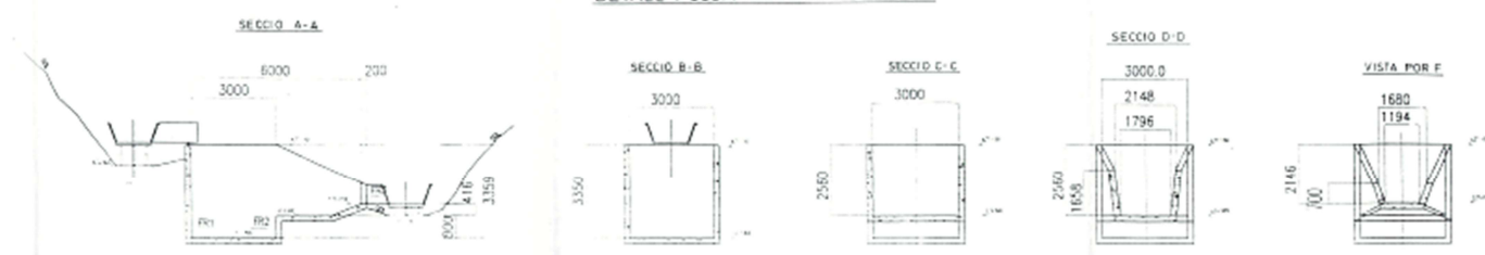
DETALL FOSSA RECEPCIÓ D'AIGUA
