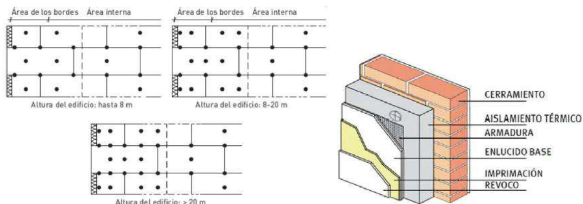
Figura 7. Imagen de la instalación de SATE en fachadas.
