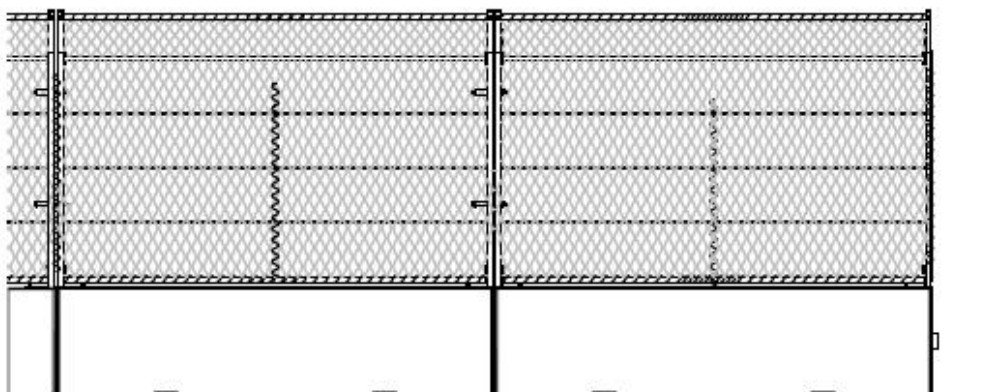
ALÇAT FRONTAL (reixa metàl·lica de seguretat amb obertura)
