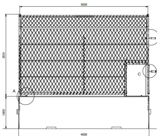
SECCIÓ TIPUS
