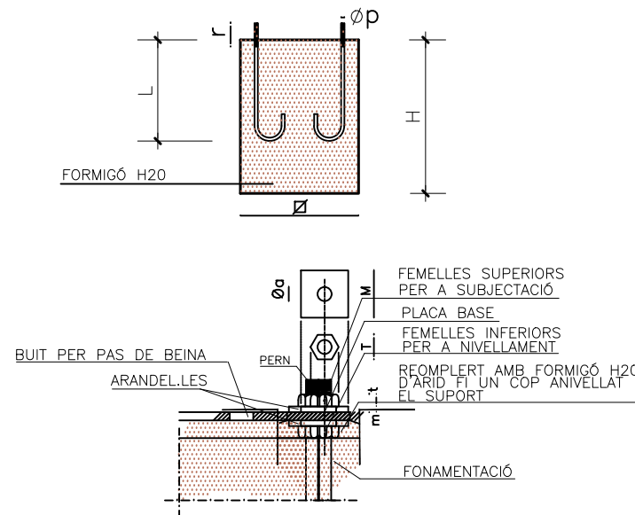
FONAMENTACIÓ I PERNS
