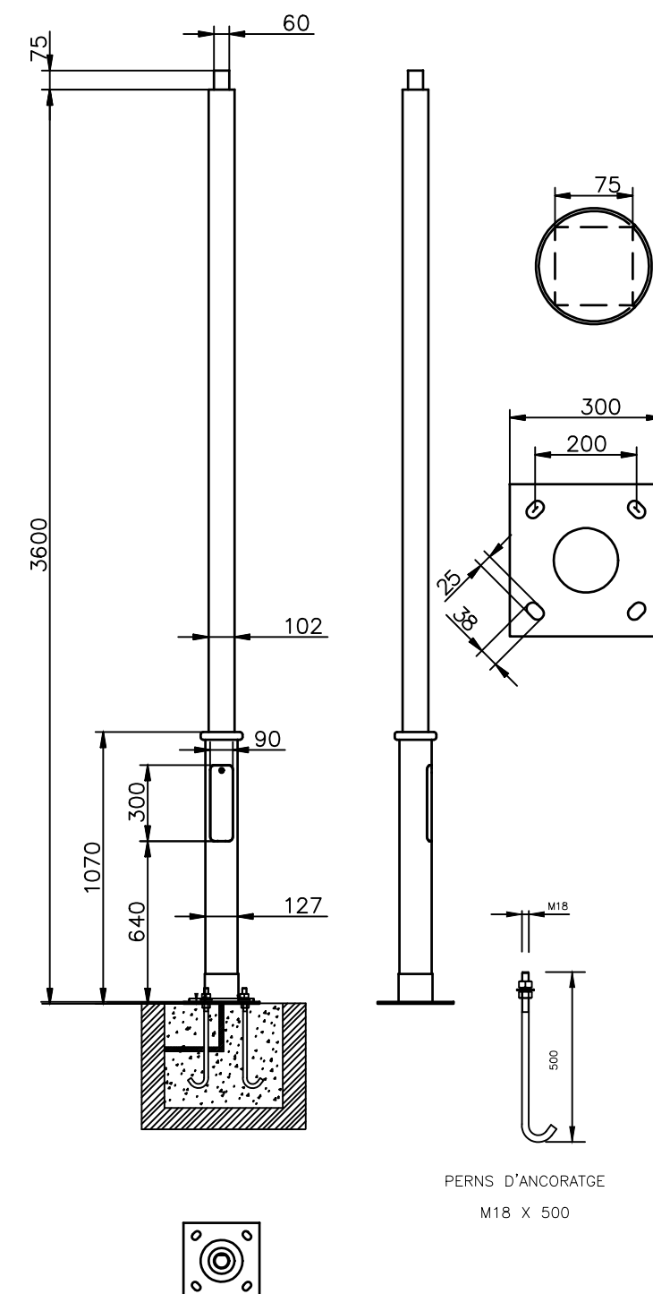
COLUMNA "OLSO 3,6" DE BENITO
