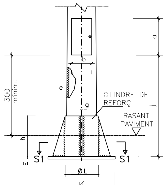
COLUMNA o BÀCUL TIPUS
