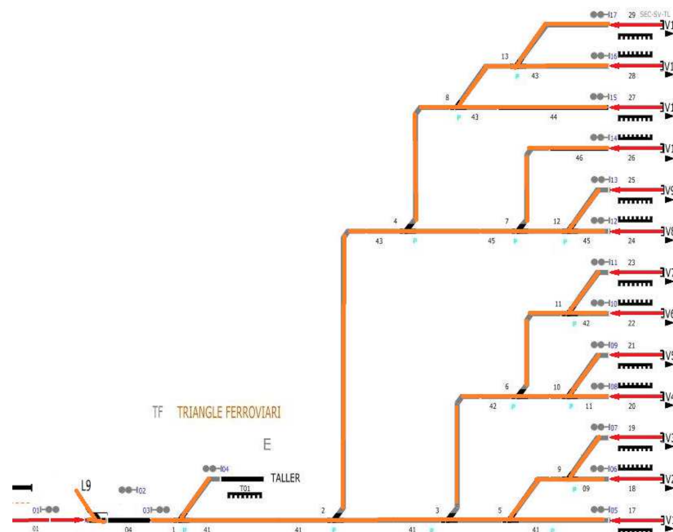
Figura 3. Orientació automàtica de CCV a Triangle Ferroviari.
