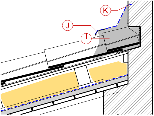
DETALL 2
