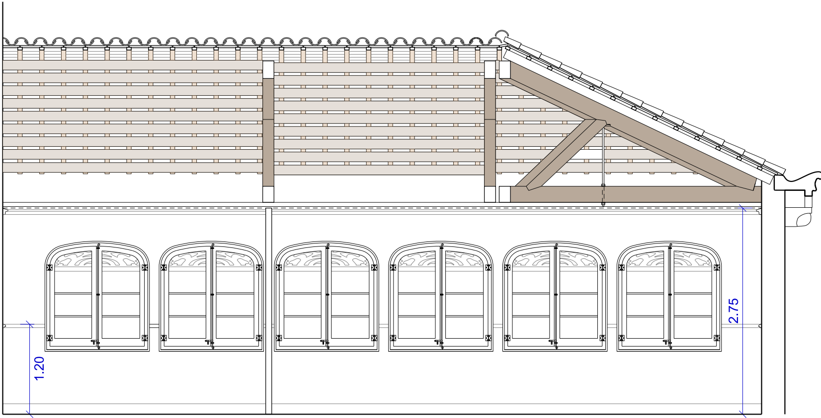
Secció / Alçat interior nord. E: 1/50
