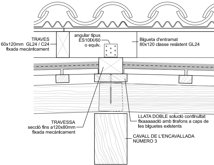
Secció detall canvi pendent coberta SD1 - E: 1/10
