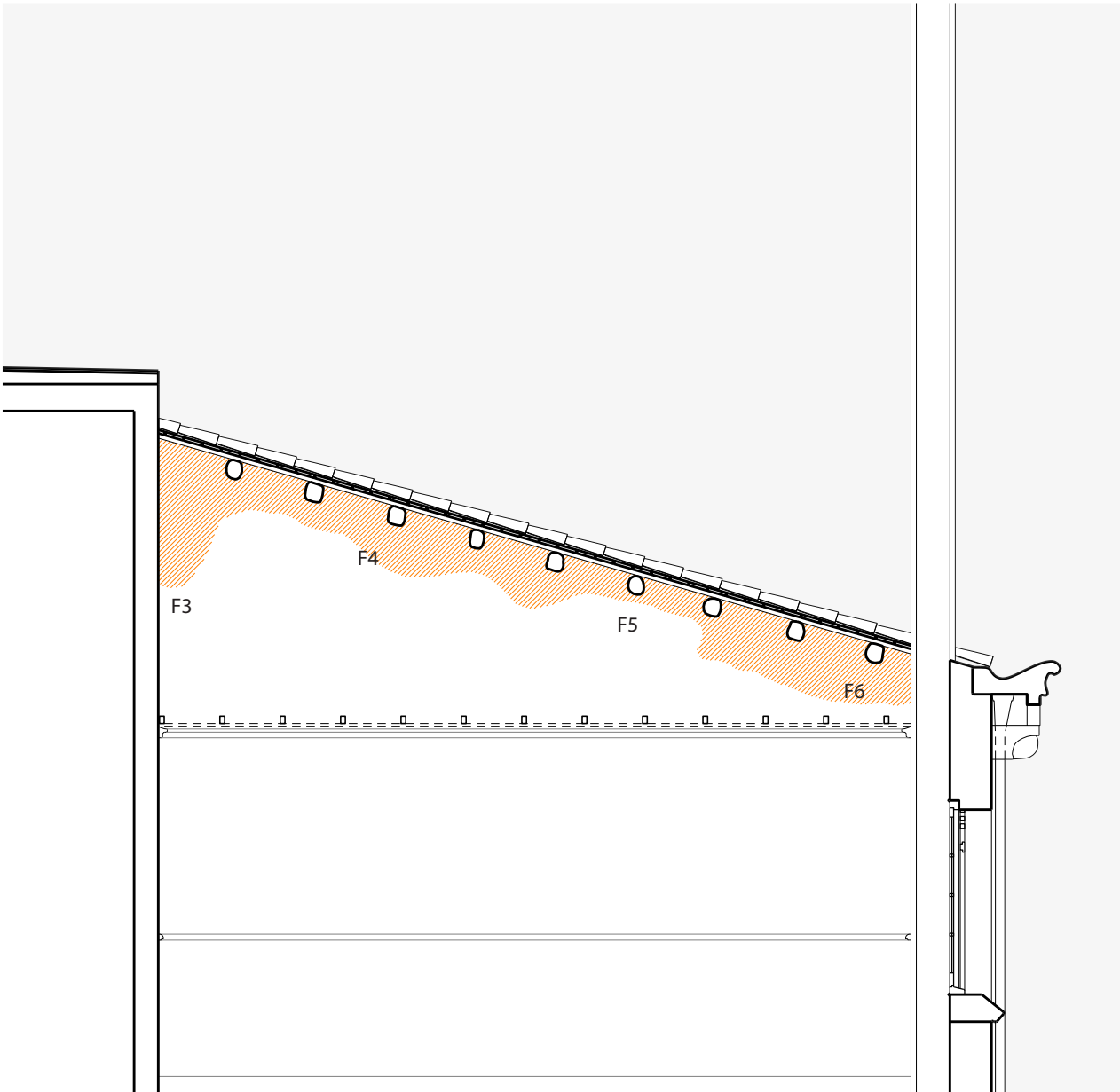
Secció / Alçat interior mitgera amb casa Gasull. E: 1/50
