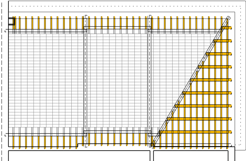
Enderrocs i desmuntatges. Bigues i llates. E: 1/50
