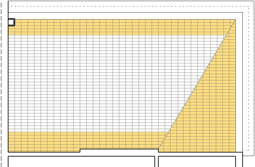
Enderrocs i desmuntatges. Tauler de rajols. E: 1/50
