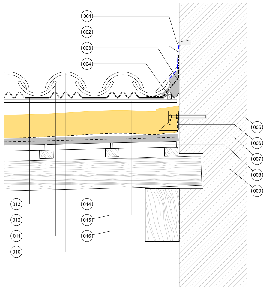
SECCIÓ DETALL A2 0 0.10 0.30m E:1/10 DIN A3 E:1/5 DIN A1
