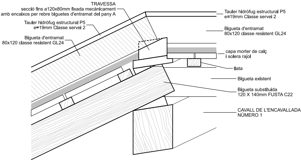
Secció detall canvi pendent coberta SD1 - E: 1/10
