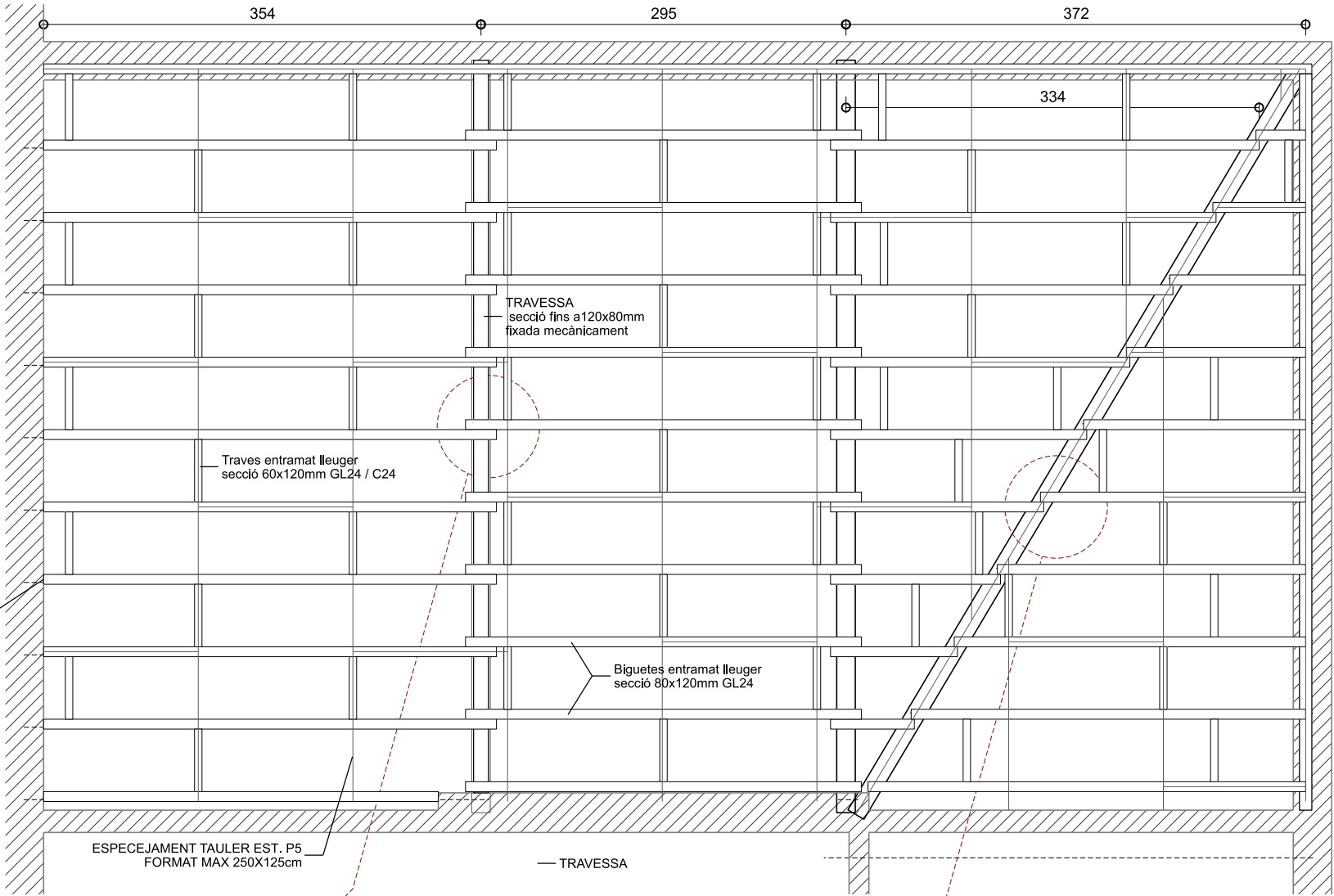
Planta entramat coberta. E: 1/50
