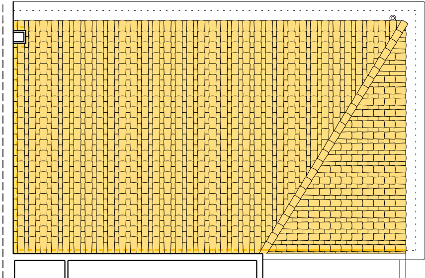
Enderrocs i desmuntatges. Teulada. E: 1/50
