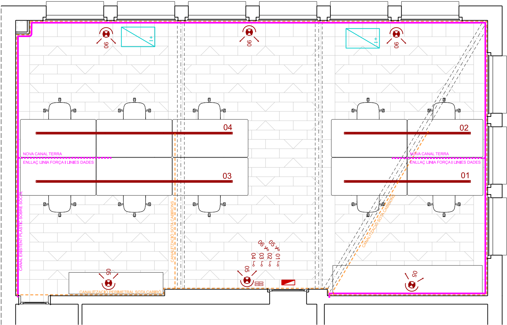
Planta instal·lacions. E: 1/50
