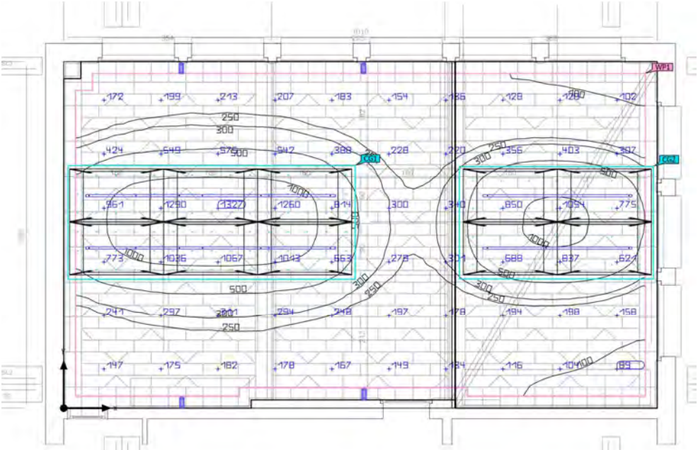
Nivell d'il·luminació mitjana calculat sobre pla de treball.
