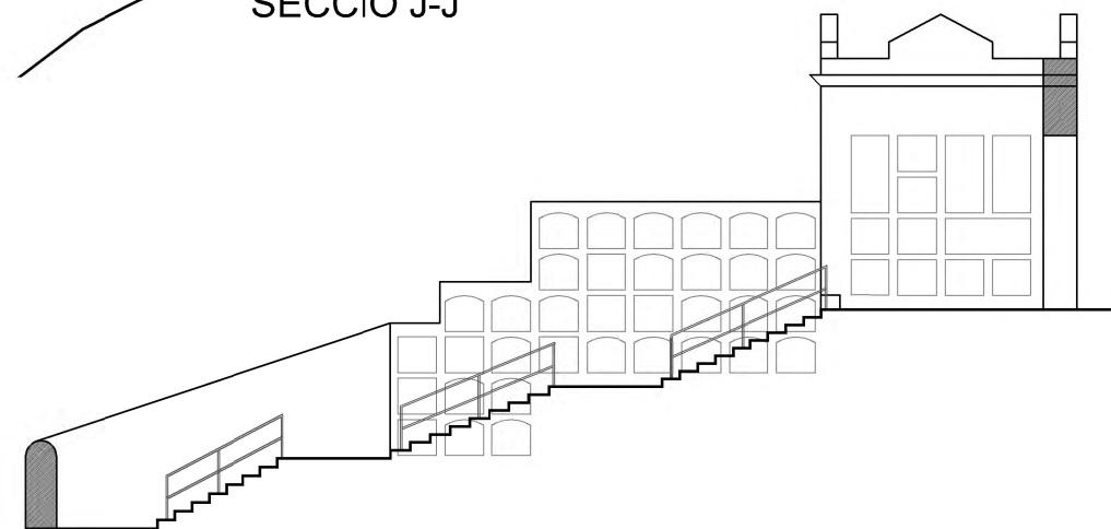
ALÇAT K-K'
