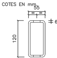
SUPORT TUBULAR DE 120x55mm S/E
