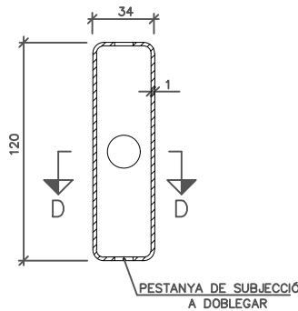
SECCIÓ D-D
