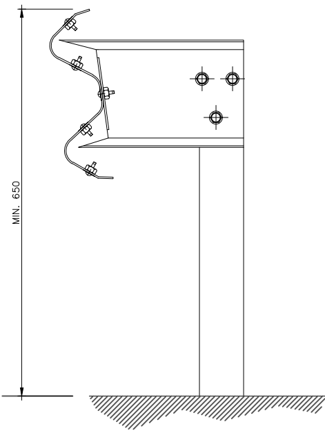
SECCIÓ METAL·LICA SIMPLE AMB DUES TANQUES SIMPLES S/E
