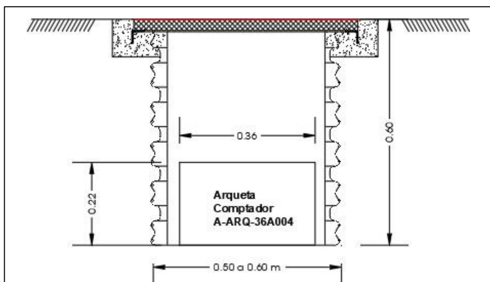
Arqueta exterior per protecció antigela de l'arqueta del comptador.
