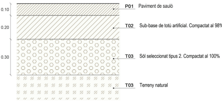
Detall Paviment de sauló
