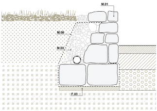
Detall mur de pedra seca / 1 cara vista
