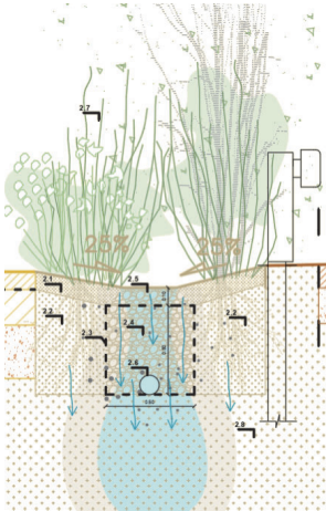
SECCIÓ DETALL 2. CUNETA VERDA
