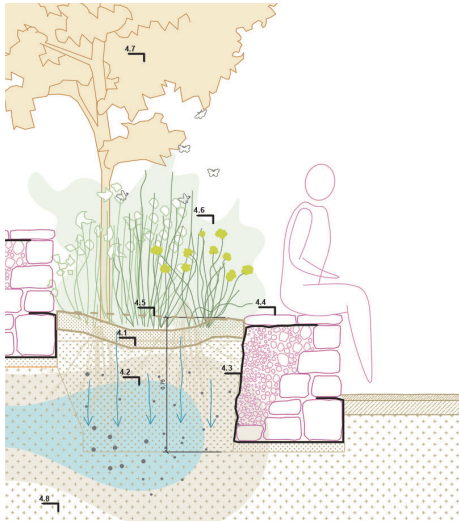
SECCIÓ DETALL 4. BANCALS DE NODE COMPLET
