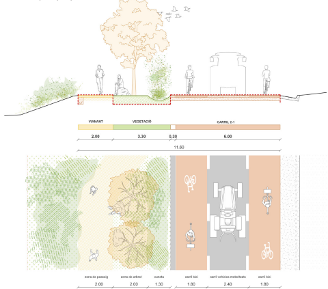
Secció tipus proposta
