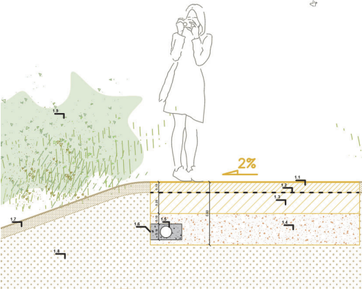
SECCIÓ DETALL 1. CAMÍ DE SAULÓ
