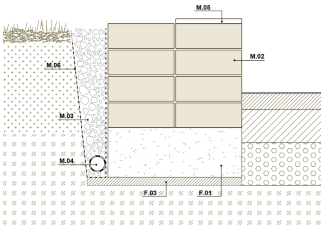
Detall mur de terra compactada
