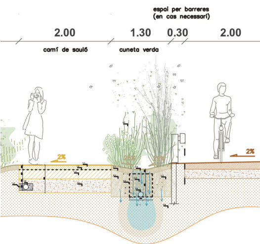
Detall de secció per l'eix 31 amb cuneta d'infiltració vegetada típica del projecte
