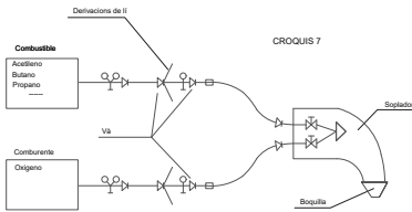
ESQUEMAS DE COMPONENTES DE UNA INSTALACIÓN OXITALLADA
