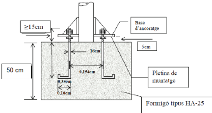
Figura 3: Base per a element de senyalització
