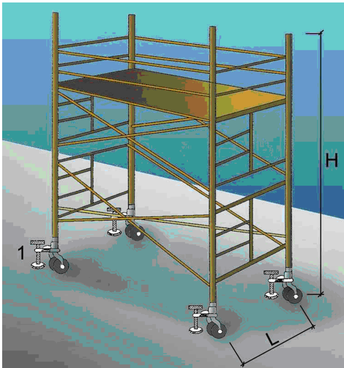
Bastides Metàl·liques Sobre Rodes
