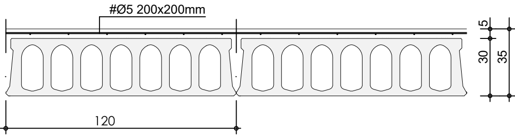
Forjat de plaques pretesades l= 120cm.;
