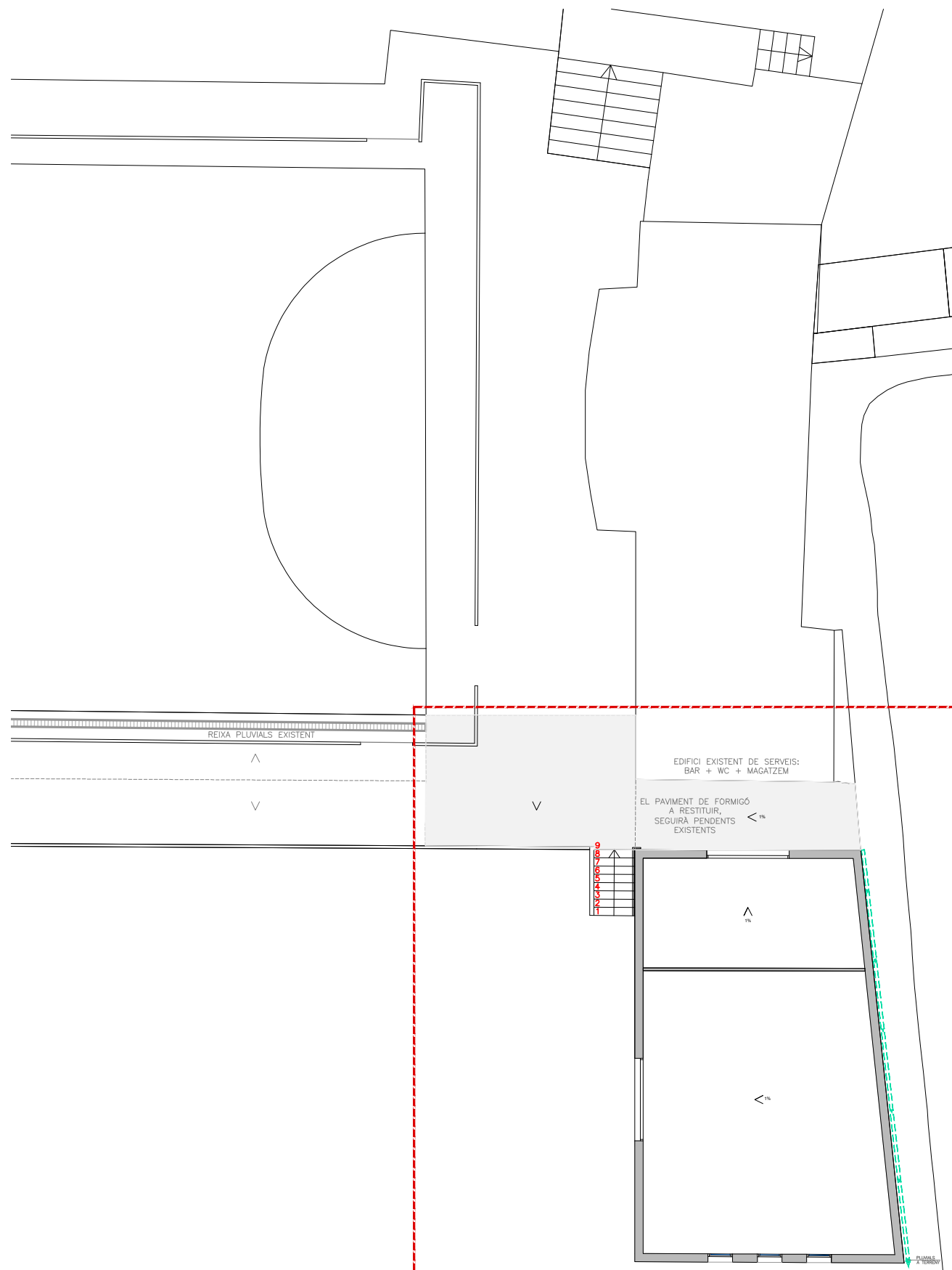
PLANTA URBANITZACIÓ - INSTAL·LACIONS PLUVIALS, e: 1/200
