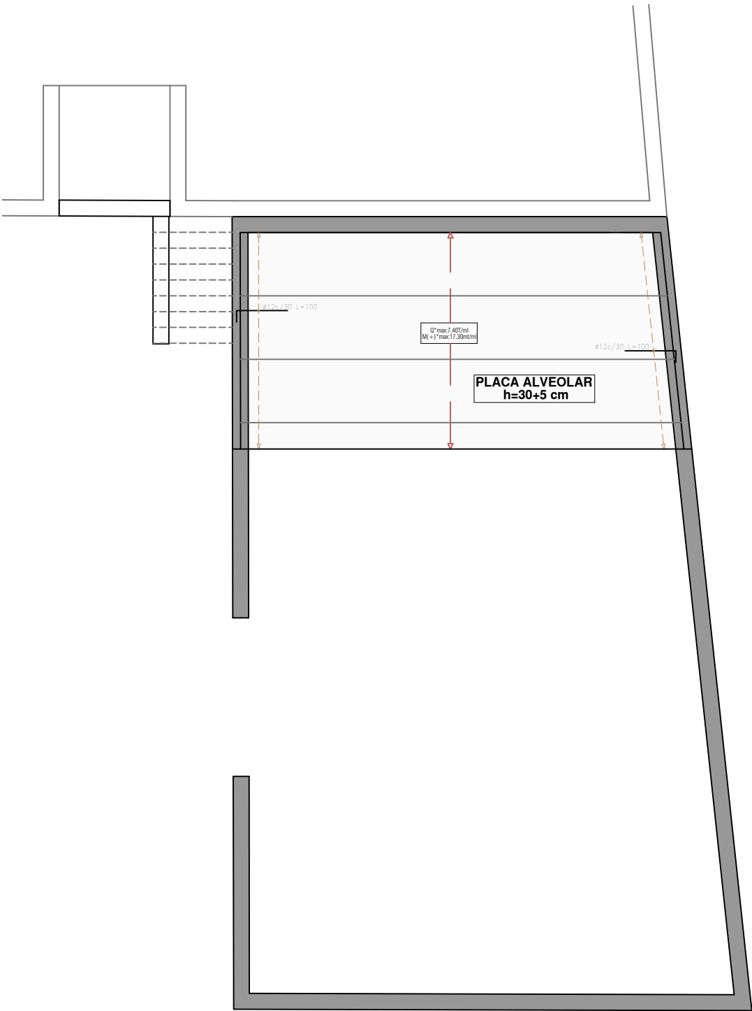
PLANTA FORJAT SANITARI e1/100
