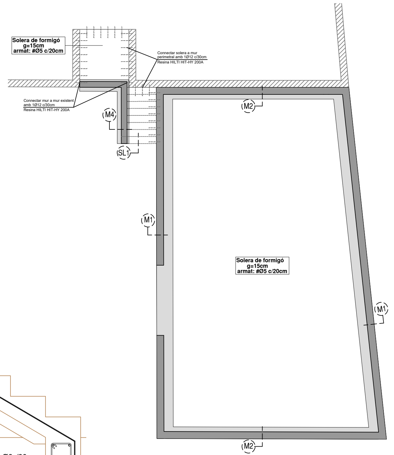
PLANTA FONAMENTS e1/100
