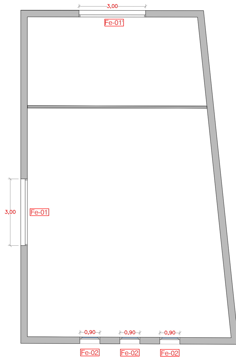
PLANTA UBICACIÓ FUSTERIES MAGATZEM, e:1/100
