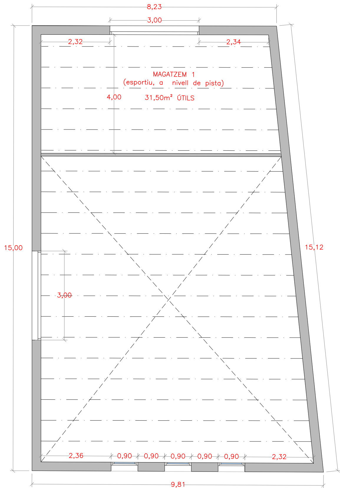
PLANTA NIVELL MAGATZEM 1 (cota+1.41m), e:1/75 (magatzem esportiu, a peu de pista esportiva)
