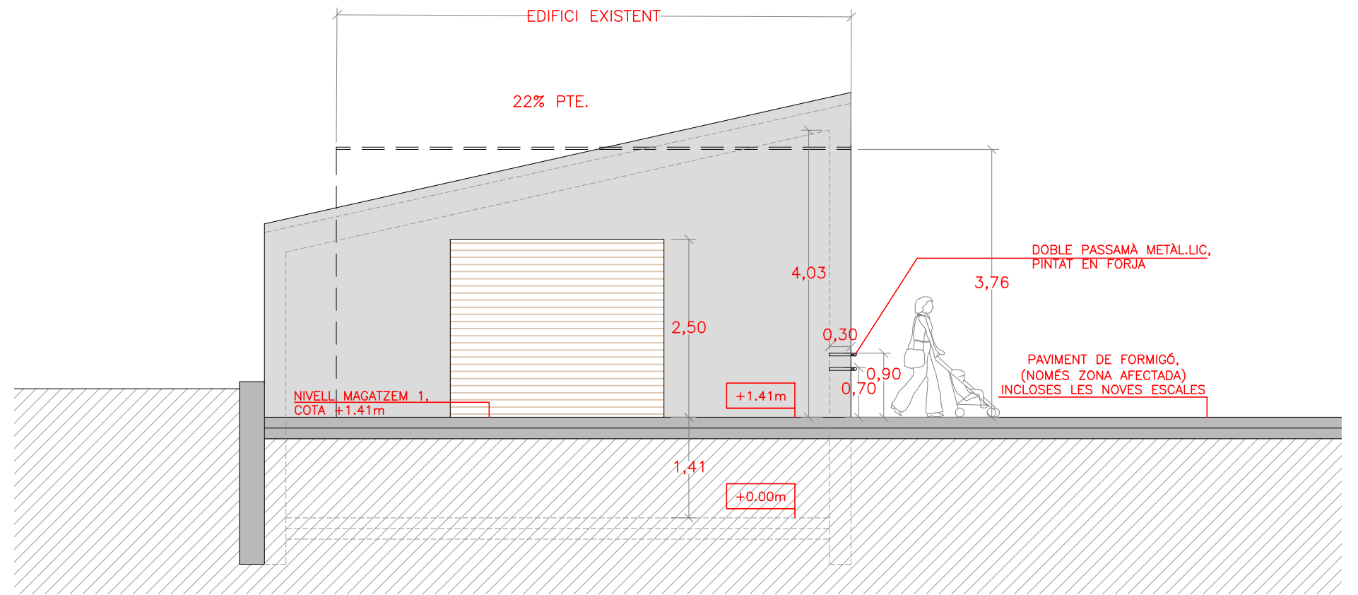
ALÇAT NORD-EST, e:1/75
