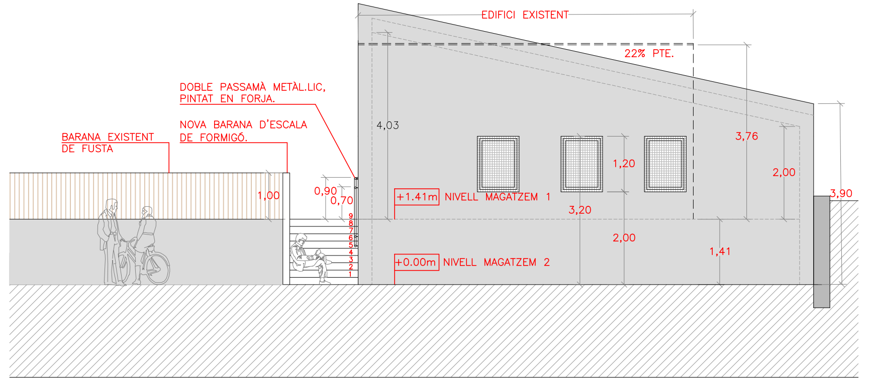
ALÇAT SUD-OEST, e:1/75
