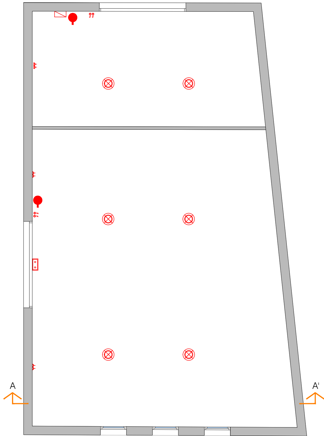
PLANTA INSTAL·LACIÓ ELÈCTRICA, e:1/75
