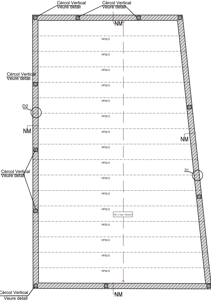
PLANTA COBERTA
