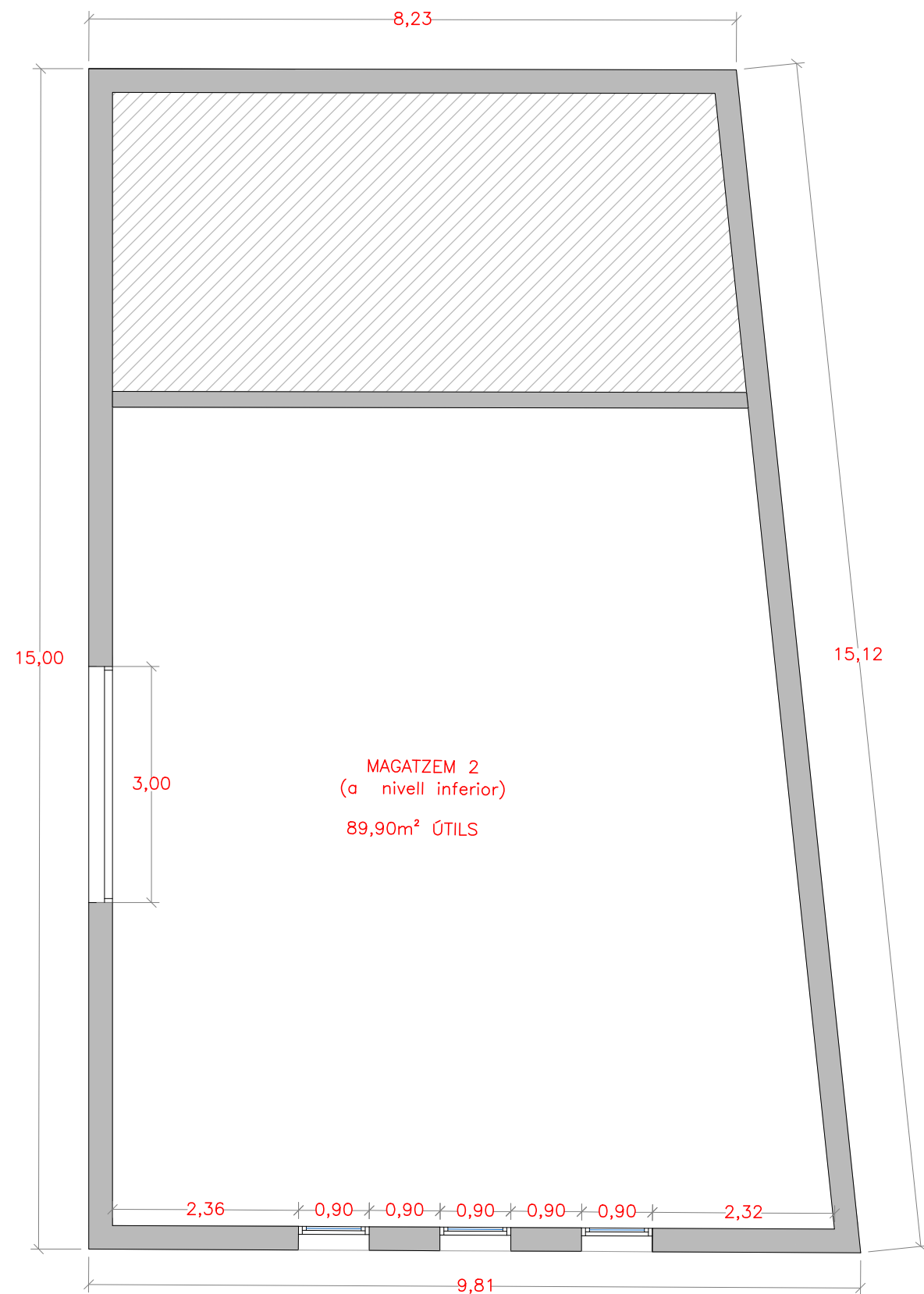
PLANTA NIVELL MAGATZEM 2 (cota+0.00m), e:1/75
