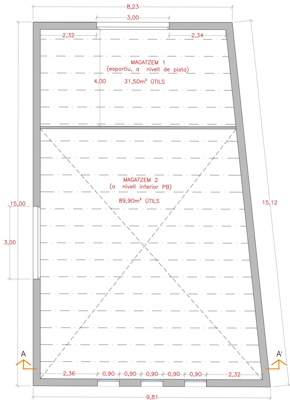
PLANTA MAGATZEM, e:1/75
