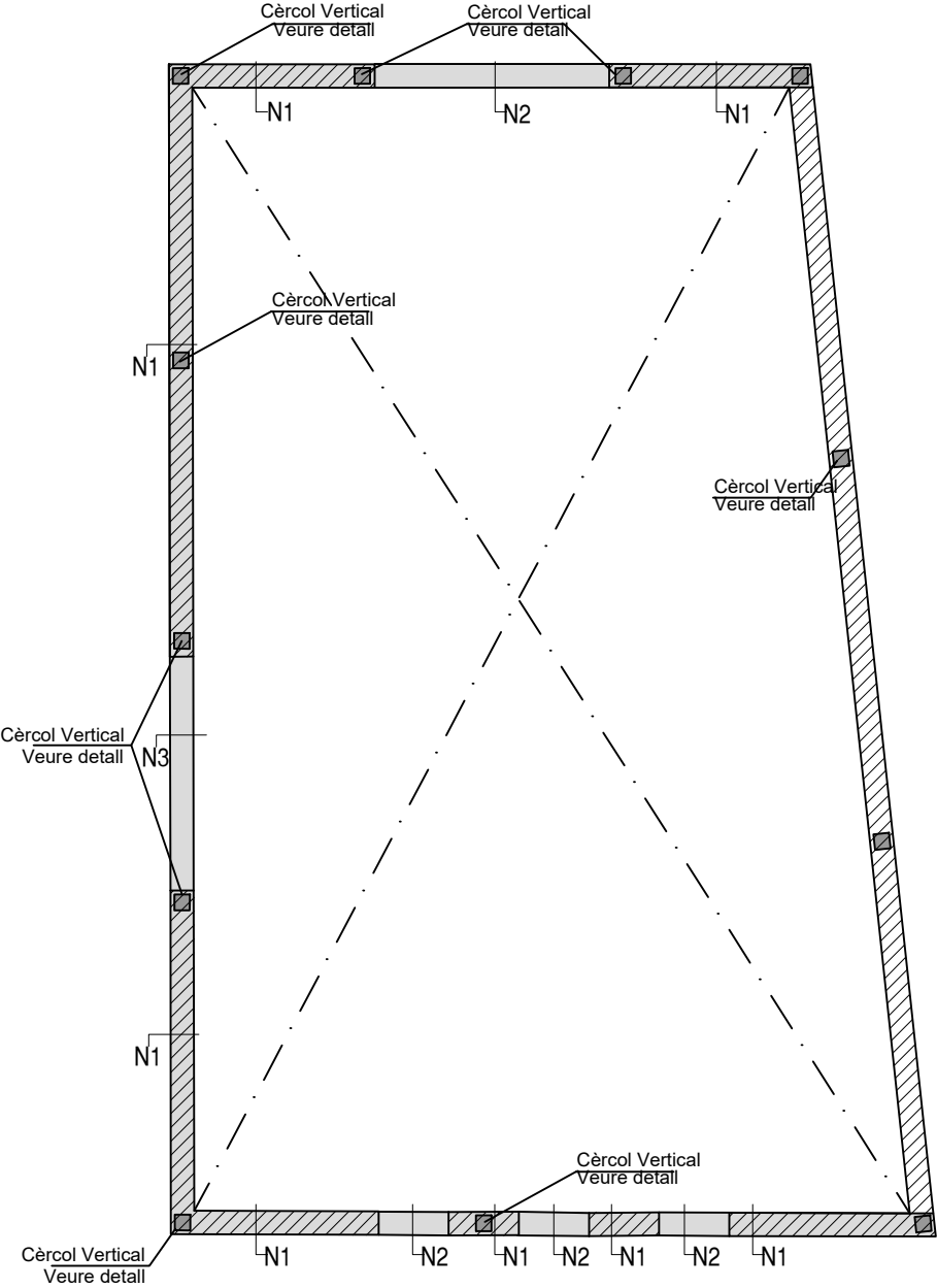
PLANTA NIVELL LLINDES
