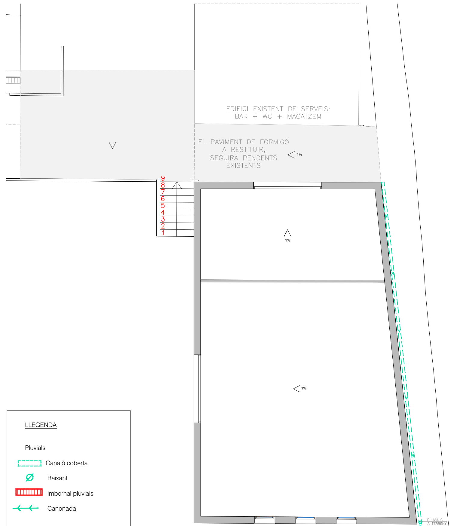
PLANTA MAGATZEM, INSTAL·LACIONS PLUVIALS - e:1/100 (NO ES PREVEU INSTAL·LACIÓ D'AIGUA NI SANEJAMENT)
