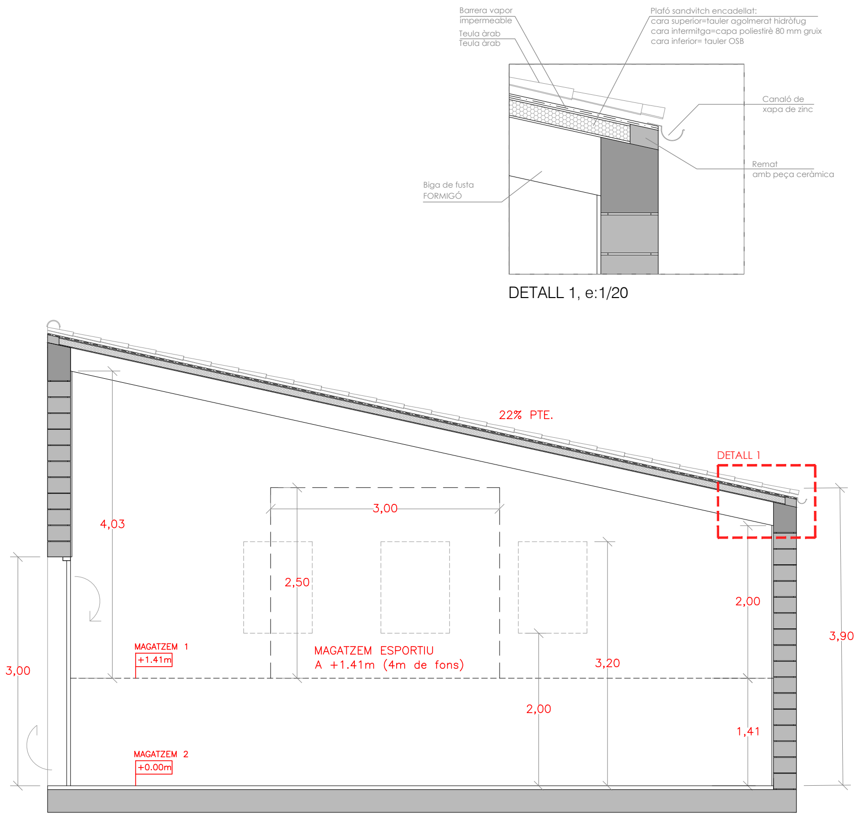
SECCIÓ CONSTRUCTIVA A-A', e:1/50
