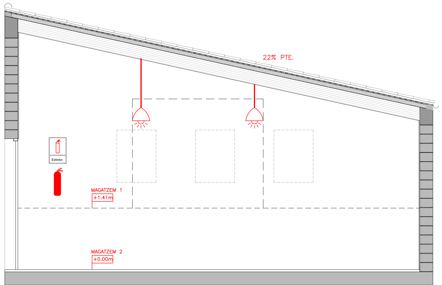
SECCIÓ A-A', e:1/50
