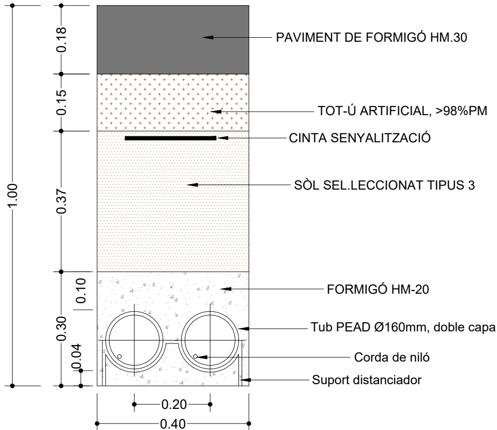
SECCIÓ TIPUS PER 2 CANONADES (2TF) EN CALÇADA
