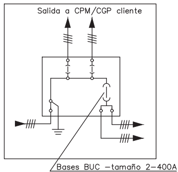
ESQUEMA UNIFILAR CAJA DE DISTRIBUCIÓN URBANA
