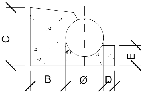
SECCIÓ
