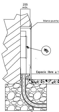
ESQUEMA CAJA SECCIONAMIENTO CON ACOMETIDA PARTE INFERIOR
