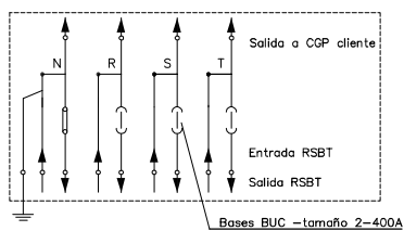
ESQUEMA CAJA SECCIONAMIENTO CON ACOMETIDA PARTE SUPERIOR
