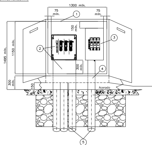
MONTAJE HORIZONTAL
