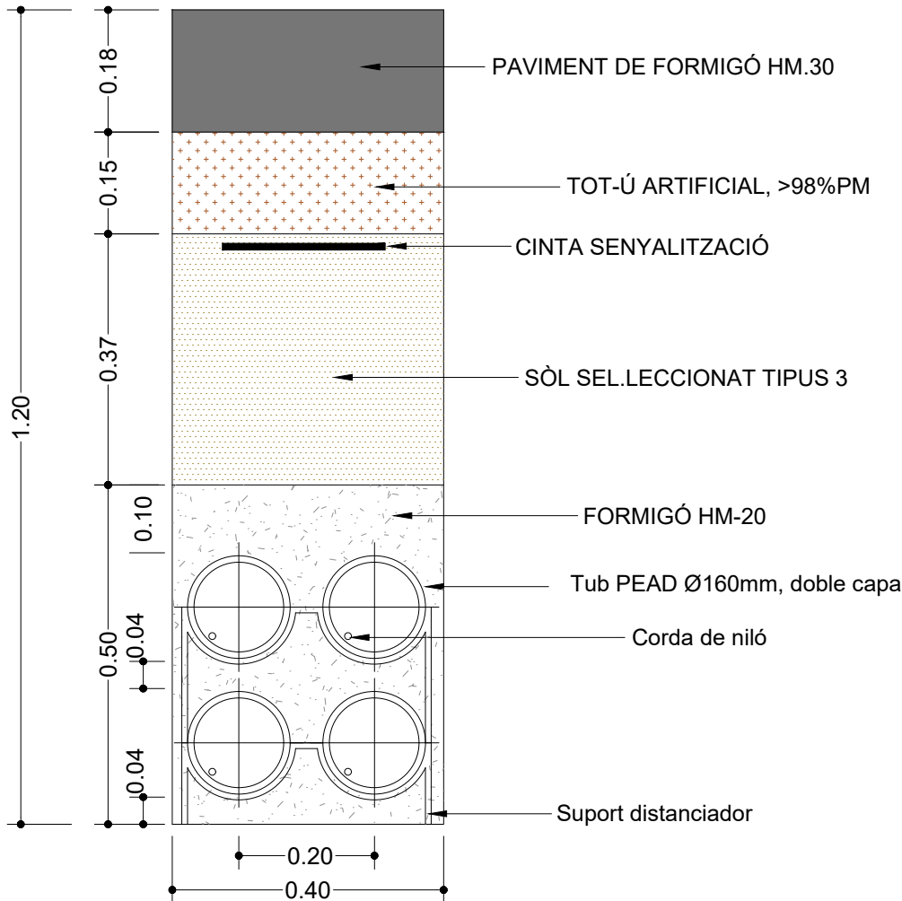
SECCIÓ TIPUS PER 4 CANONADES (4TF) EN CALÇADA
