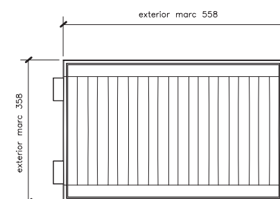
TAPA EMBORNAL B-22BD FUNDICIO DUCTIL
