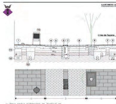
DETALL ESCOBELL PAVIMENTS
