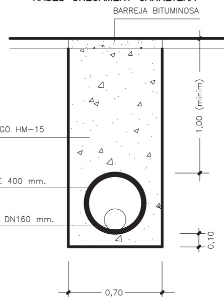
RASES CREUAMENT CARRETERA
