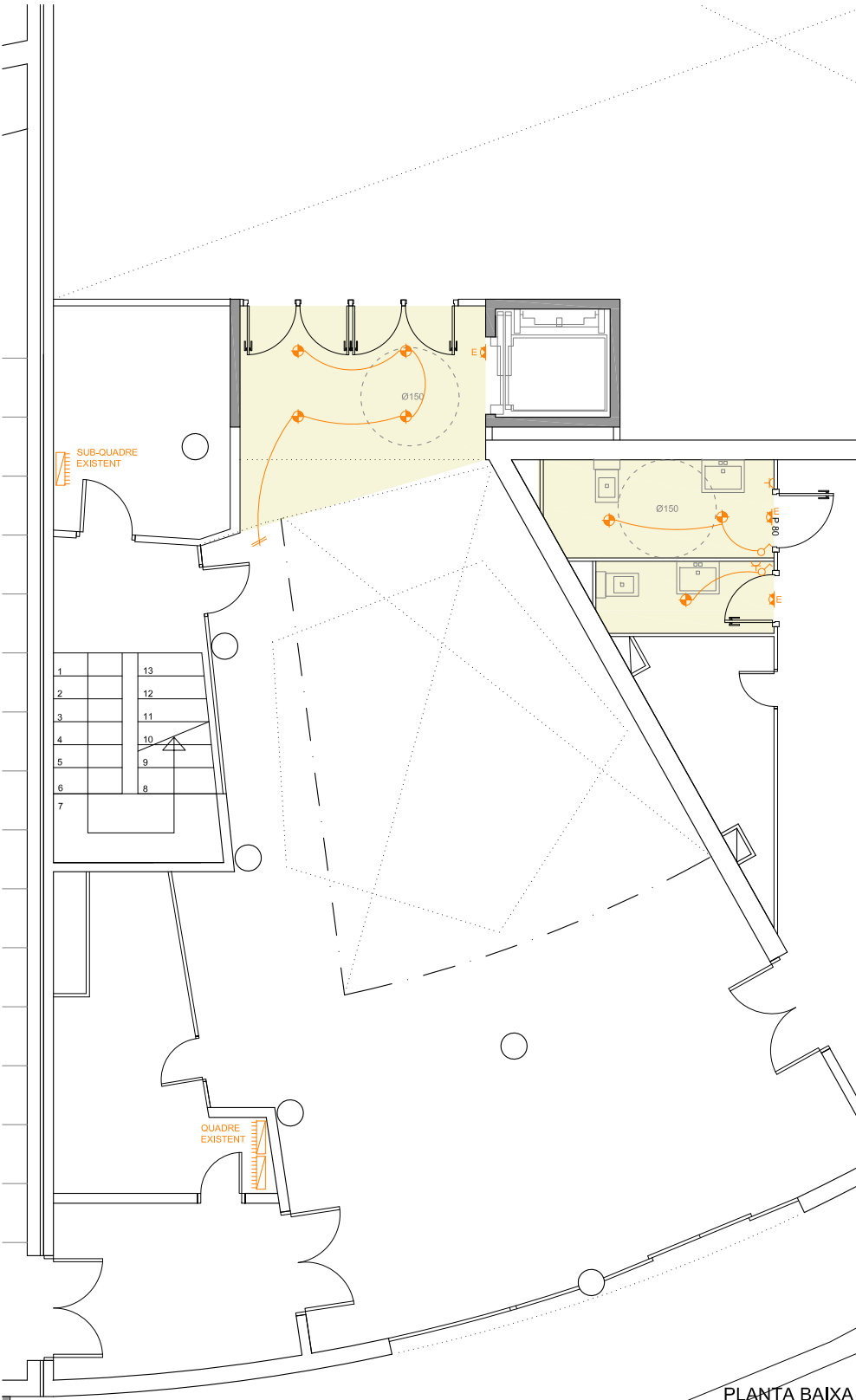
PLANTA BAIXA
