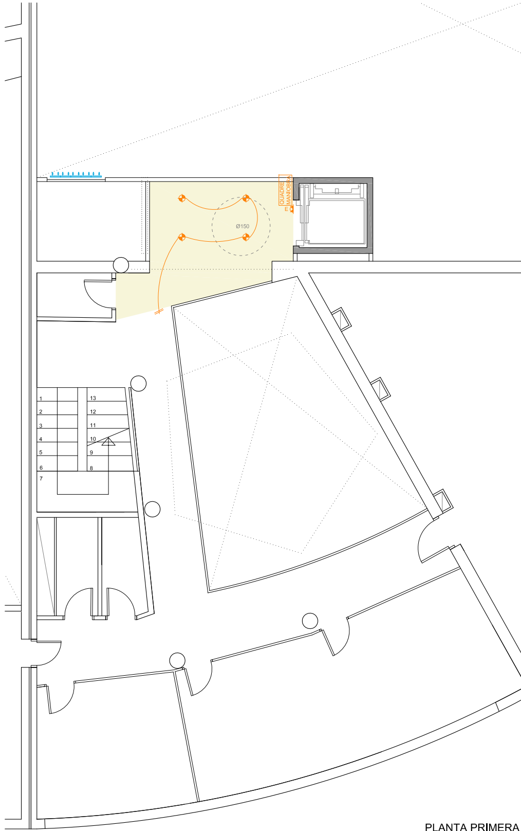
PLANTA PRIMERA
