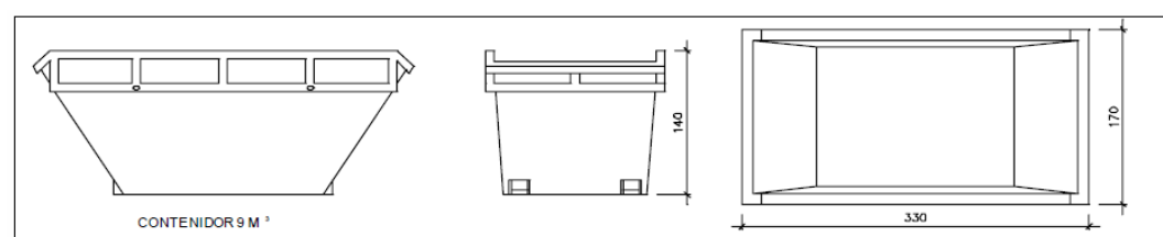
Figura 4 Contenidor de residus inerts.
