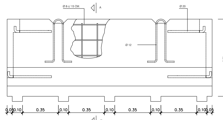
SECCIÓ A-A
