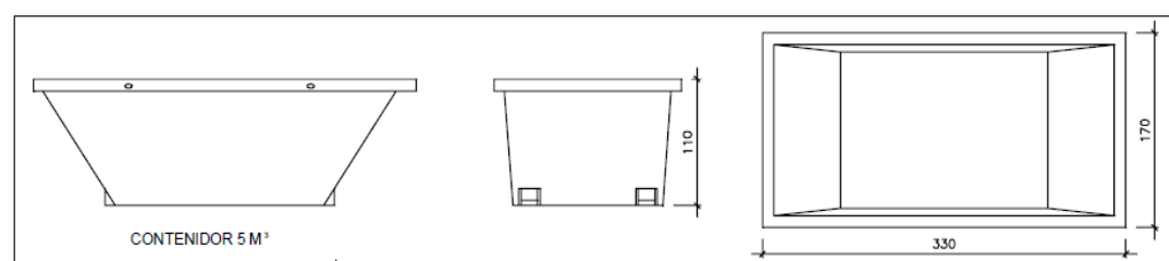
Figura 5 Contenidor de residus no especials.
