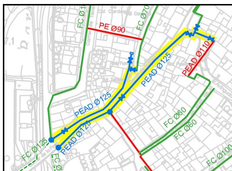
Actuació 6 proposada en la xarxa en baixa al centre del municipi
