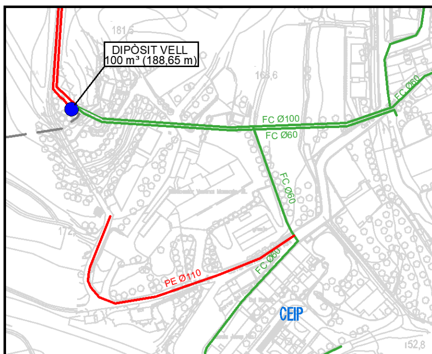
Estat actual de la xarxa en baixa a la zona propera al Dipòsit Vell
