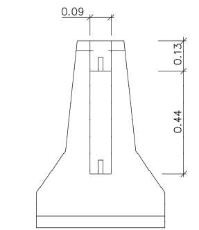
ALÇAT TRANSVERSAL
