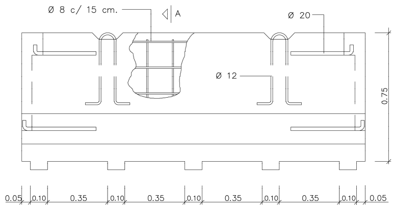
SECCIÓ A-A'
