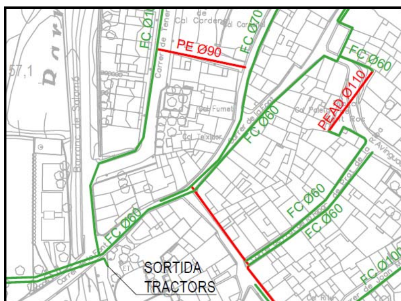
Estat actual de la xarxa en baixa al centre del municipi
