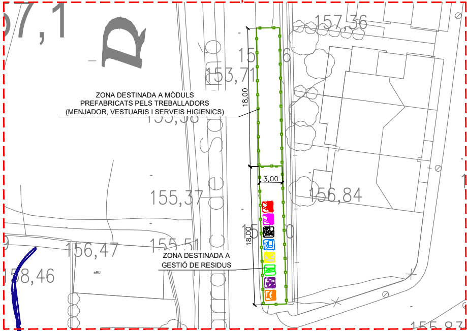
SITUACIÓ DE CASETES D'OBRA E:1/500
