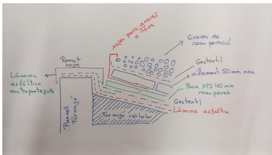
Detall secció constructiva
