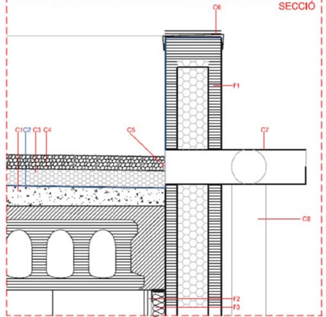
DETALL A. BAIXANTS-SOBREIXIDORS
