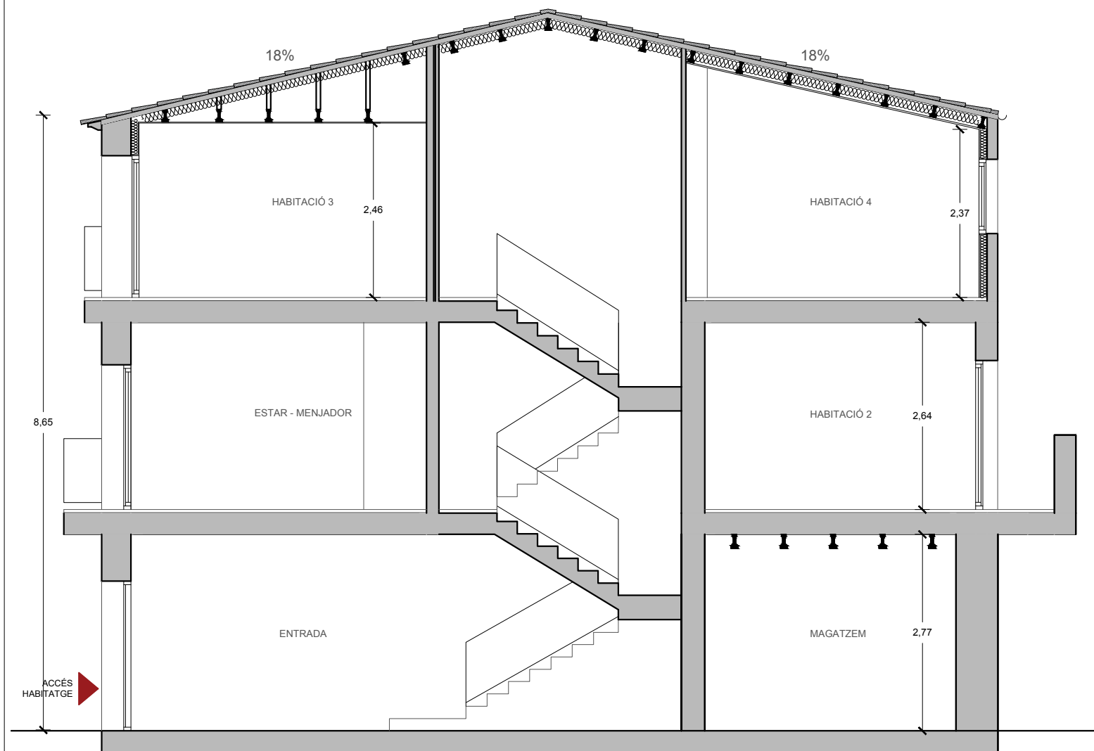
Proposta - secció E 1:75
