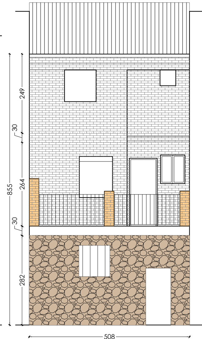
Estat actual - A2 pati E 1:75
