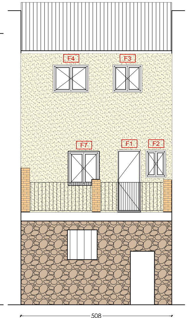
Proposta - alçat pati E 1:75
