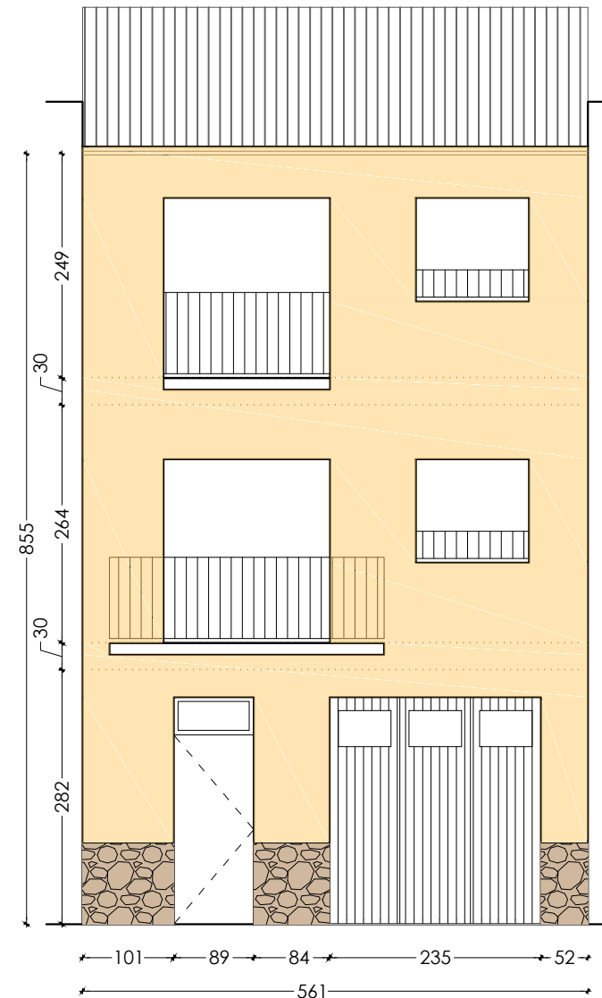
Estat actual - A1 carrer Bassa E 1:75
