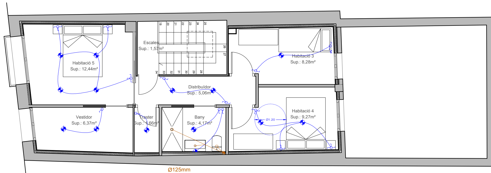
Instal·lació elèctrica i sanejament planta sota coberta E 1:75
