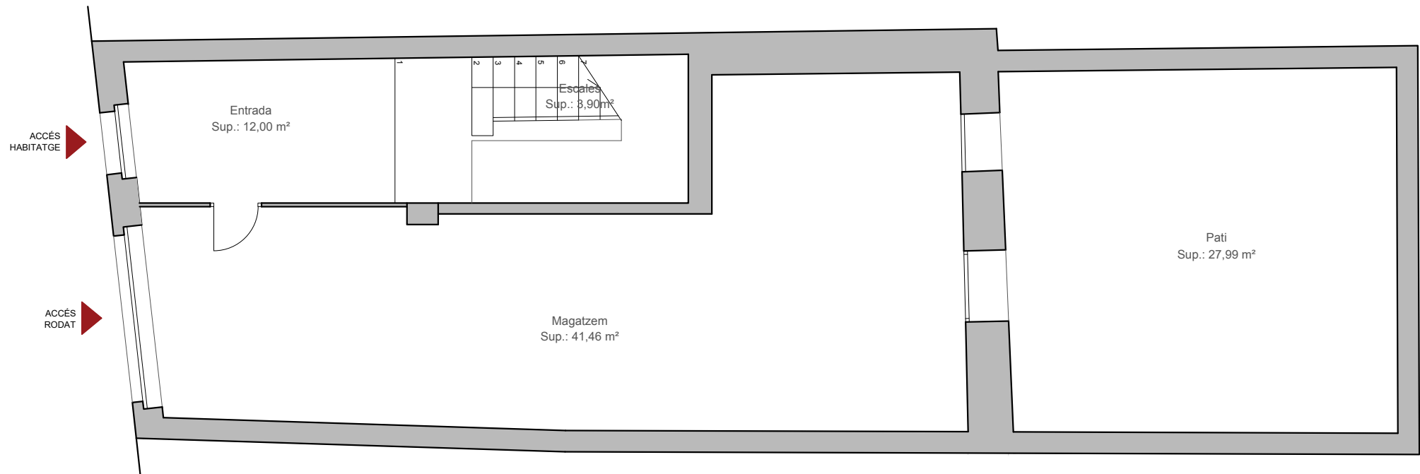
Estat actual planta baixa
