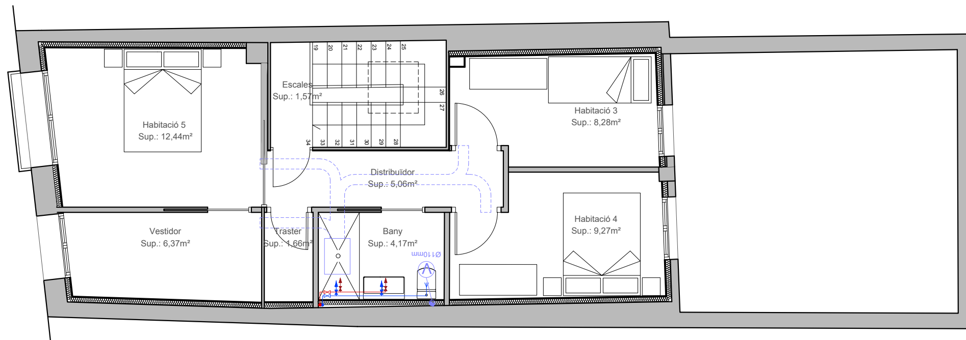
Instal·lació aigua sanitària i ventil·lació planta sota coberta E 1:75
