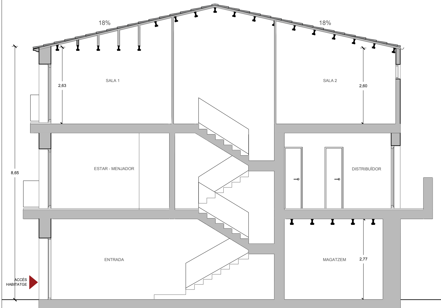
Estat actual - secció E 1:75
