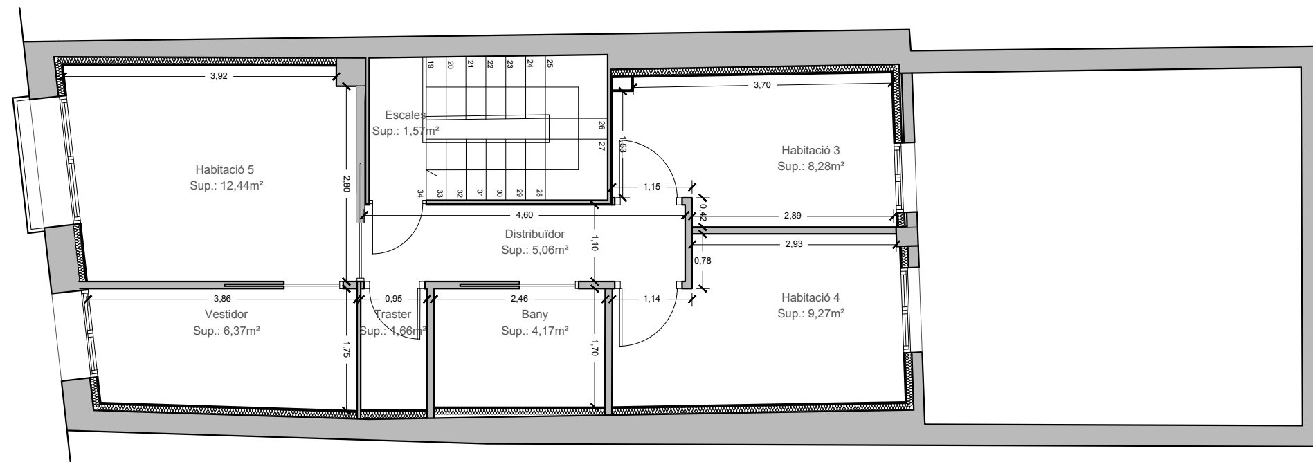
Replanteig proposta planta sota coberta E 1:75
