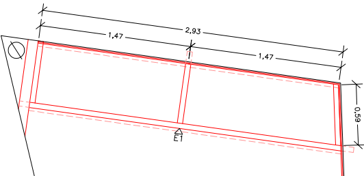
PLANTA SUBSTRUCTURA METÀL·LICA SUPORT TAULELL
