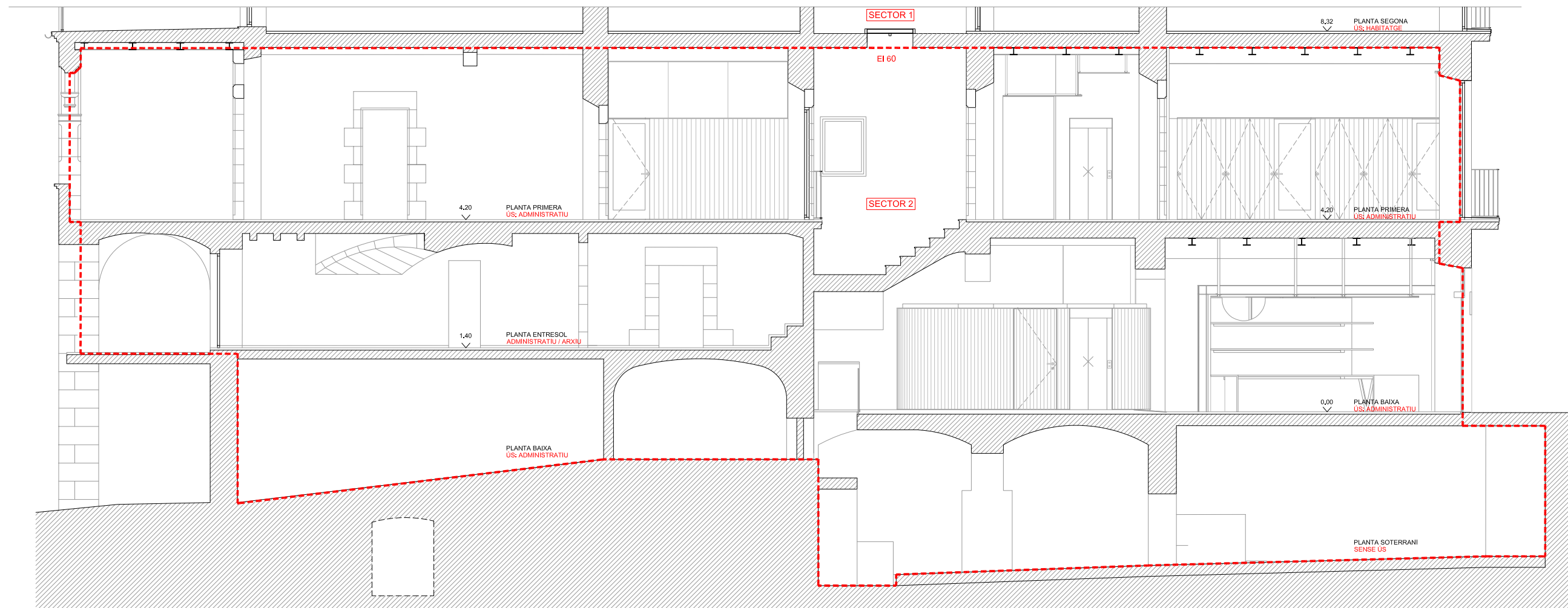
SECCIÓ GENERAL A-A'
