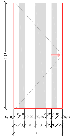
ALÇAT SALA DE TREBALL
