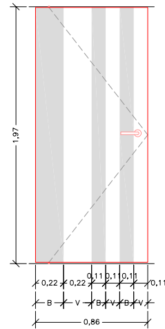
ALÇAT DESPATX 1
