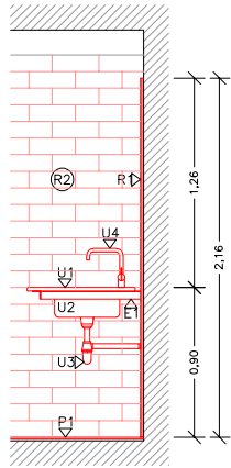
SECCIÓ C-C'
