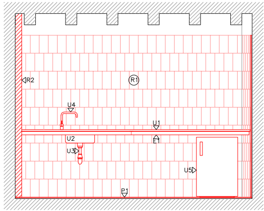
SECCIÓ A-A'
