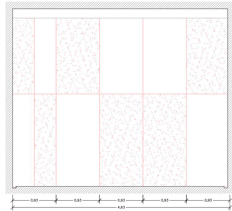
SECCIÓ B-B'
