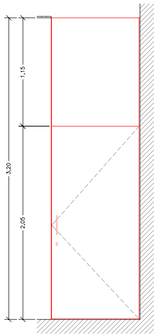
ALÇAT
