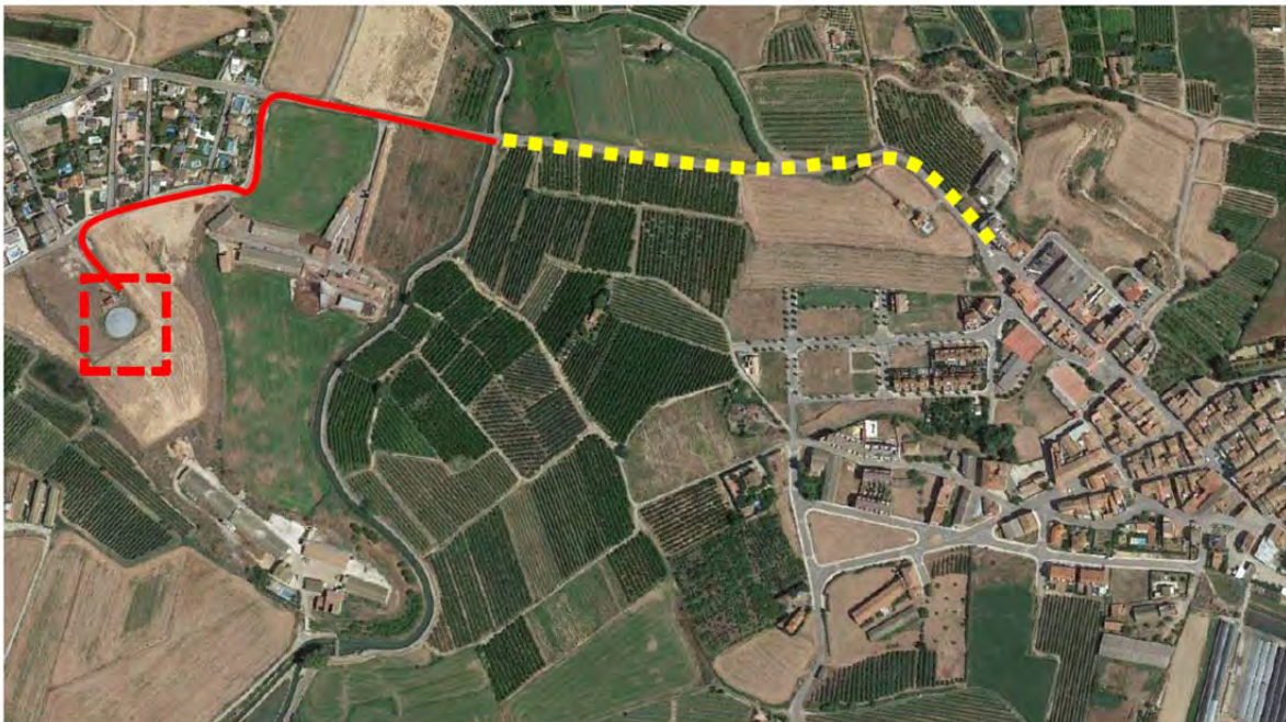
En vermell tram de canonada en polietilè, en groc tram de canonada a substituir (actualment de fibrociment DN250)
