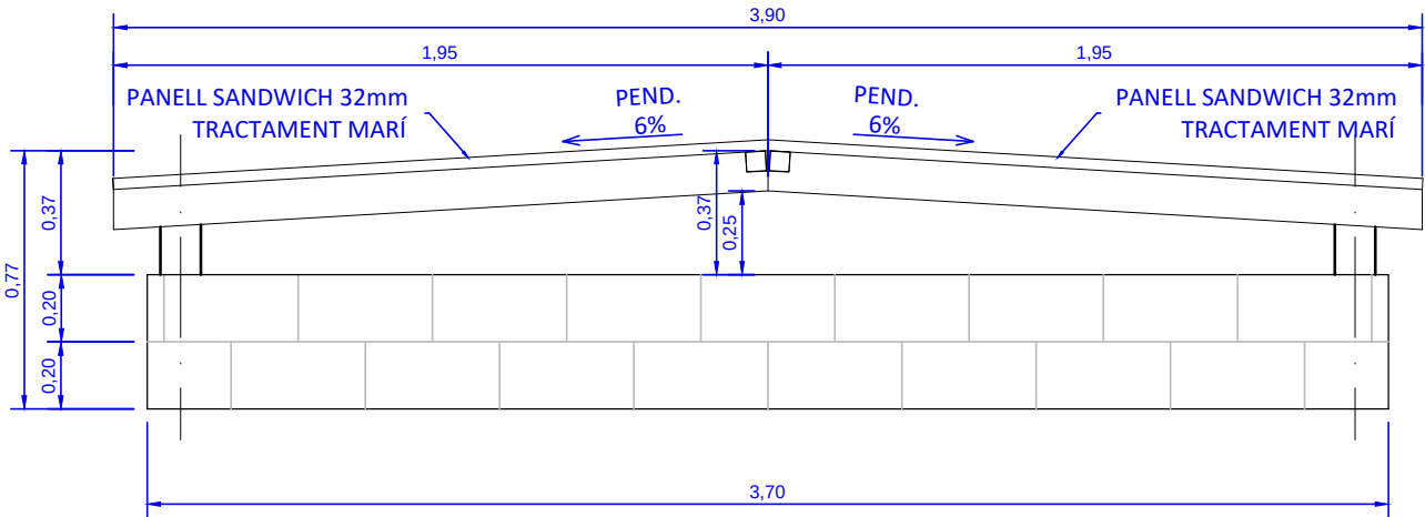
COBERTA ALÇAT ESC. 1/25
