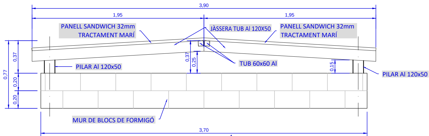
ESTRUCTURA SECCIÓ TRANSVERSAL ESC. 1/25
