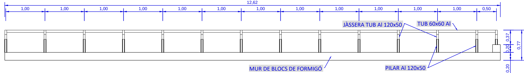
ESTRUCTURA SECCIÓ LONGITUDINAL ESC. 1/50
