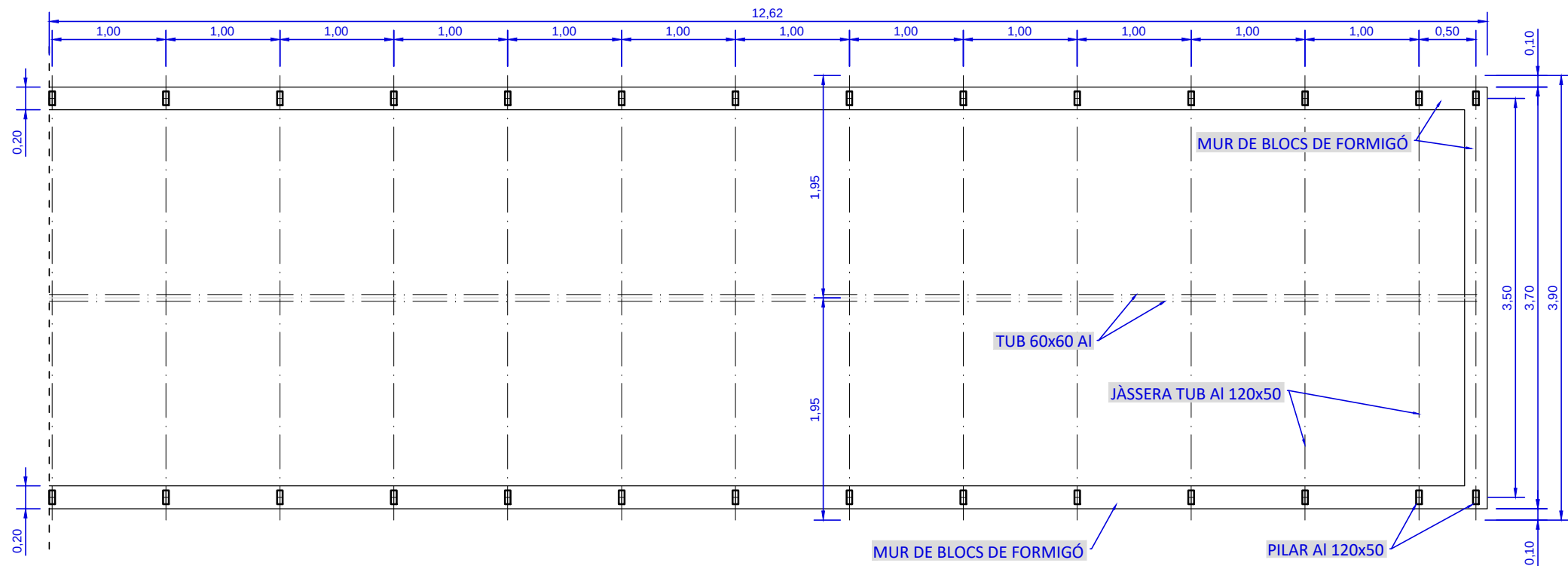
ESTRUCTURA PLANTA Esc. 1/50
