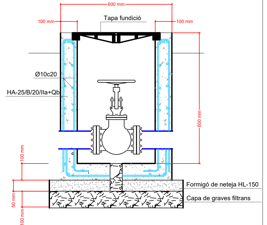
SECCIÓ A-A
