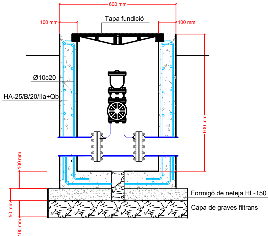
SECCIÓ A-A'
