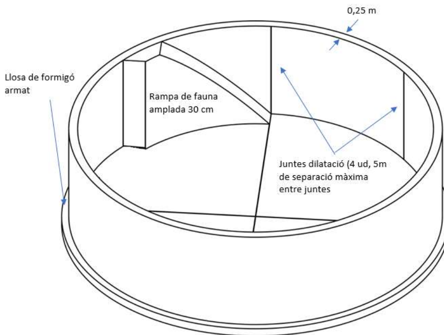
Imatge 22: Esquema del nou punt d'aigua proposat
