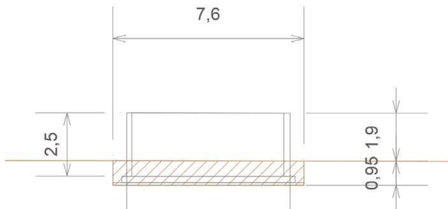
Imatge 23: Esquema dels moviments de terra.
