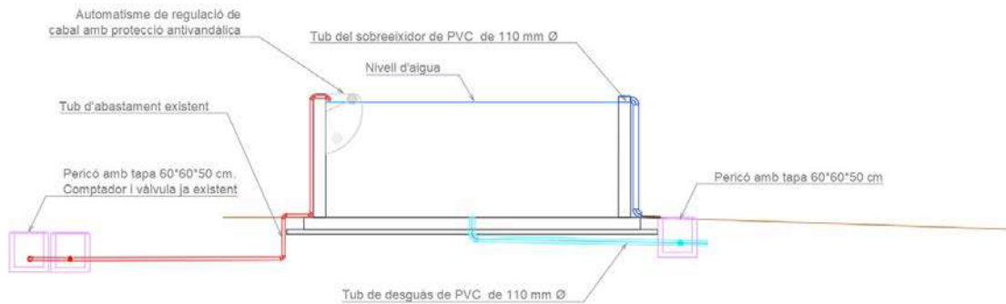
Imatge 32: Elements hidràulics dels punts d'aigua.
