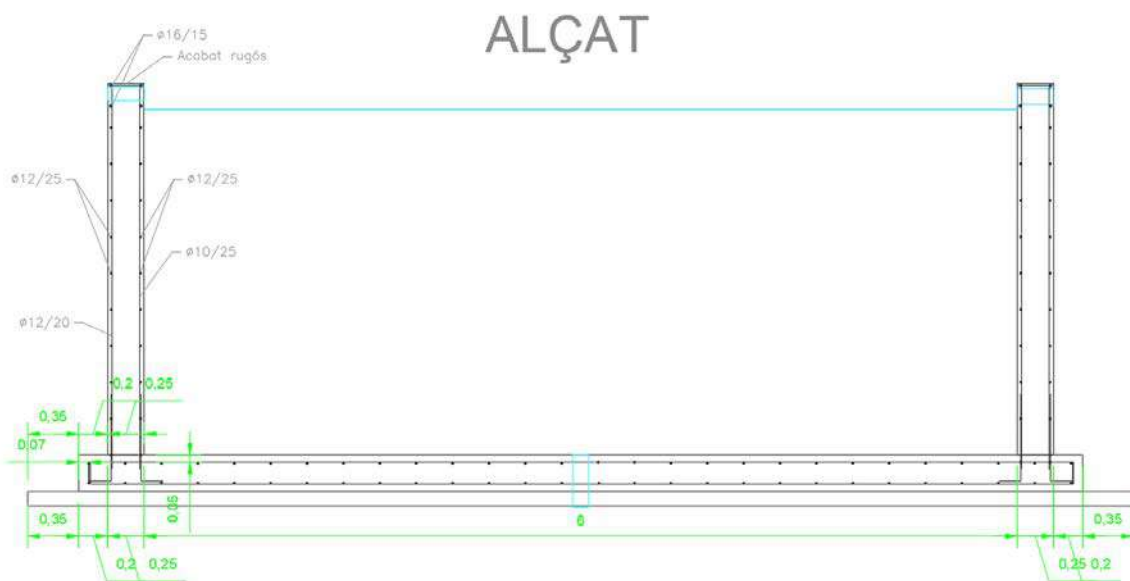
Imatge 27: Esquema de l'armat de les parets del punt d'aigua.
