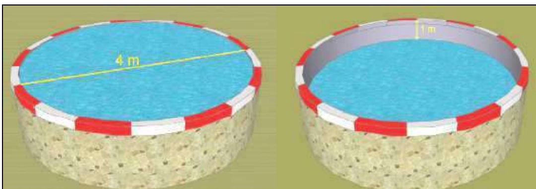
Imatge 21: Dimensió mínima de la làmina d'aigua i requeriment mínim de fondària de la làmina d'aigua per a la càrrega de mitjans aeris.
