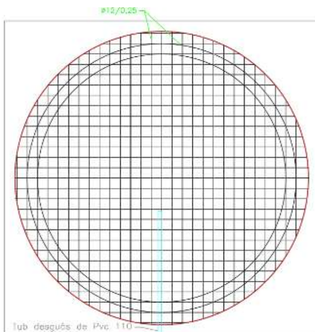
Imatge 25: Esquema de l'armat de la sabata.
