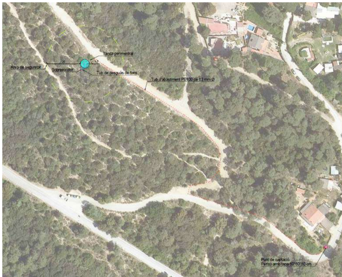
Imatge 34: Localització del punt de captació i l'abastiment proposat pel punt d'aigua del Turó Pelat.
