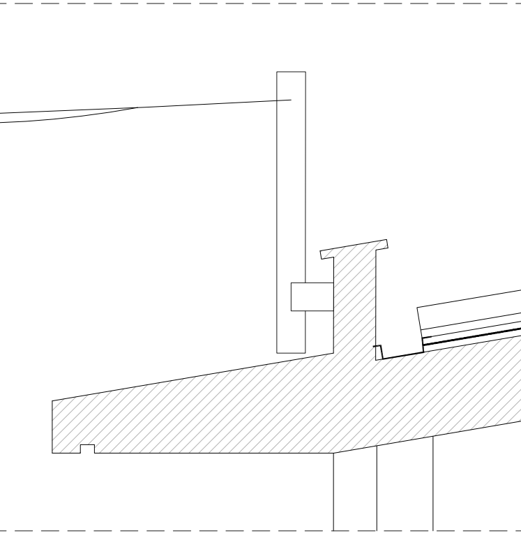
Detall anclatge màstils
