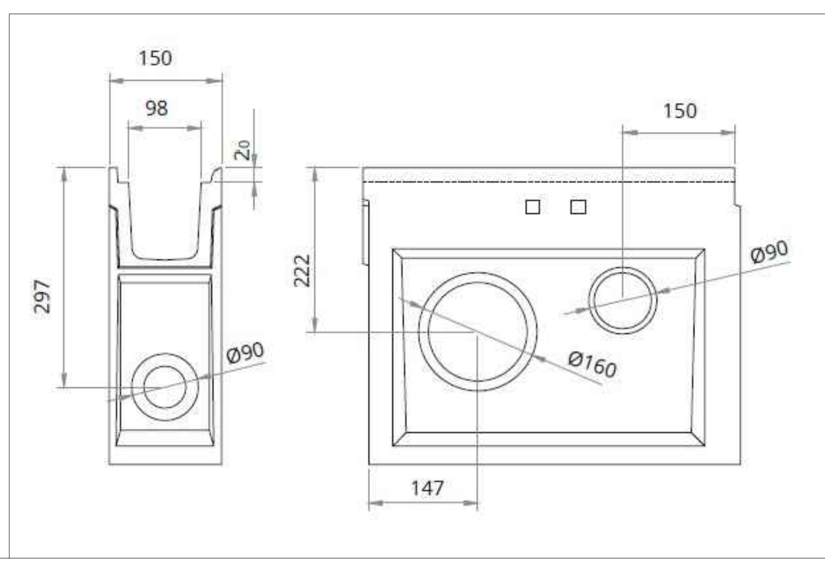
DETALL DE L'ARQUETA ARENERA
