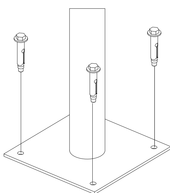
DETALL PERN DE FIXACIÓ
