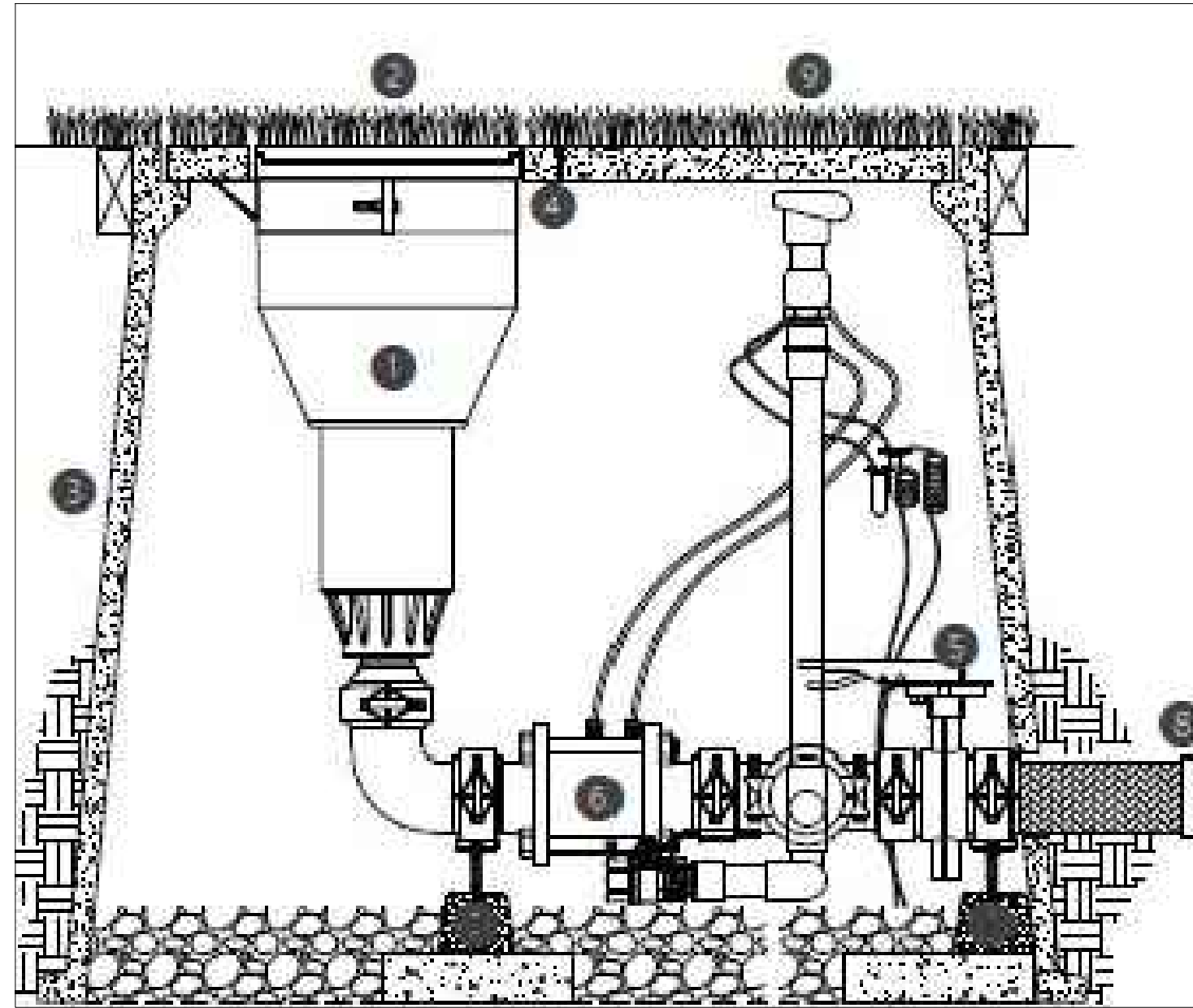
DETALL DE LA CANAL
