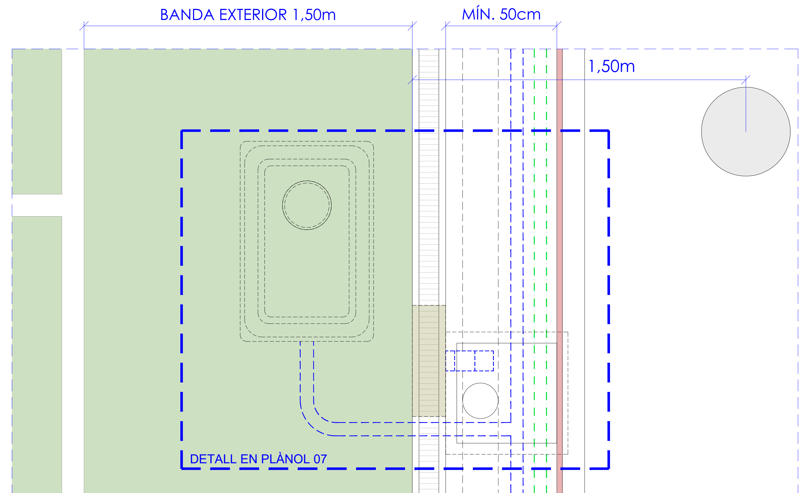
DETALL TROBADA PAVIMENT GESPA EN EXTREM LATERAL DEL CAMP
