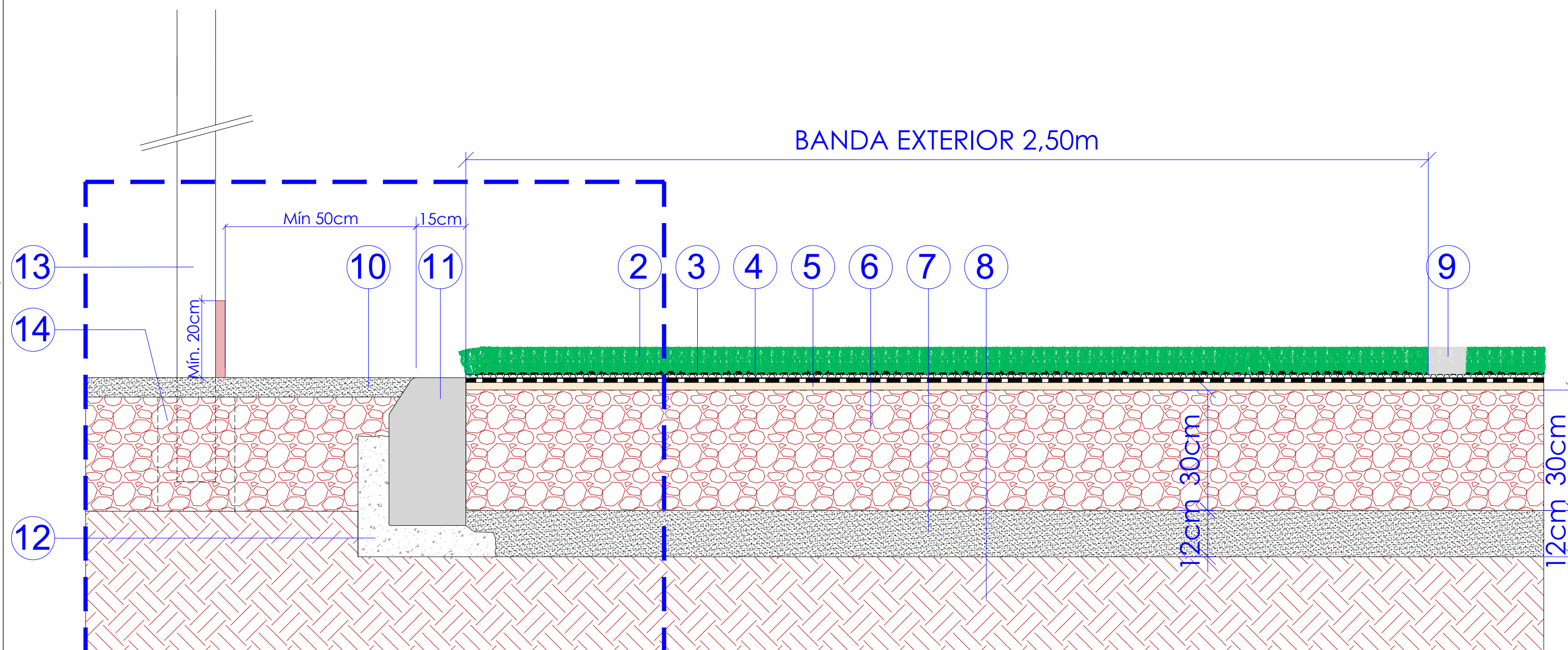
DETALL TROBADA PAVIMENT GESPA EN EXTREM FINAL DEL CAMP
