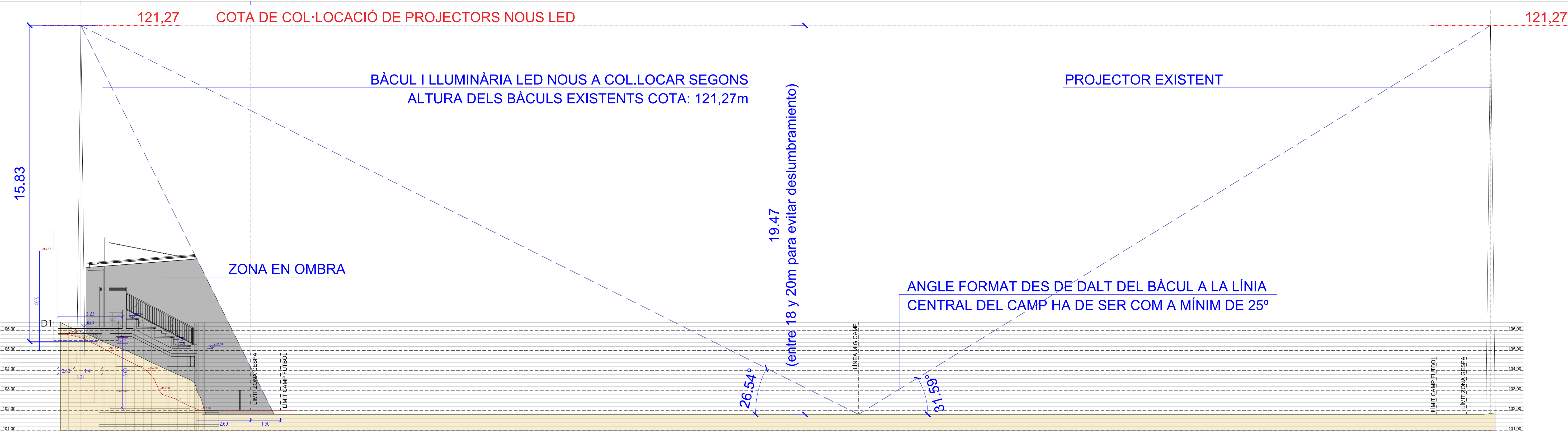
SECCIÓ TRANSVERSAL
