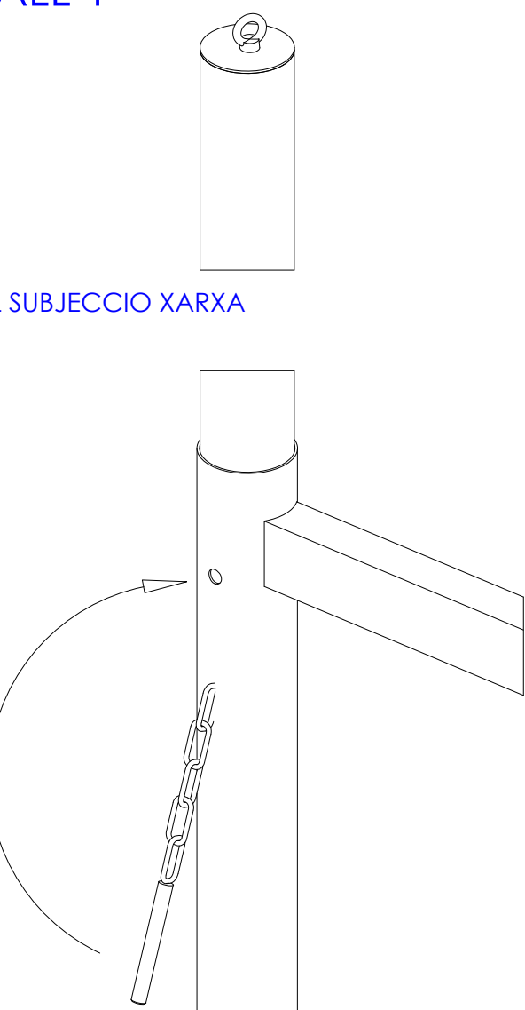
DETALL PERN DE FIXACIÓ
