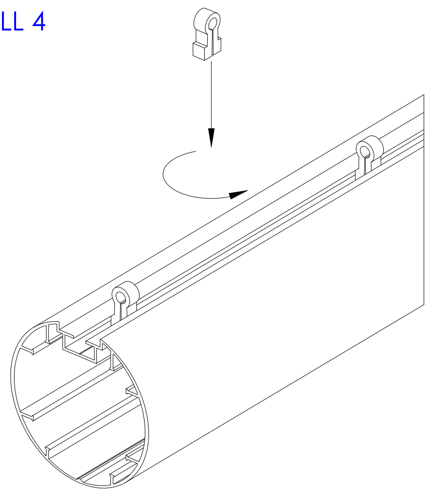
DETALL SUBJECCIÓ DE LA XARXA
