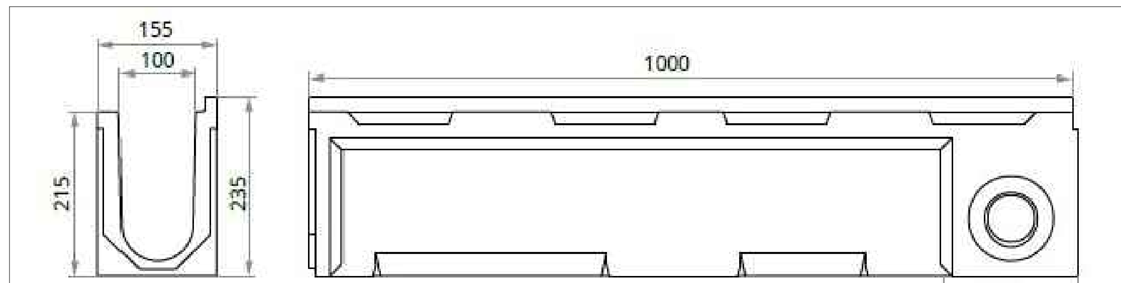
DETALL DE L'ARQUETA ARENERA
