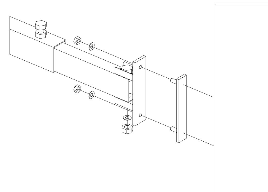
DETALLE UNIÓ PAL AMB ESTRUCTURA D'ABATIMENT
