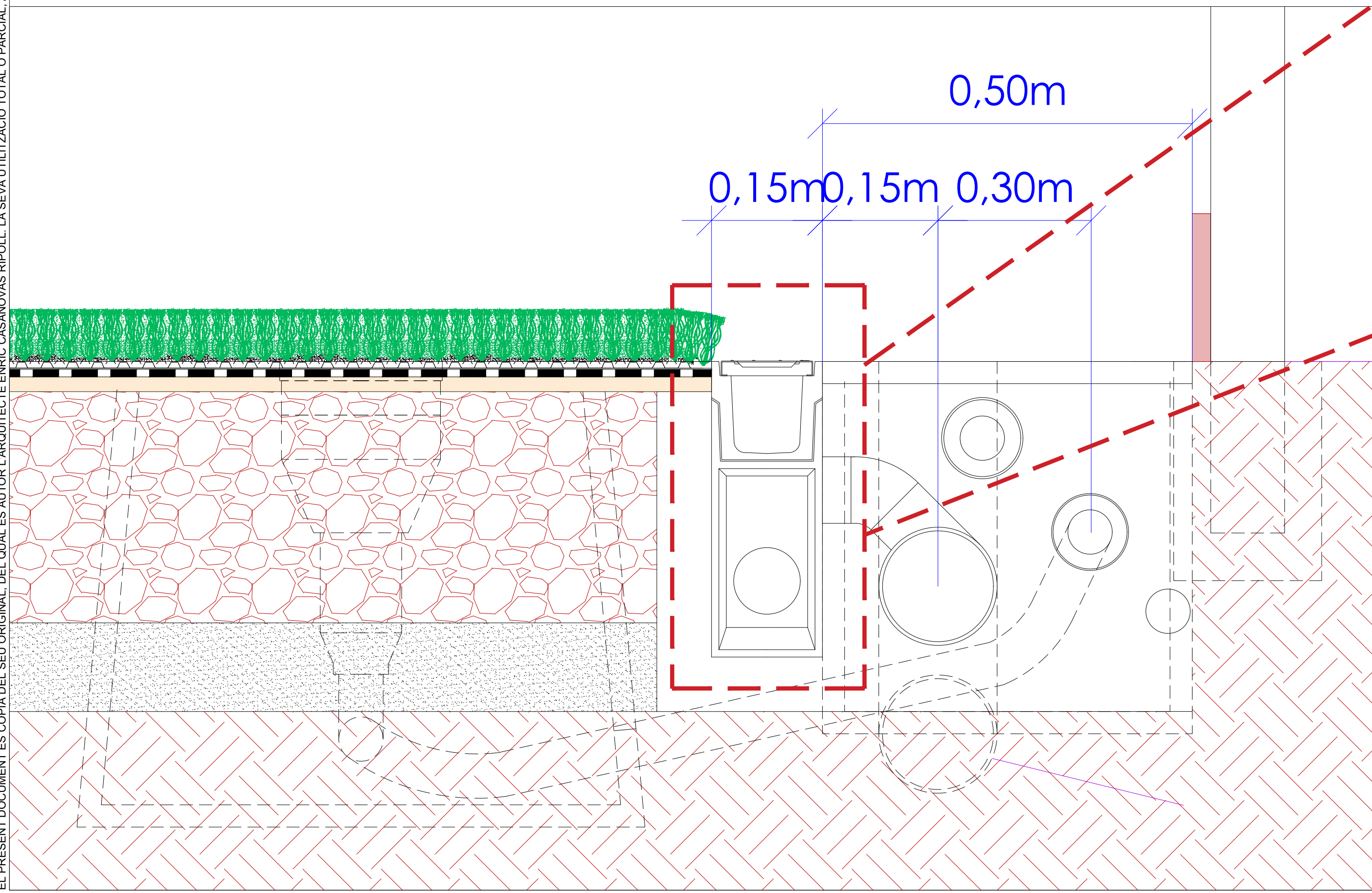
DETALL DE L'ARQUETA ARENERA
