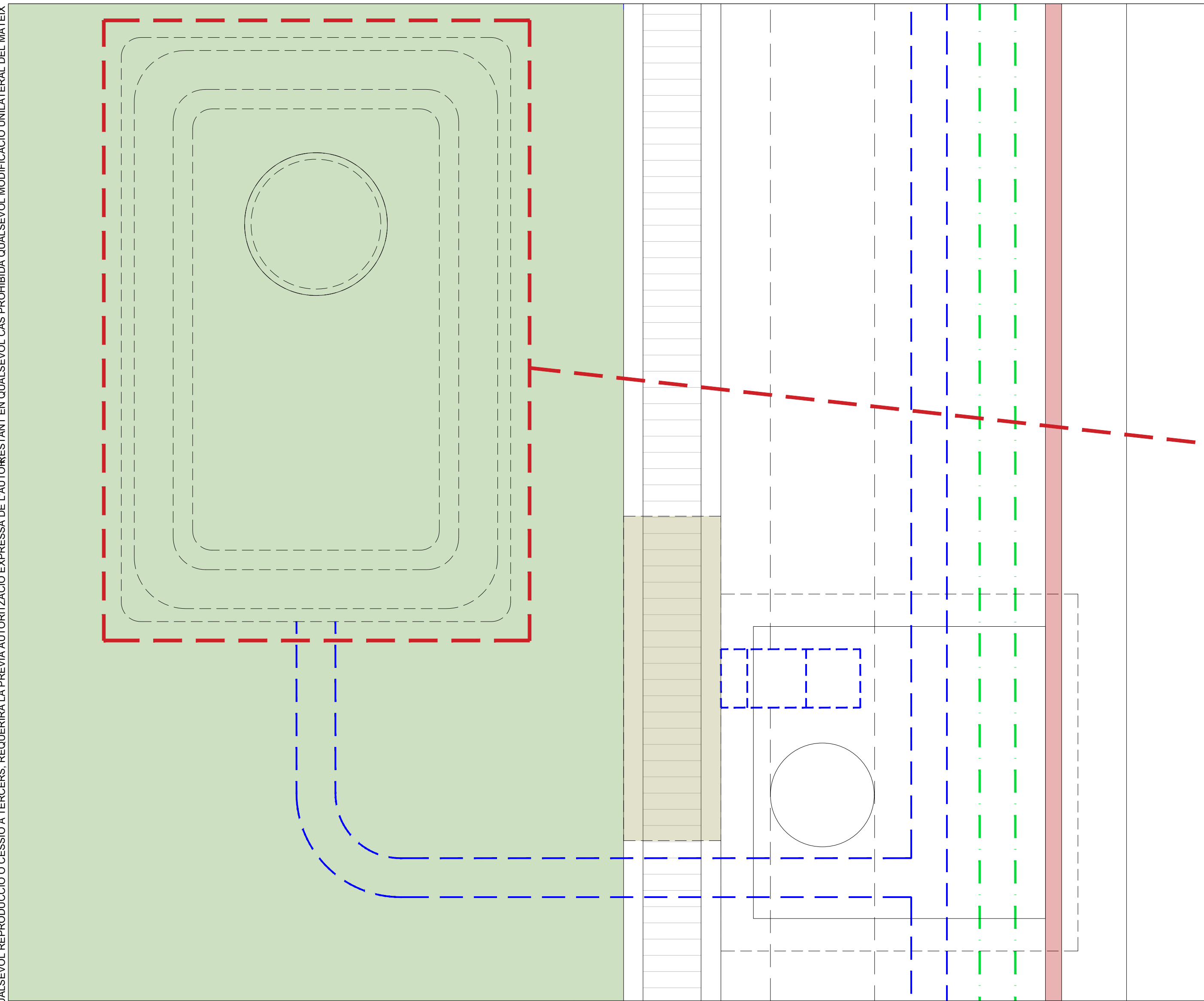
DETALL DE L'ASPIRSOR ACABAT GESPA
