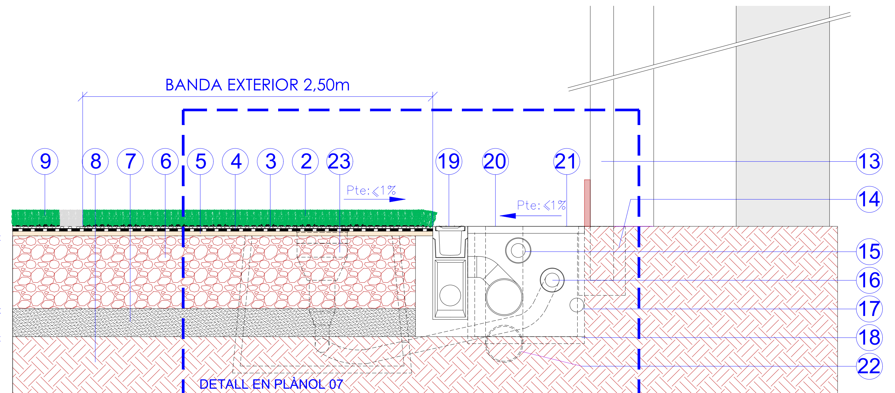
DETALL TROBADA PAVIMENT GESPA EN EXTREM LATERAL DEL CAMP
