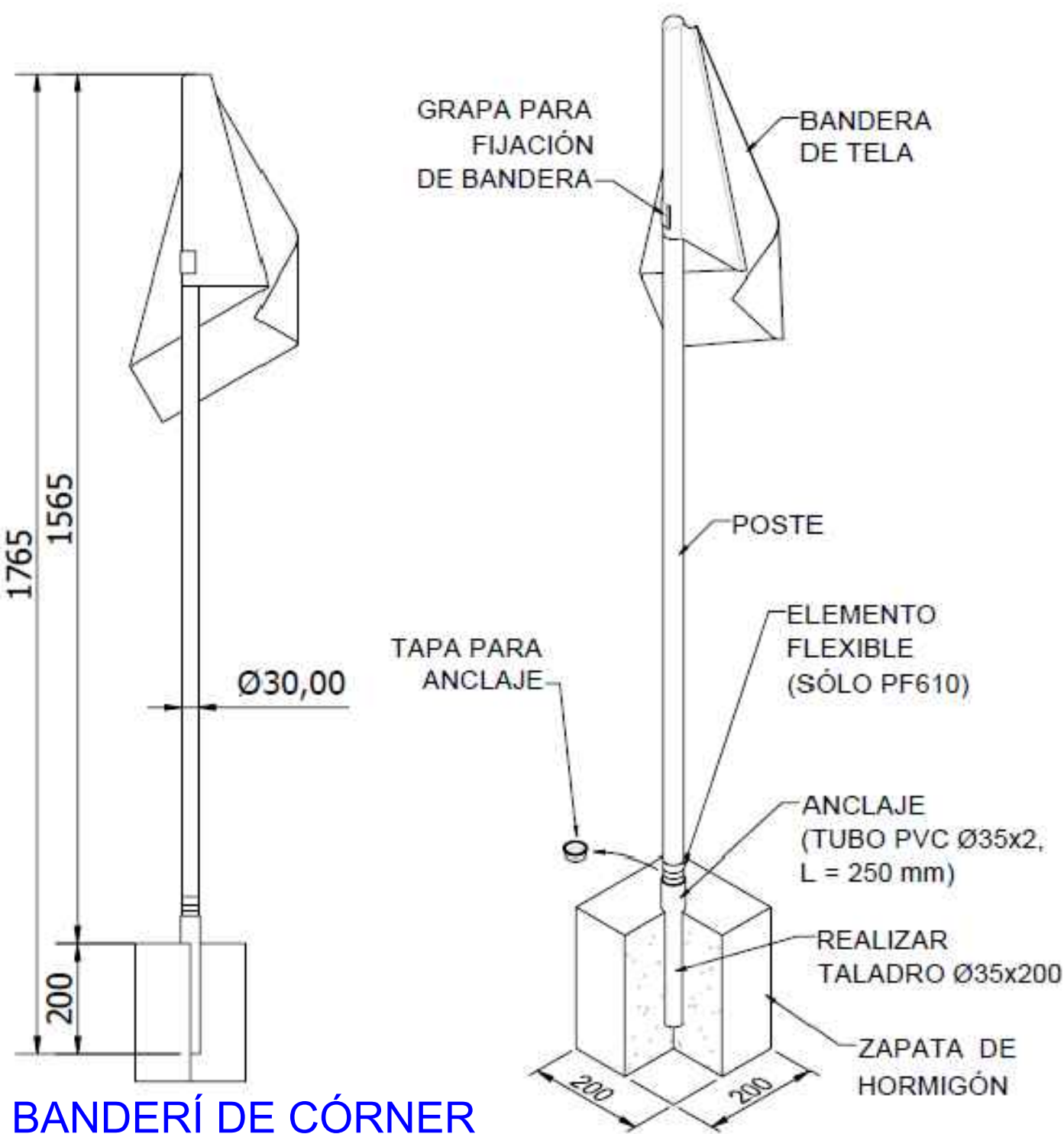
BANDERÍ DE CÓRNER
