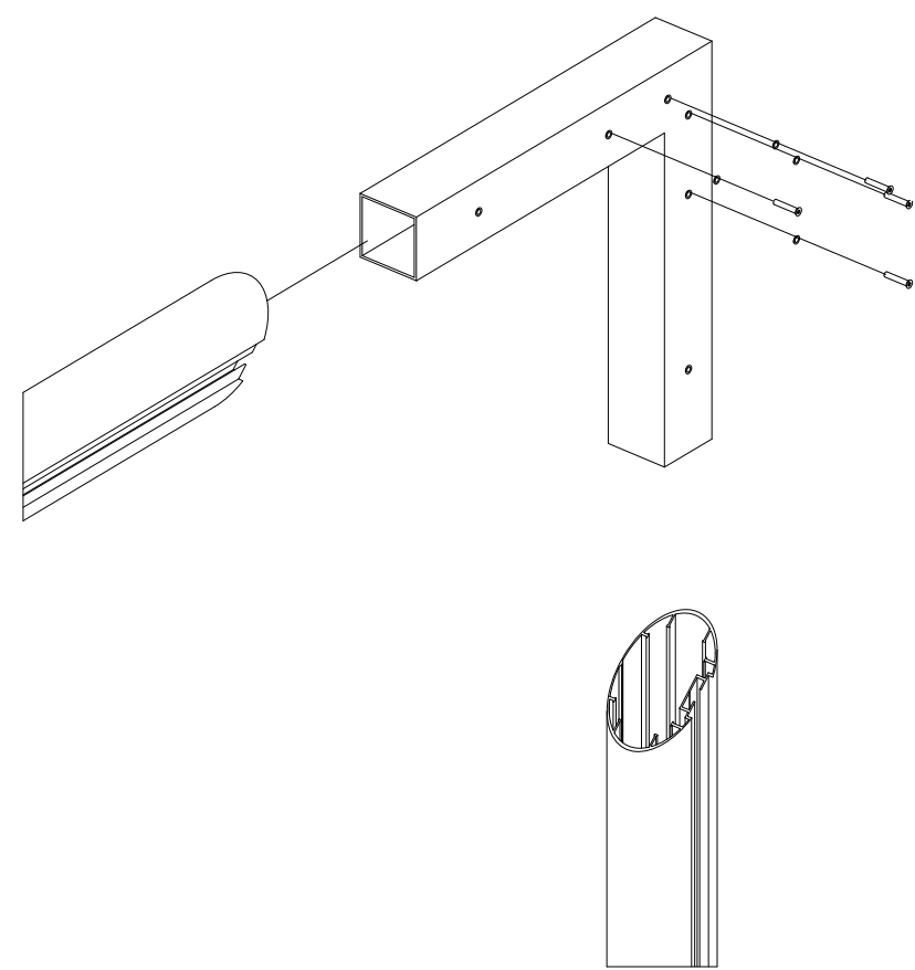
DETALL UNIÓ PAL I TRAVESSER I ARQUILLO XARXA
