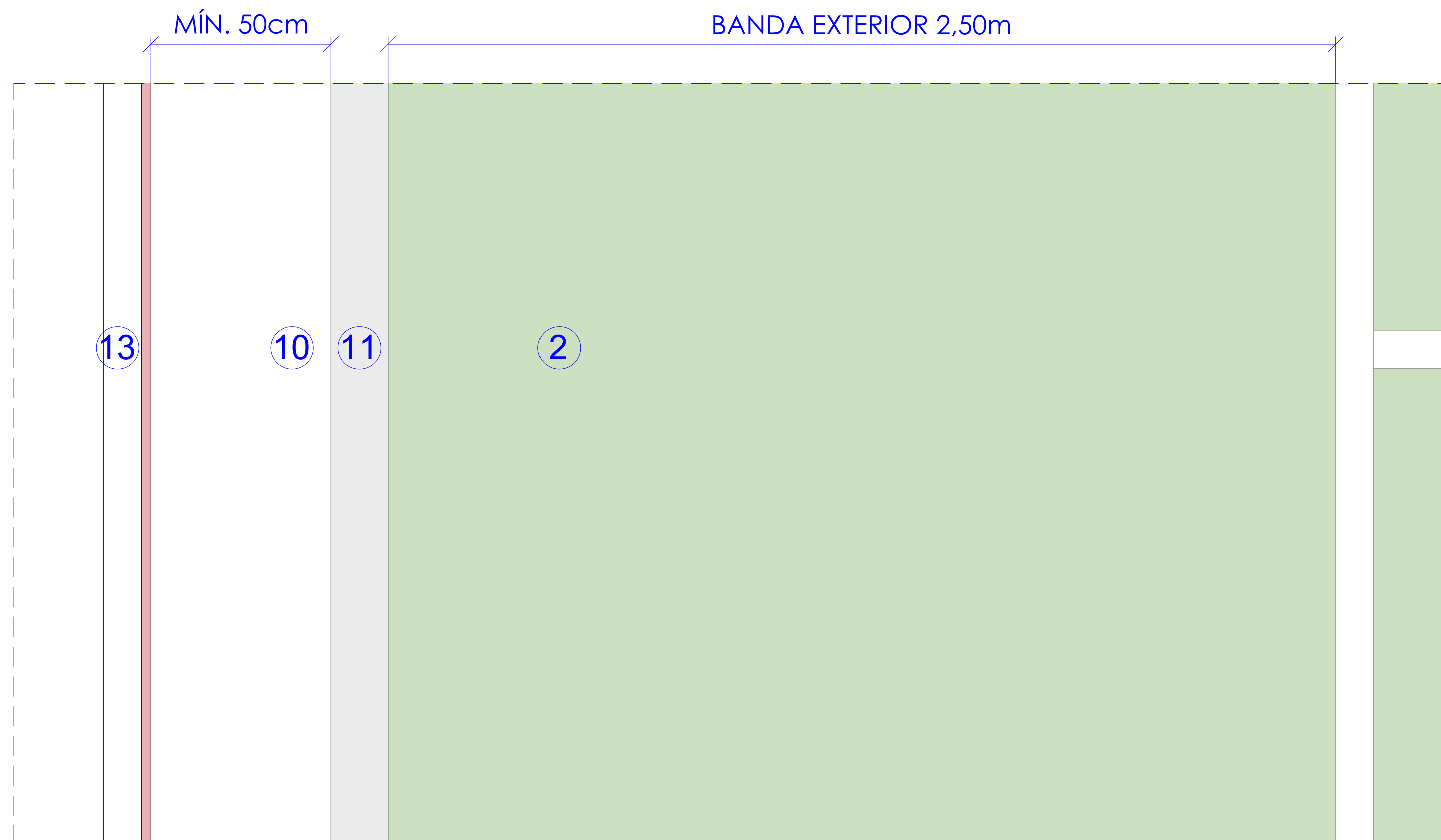
DETALL TROBADA PAVIMENT GESPA EN EXTREM FINAL DEL CAMP
